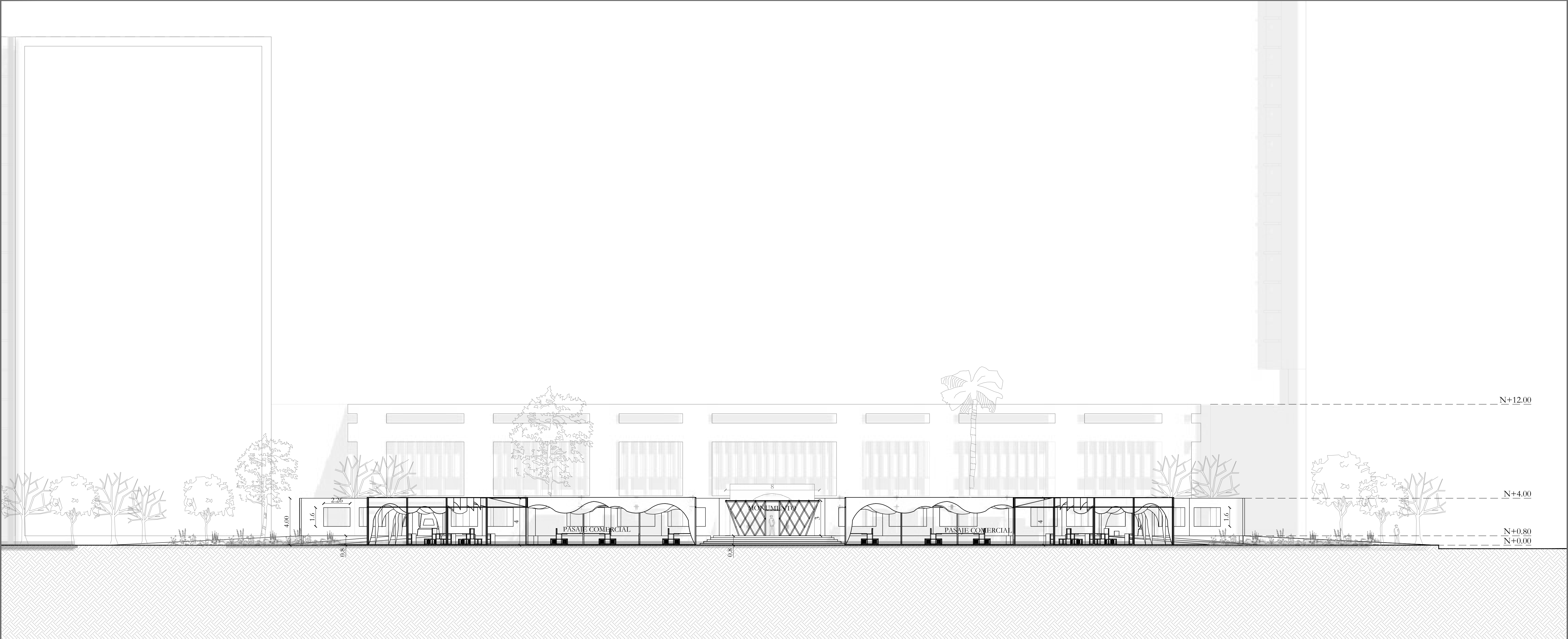
G-003 CORTE TRANSVERSAL 1-1' ESC: 1 : 150
