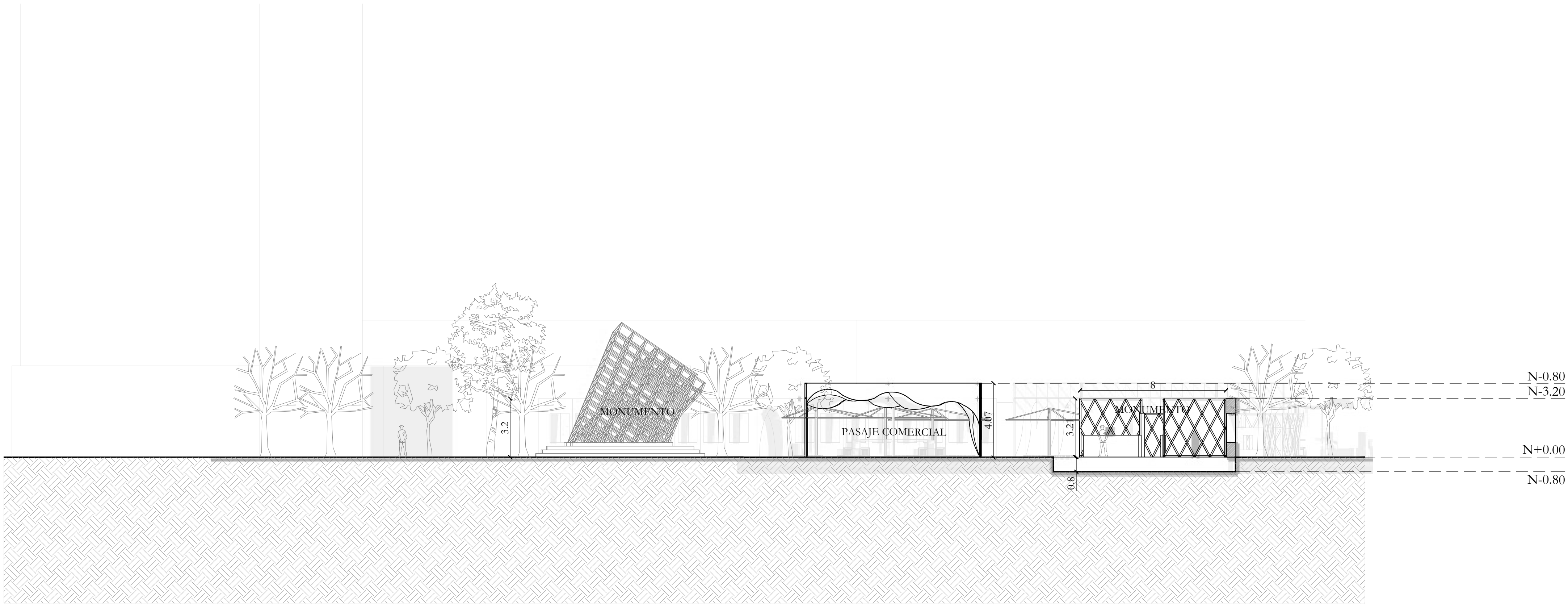
G-004 CORTE TRANSVERSAL 3-3' ESC: 1 : 150
