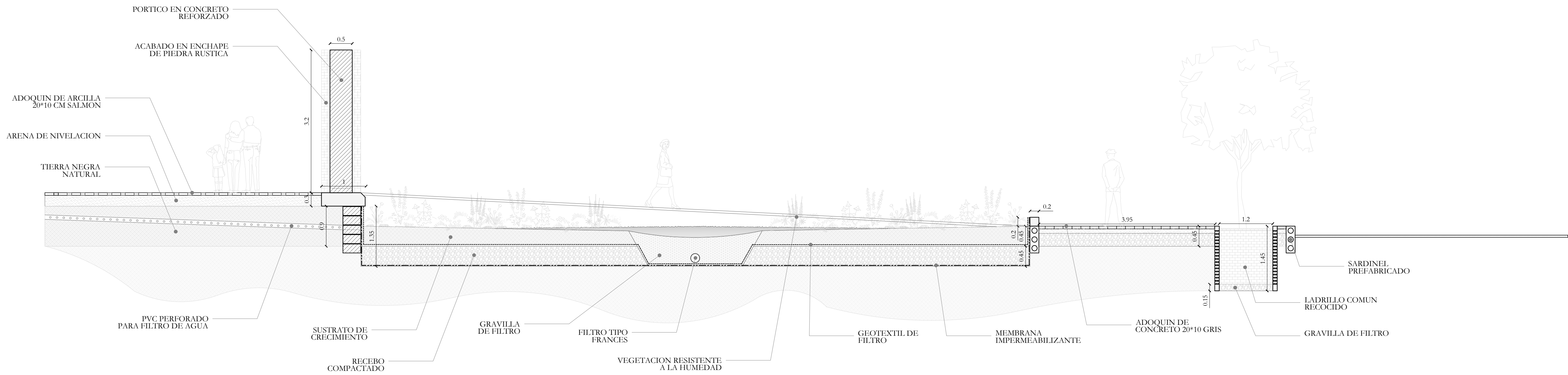
G-007 DETALLE JARDIN DE LLUVIA ESC: 1 : 50
