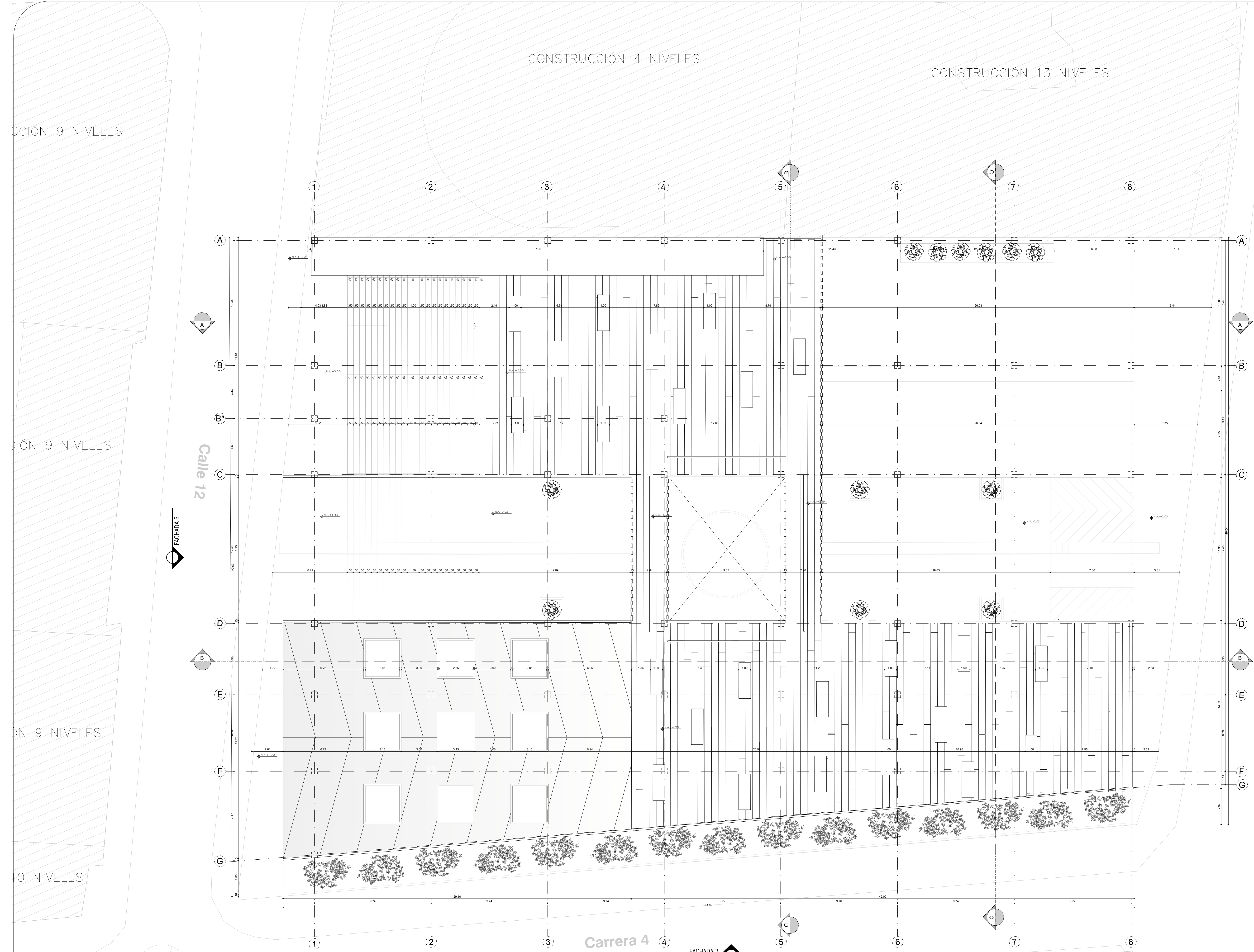
PLANTA PISO 3 ESC: 1 ____ 150
