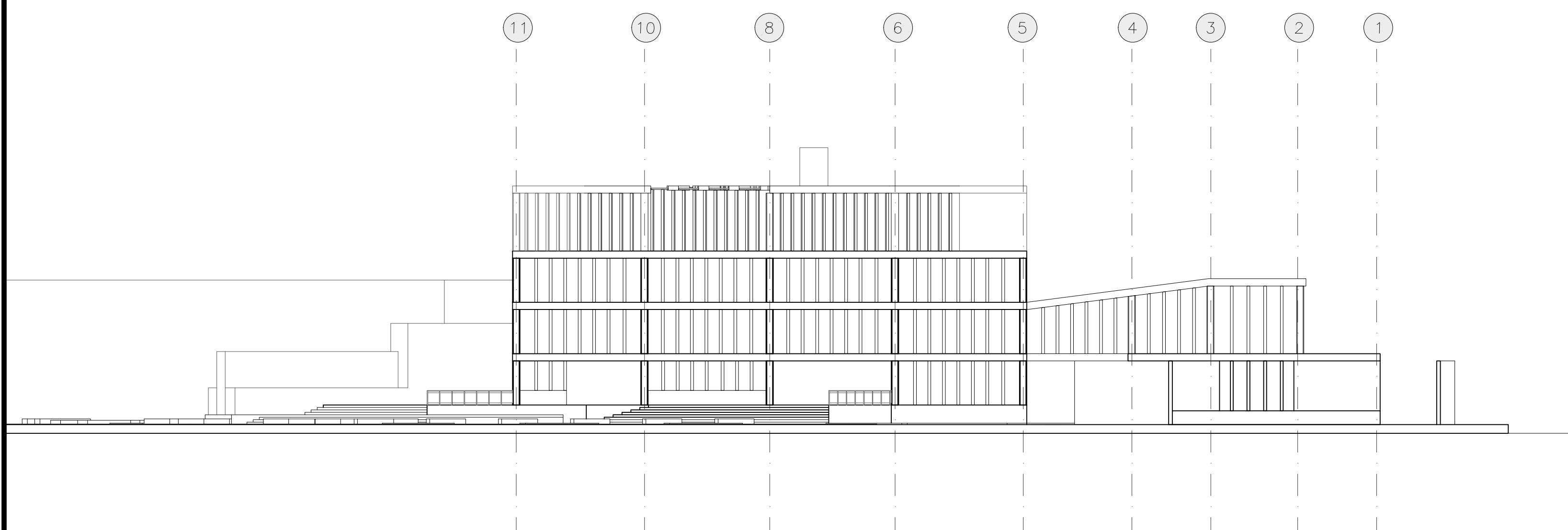
F1 FACHADA NORTE
