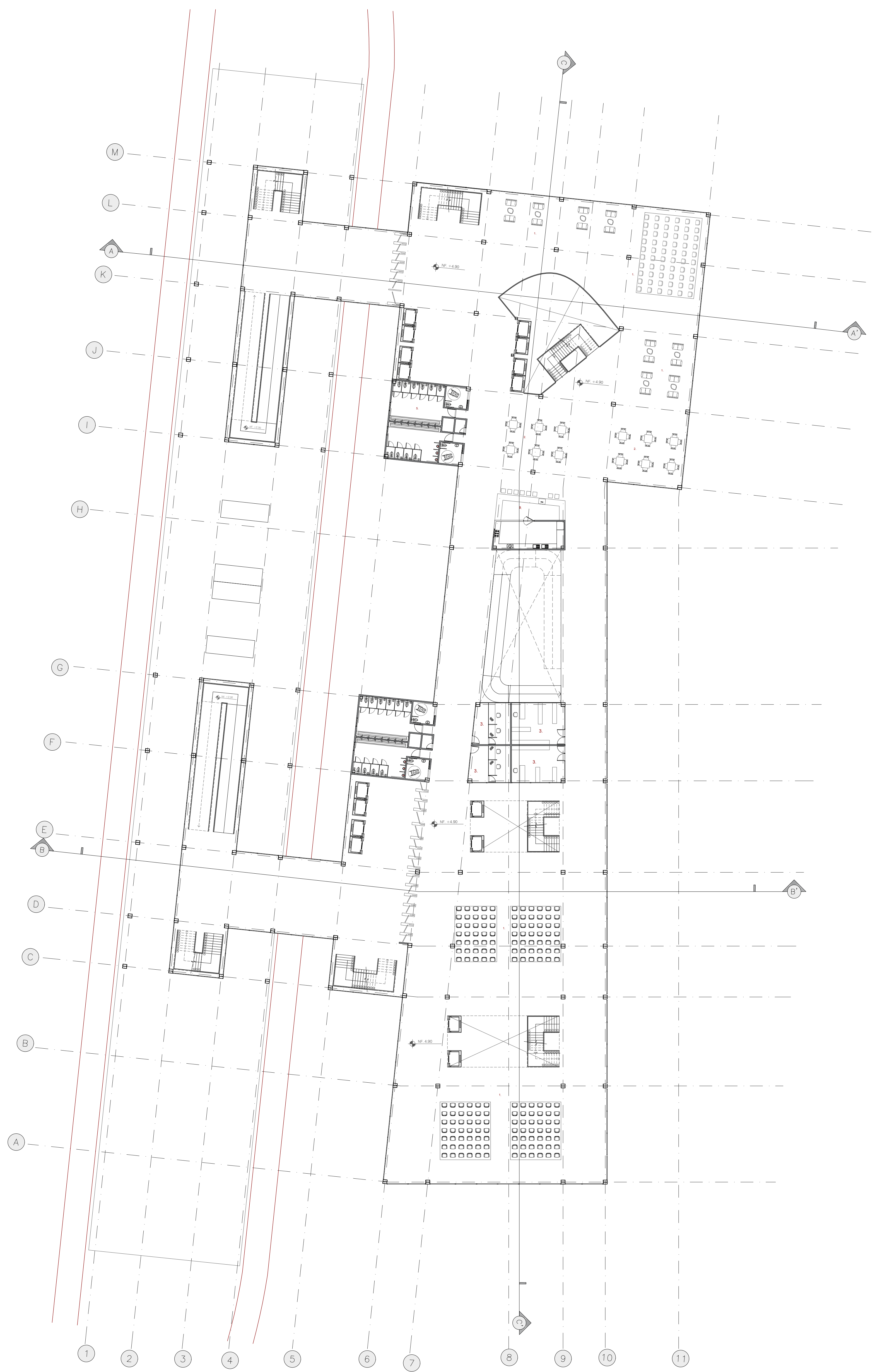
P2 SEGUNDA PLANTA ESCALA 1:250
