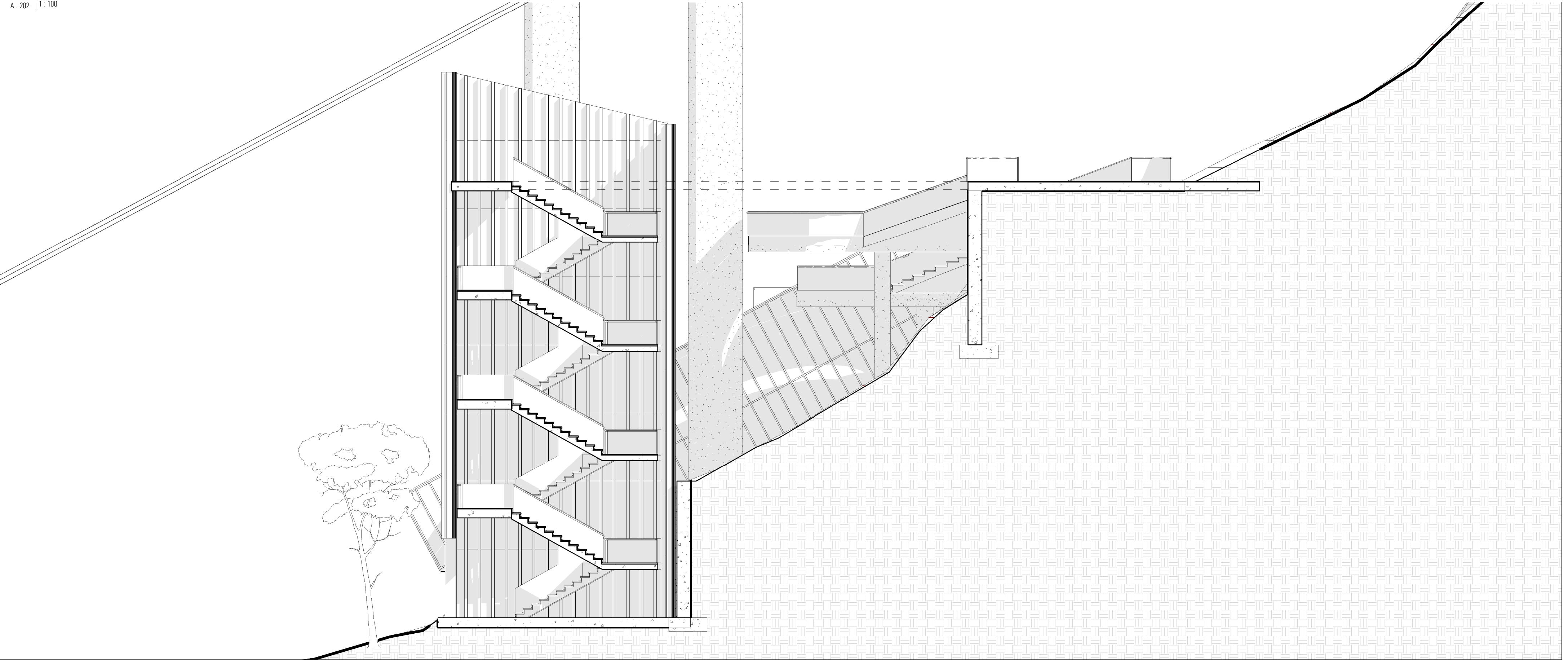
1 | Corte Longitudinal - 1 A. 202 | 1:100
