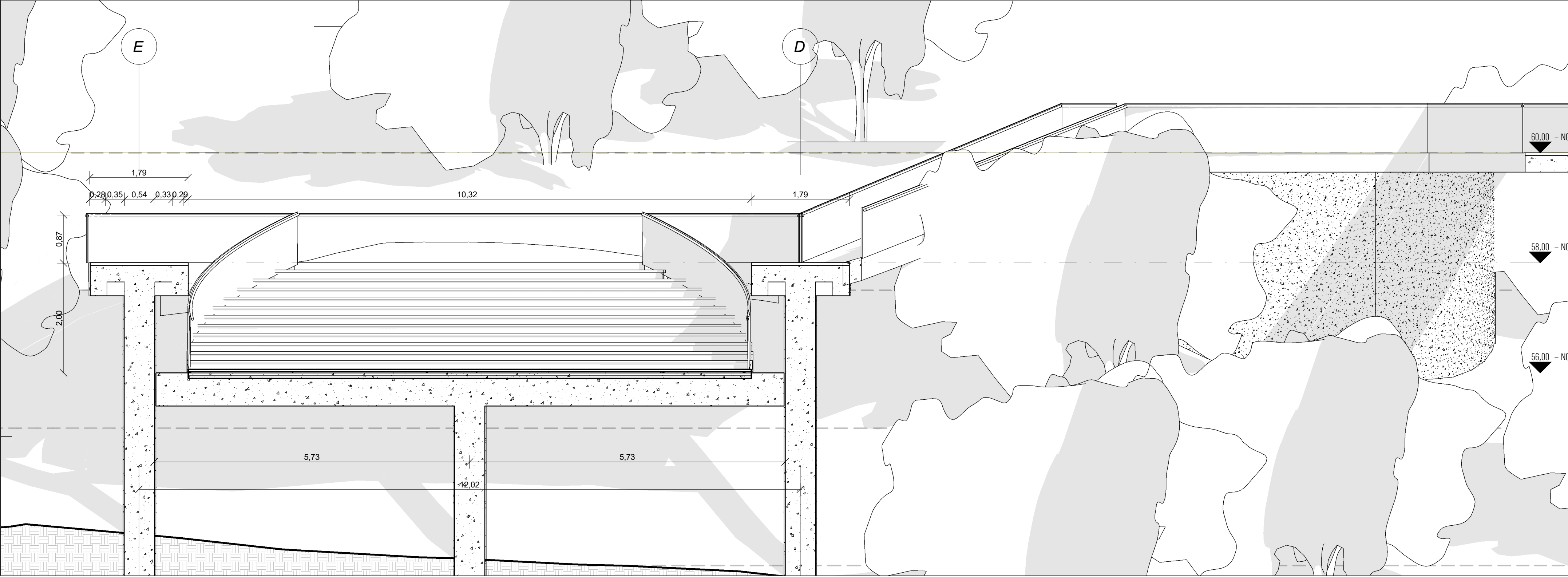
2 | Corte Trasversal Auditorio A . 214 | 1 : 50
