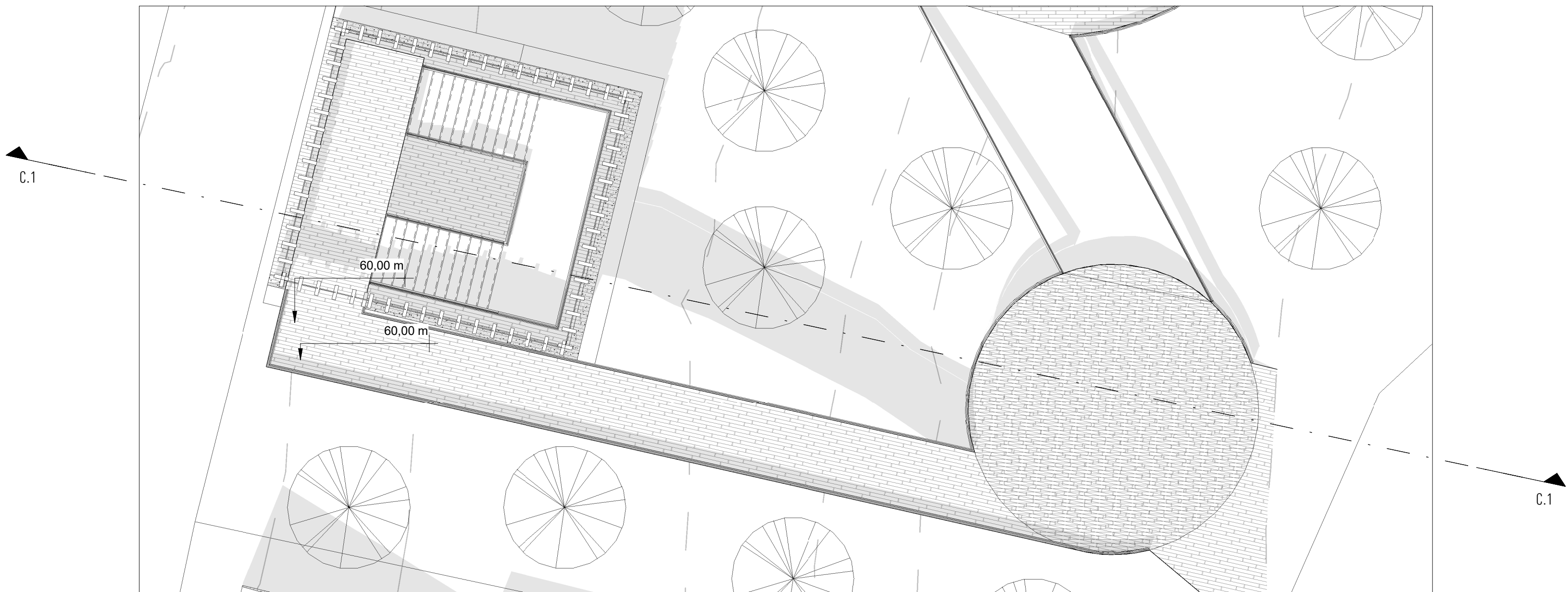
3 | Planta Escalera A. 203 | 1:100
