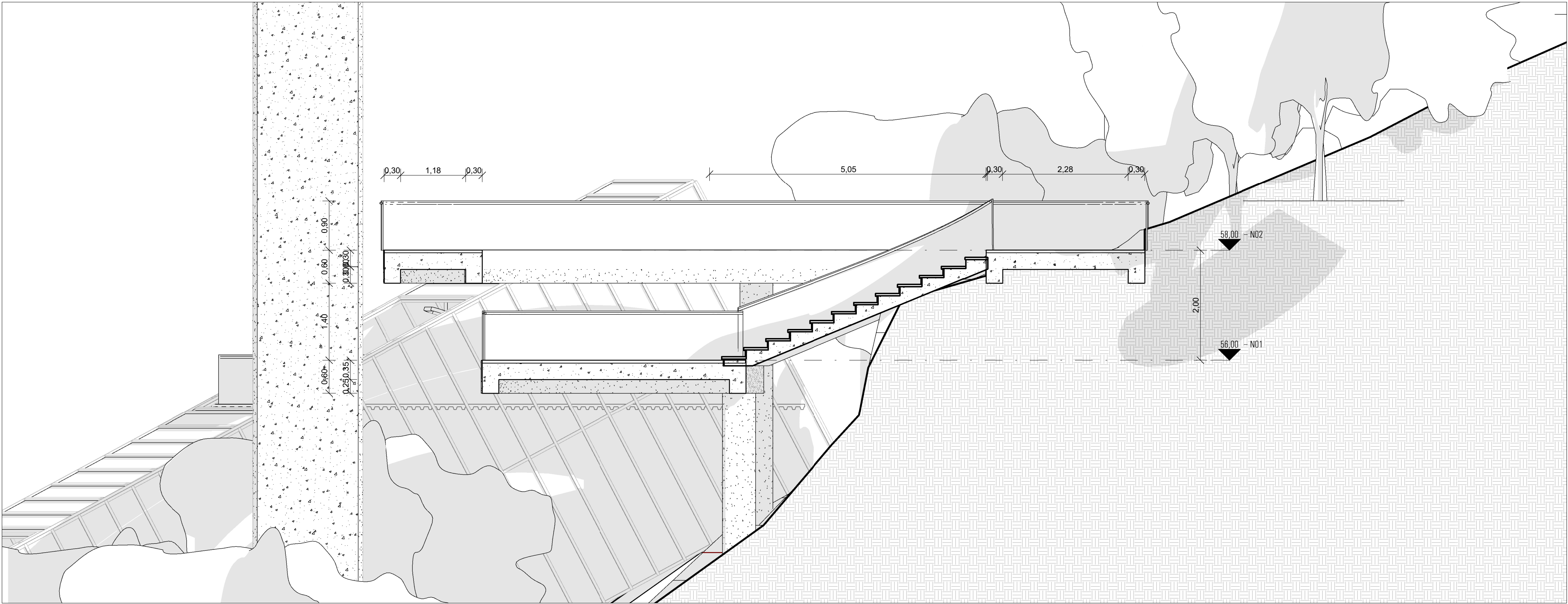
1 | Corte Longitudinal Auditorio A . 214 | 1 : 50
