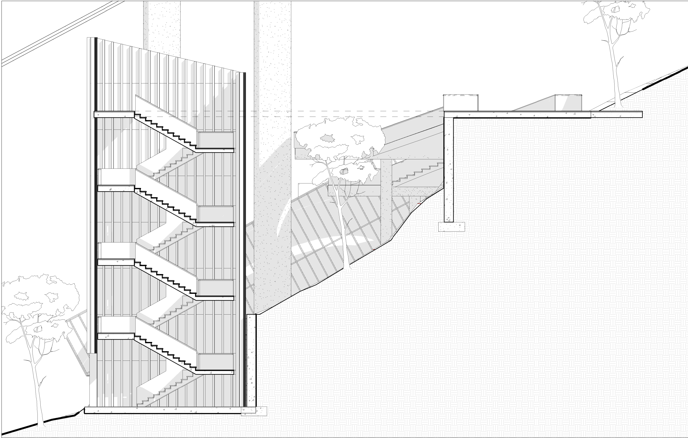
1 | Corte Escalera A. 203 | 1:100
