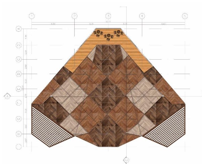
Imagen 8. Planta cubierta
