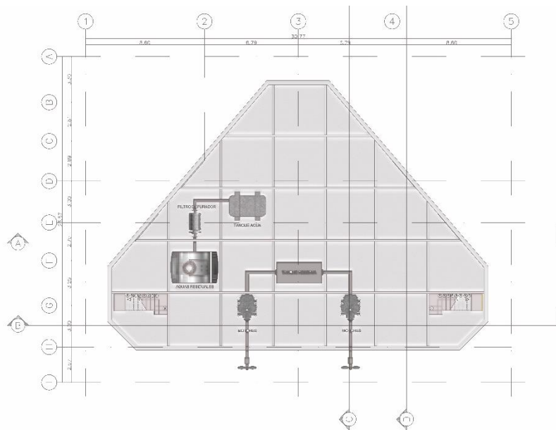
Imagen 5. Planta cuarto de bombas. “planchón”
