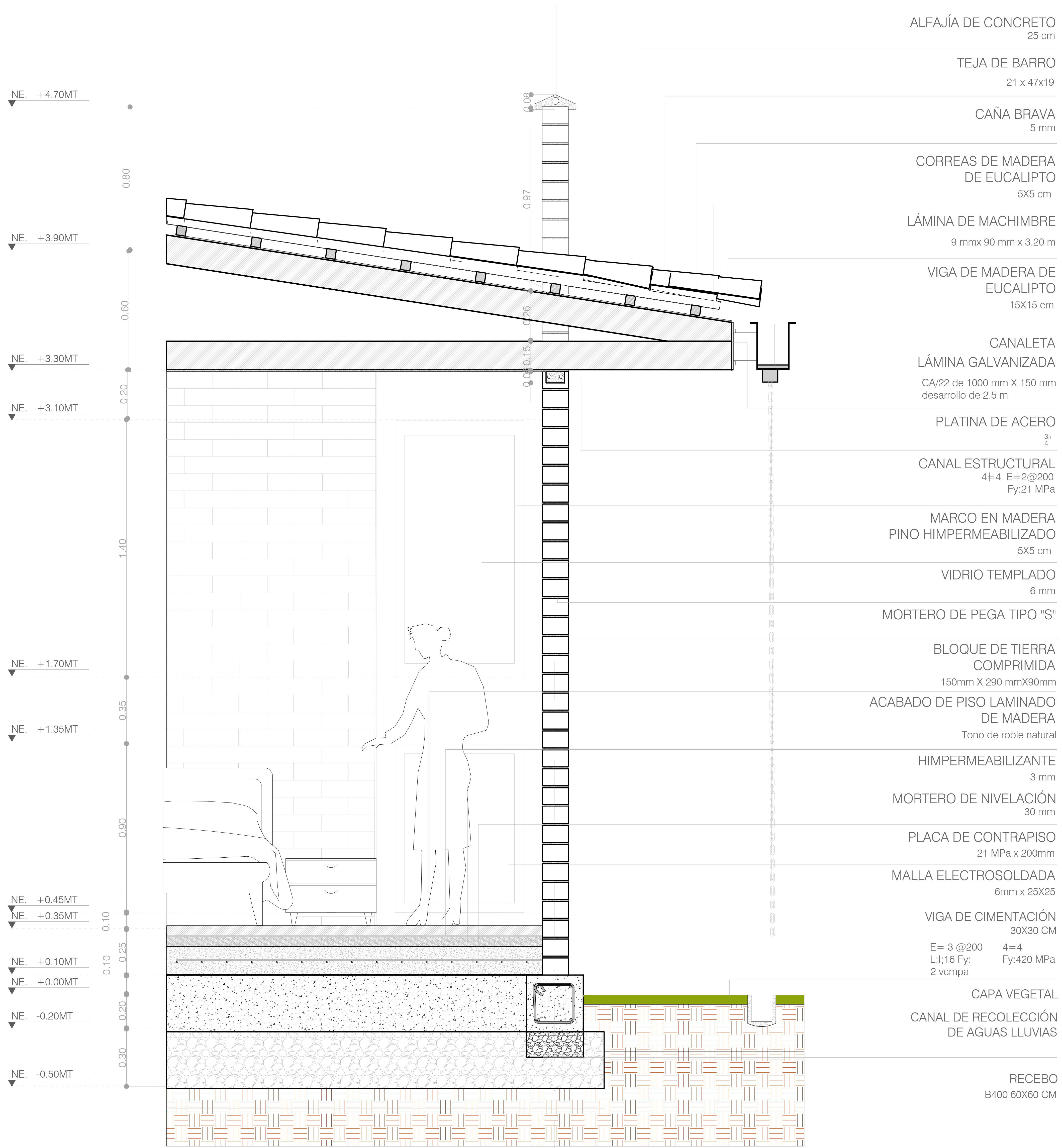
CF CORTE FACHADA 01 ESCALA 1:10
