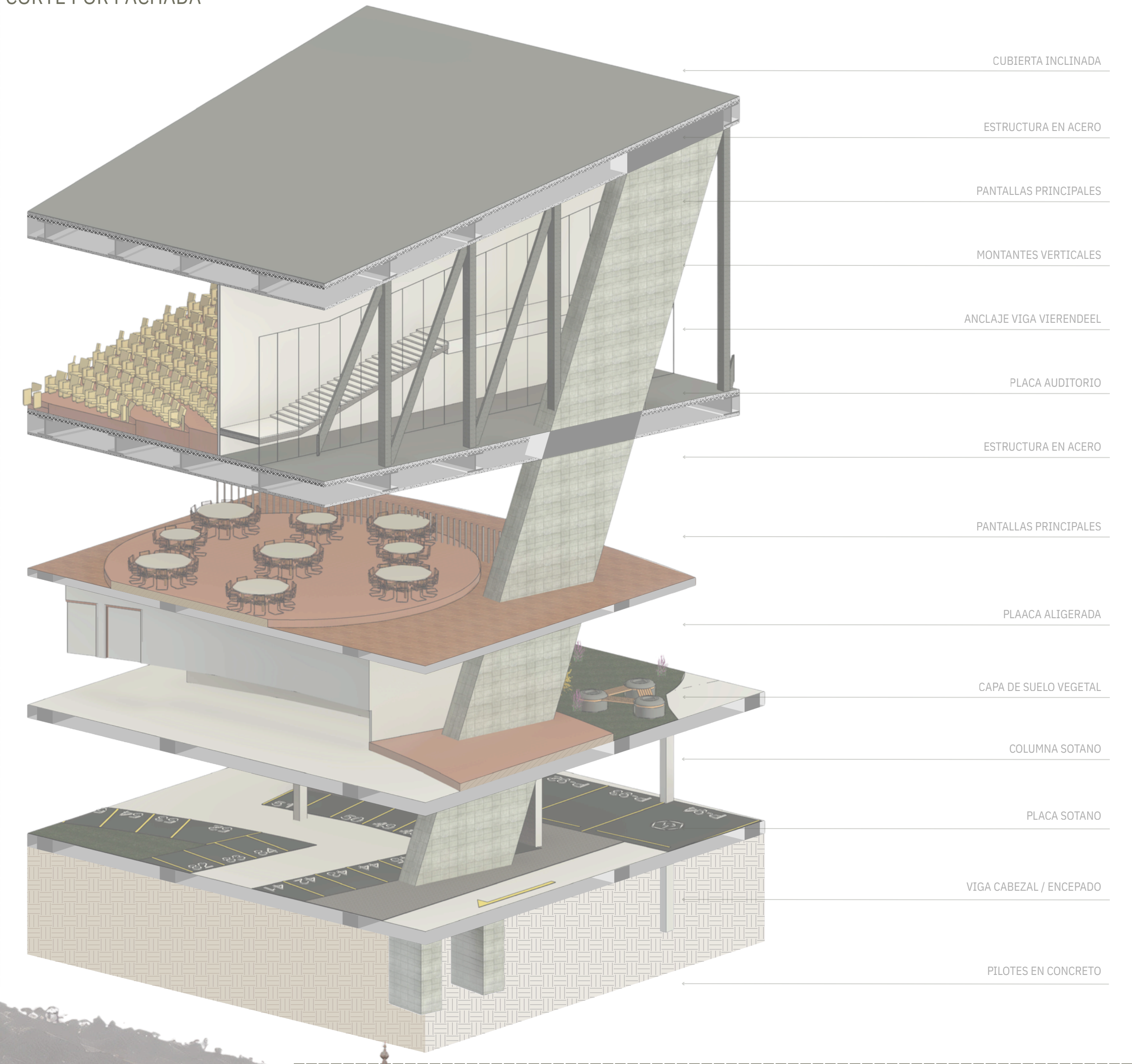
CORTE POR FACHADA
