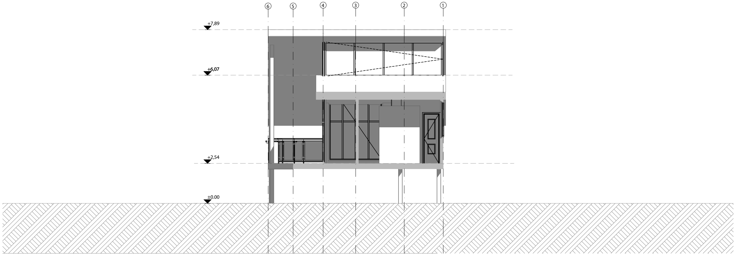
1. CORTE LONGITUDINAL 1:100
