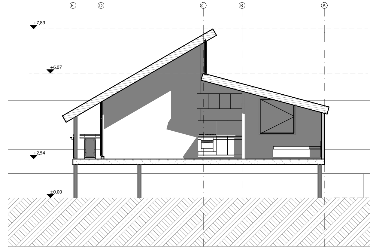
2- CORTE TRANSVERSAL 1:100
