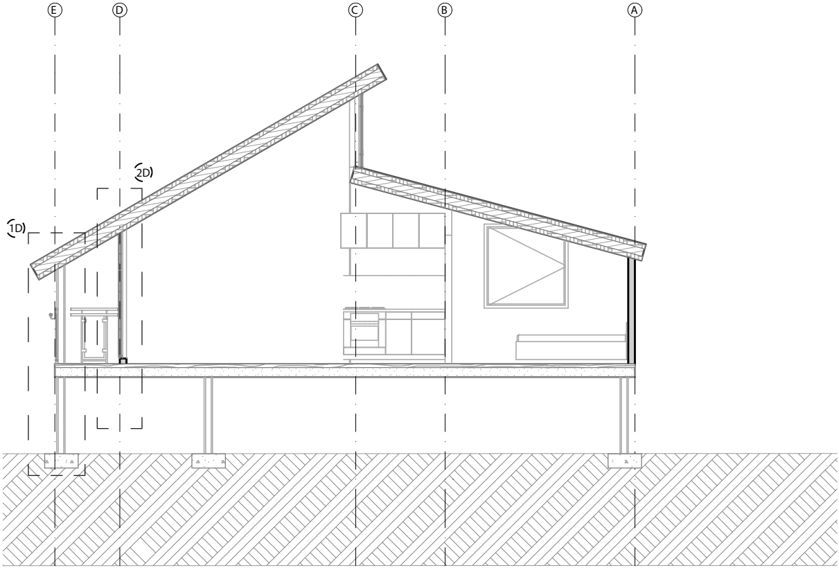
1. DETALLE LONGITUDINAL 1:100
