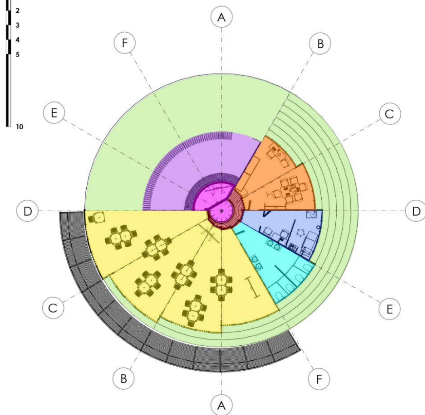
01 Estructura Cerrada Esc. 1:150
