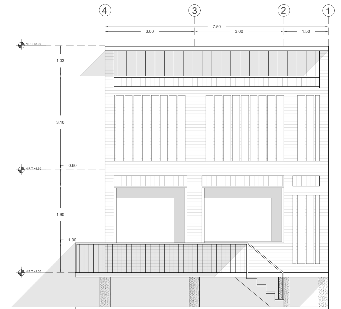
Fachada B-B
