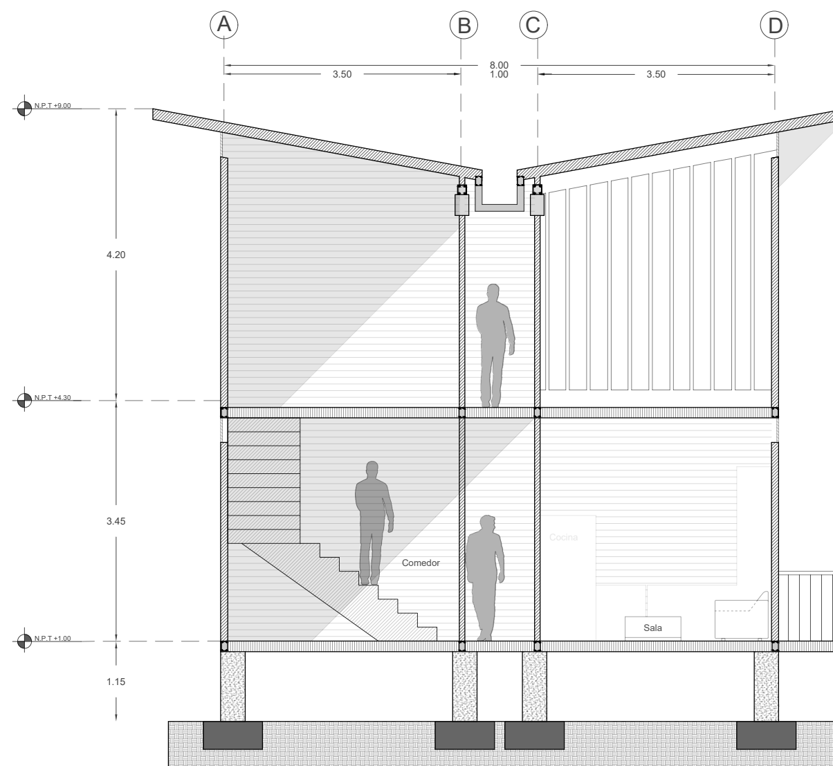
Corte A-A
