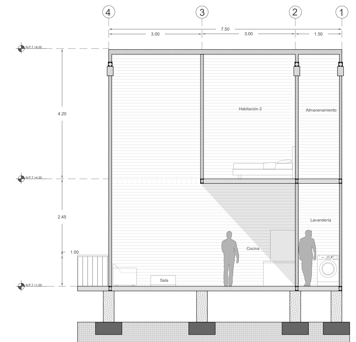
Corte B-B
