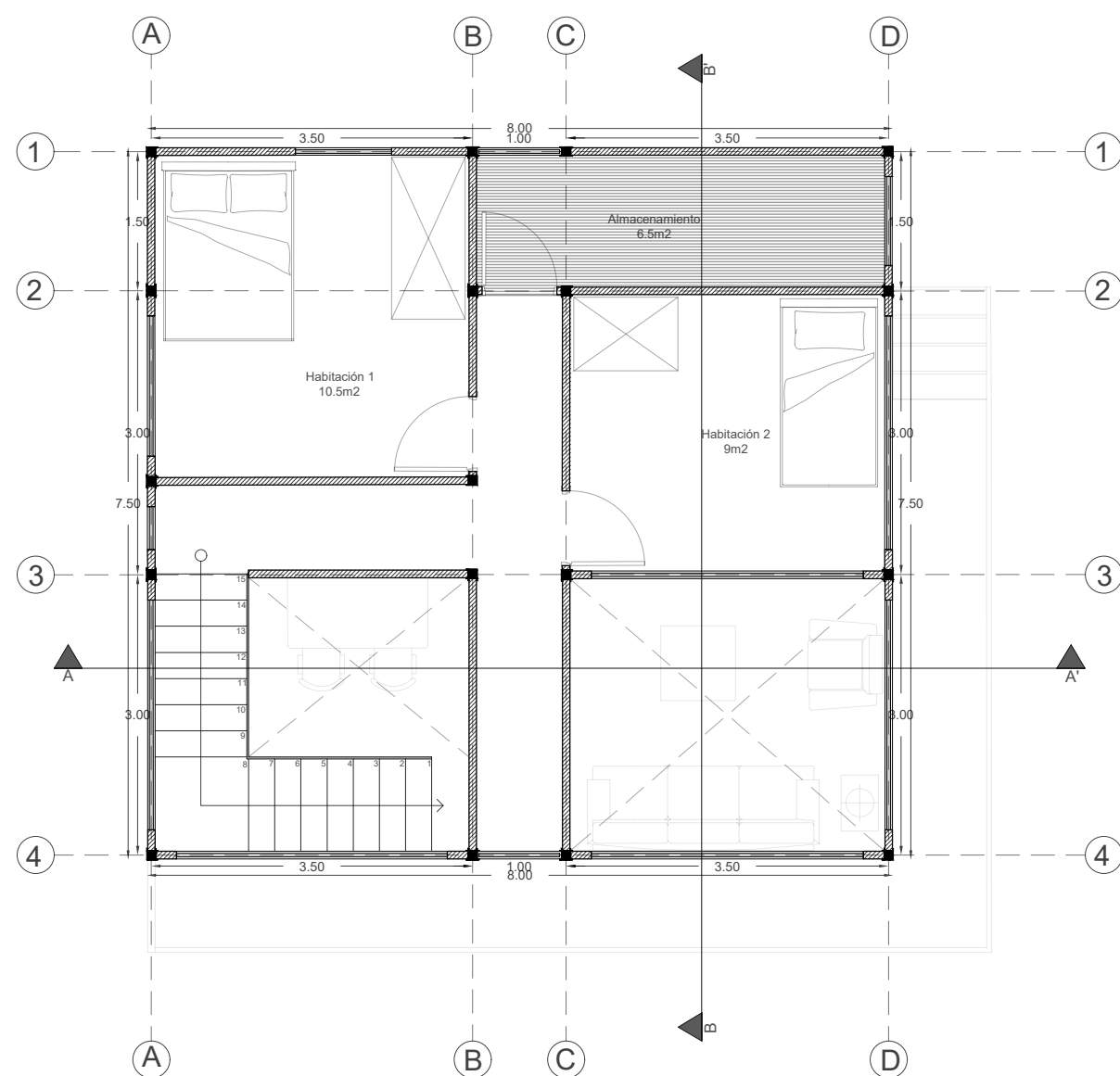
Segunda Planta 60m 2
