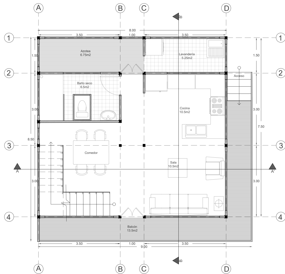
Primera Planta 75m 2
