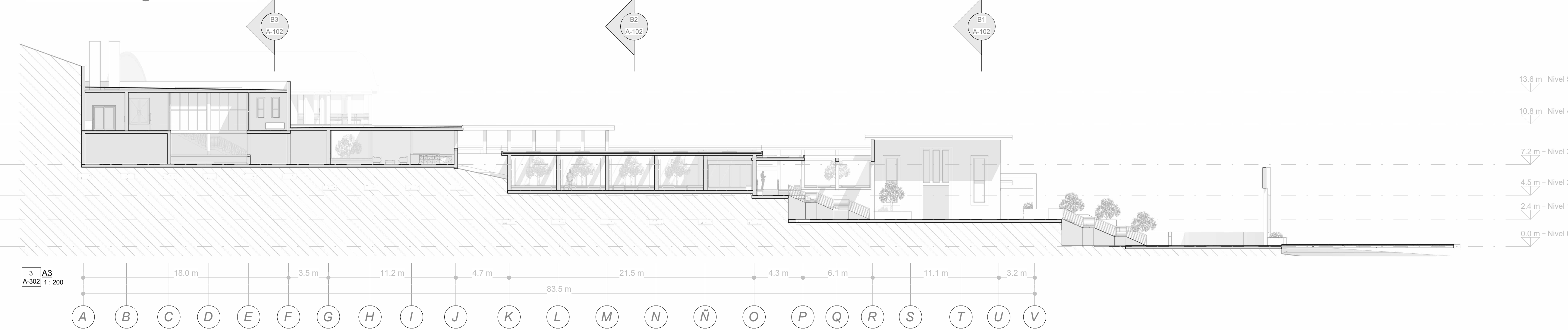
Sección longitudinal A3
