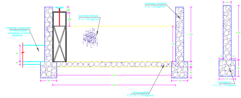
CORTE A-A'
