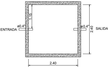
VISTA EN PLANTA
