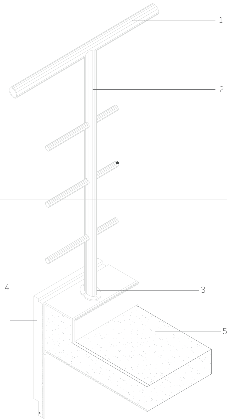
D1 DETALLE BARANDA
