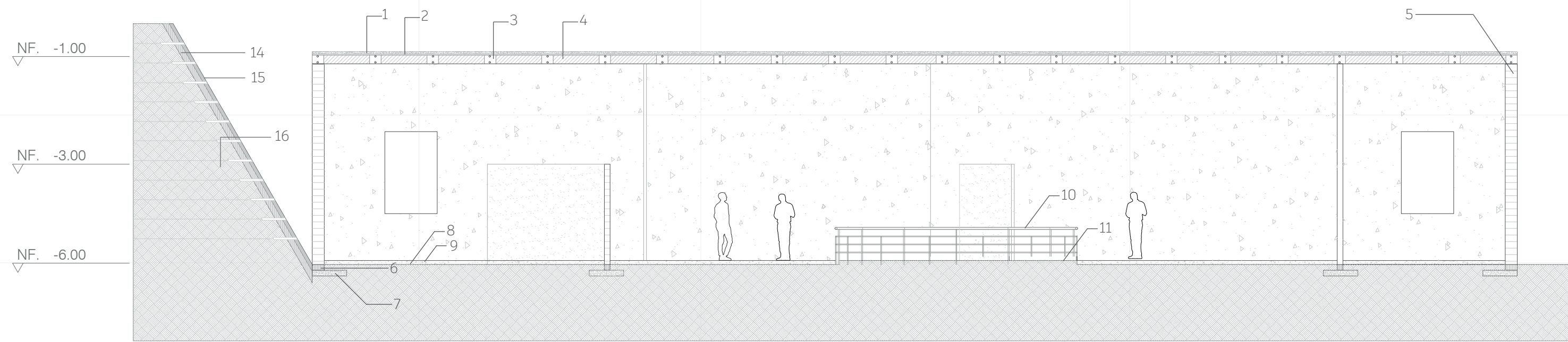
C5 CORTE PABELLÓN IRA Y LUCHA
