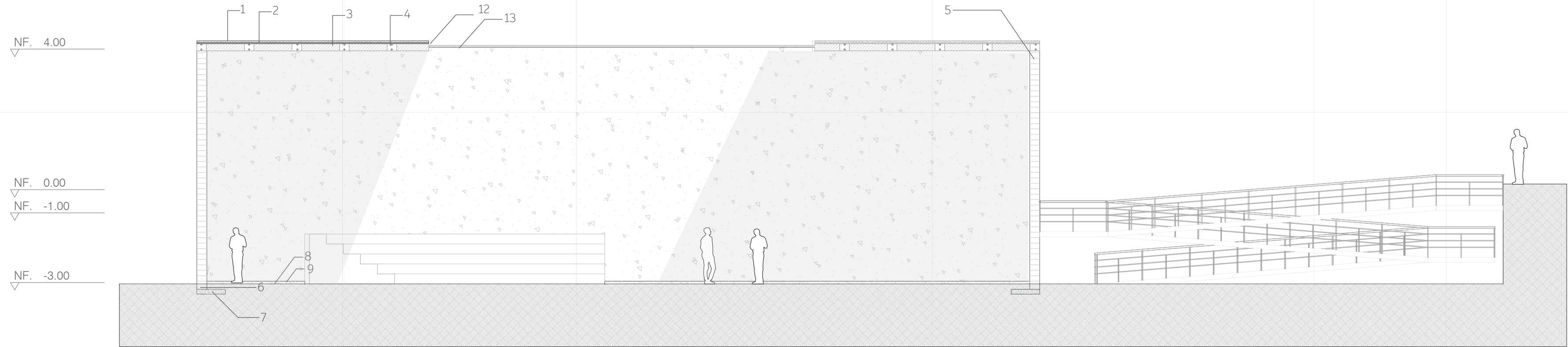
C9 CORTE PABELLÓN CONMEMORACIÓN
