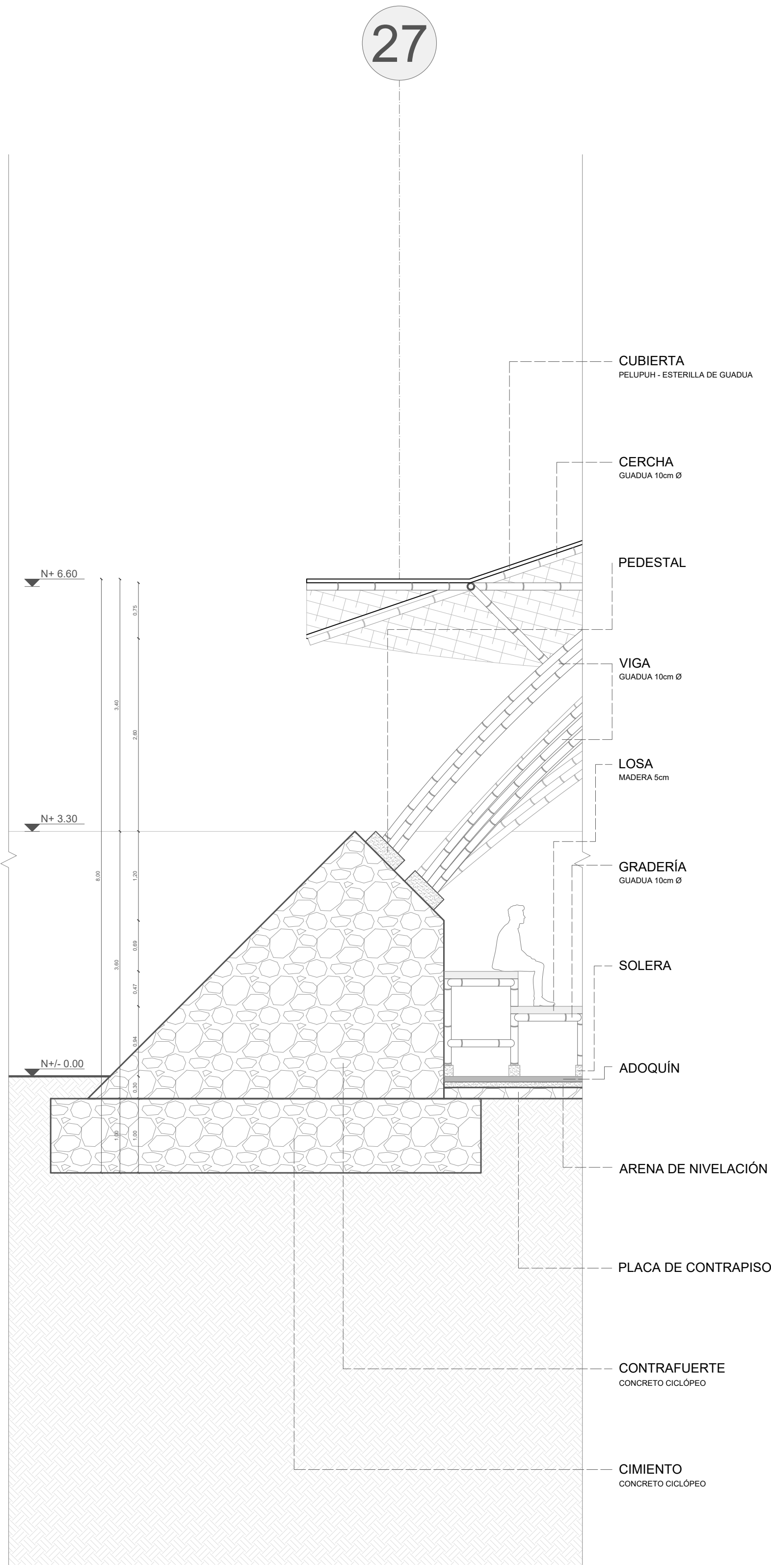
CORTE POR FACHADA 03
