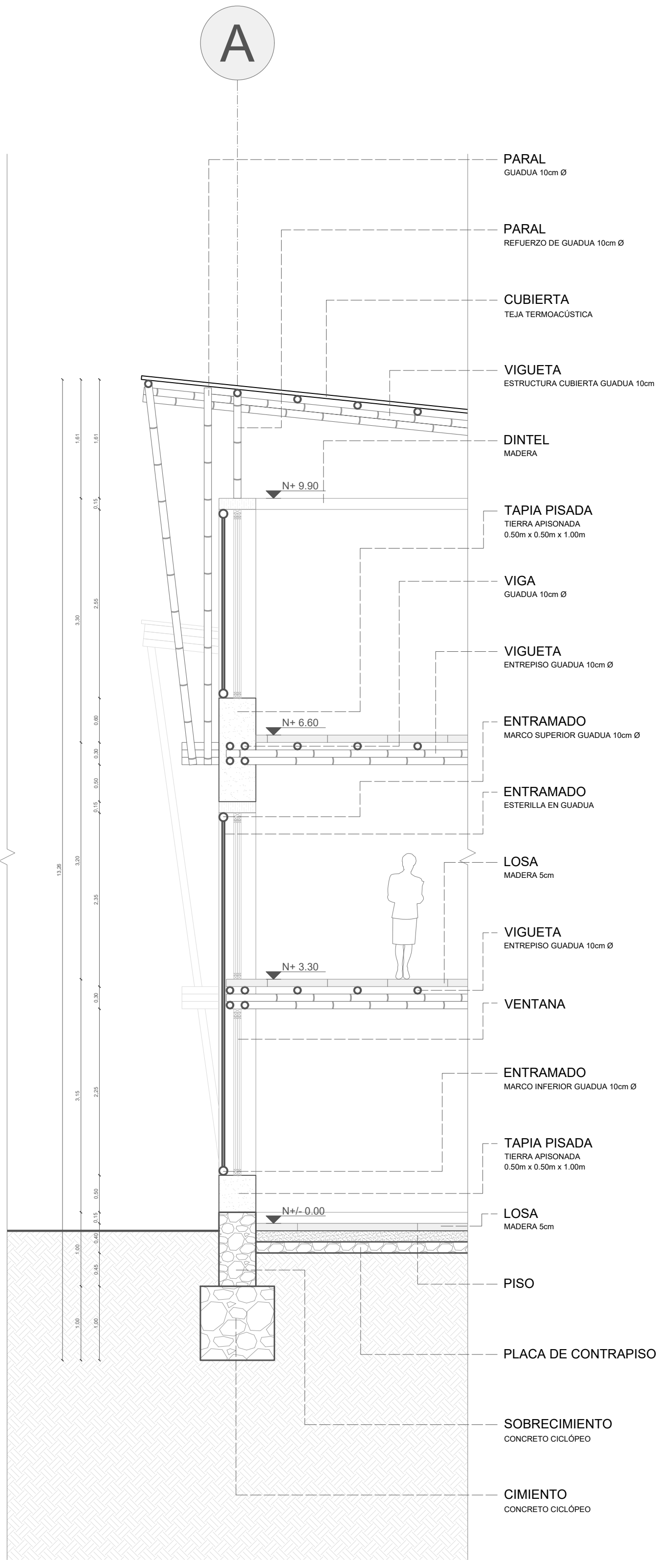
CORTE POR FACHADA 02
