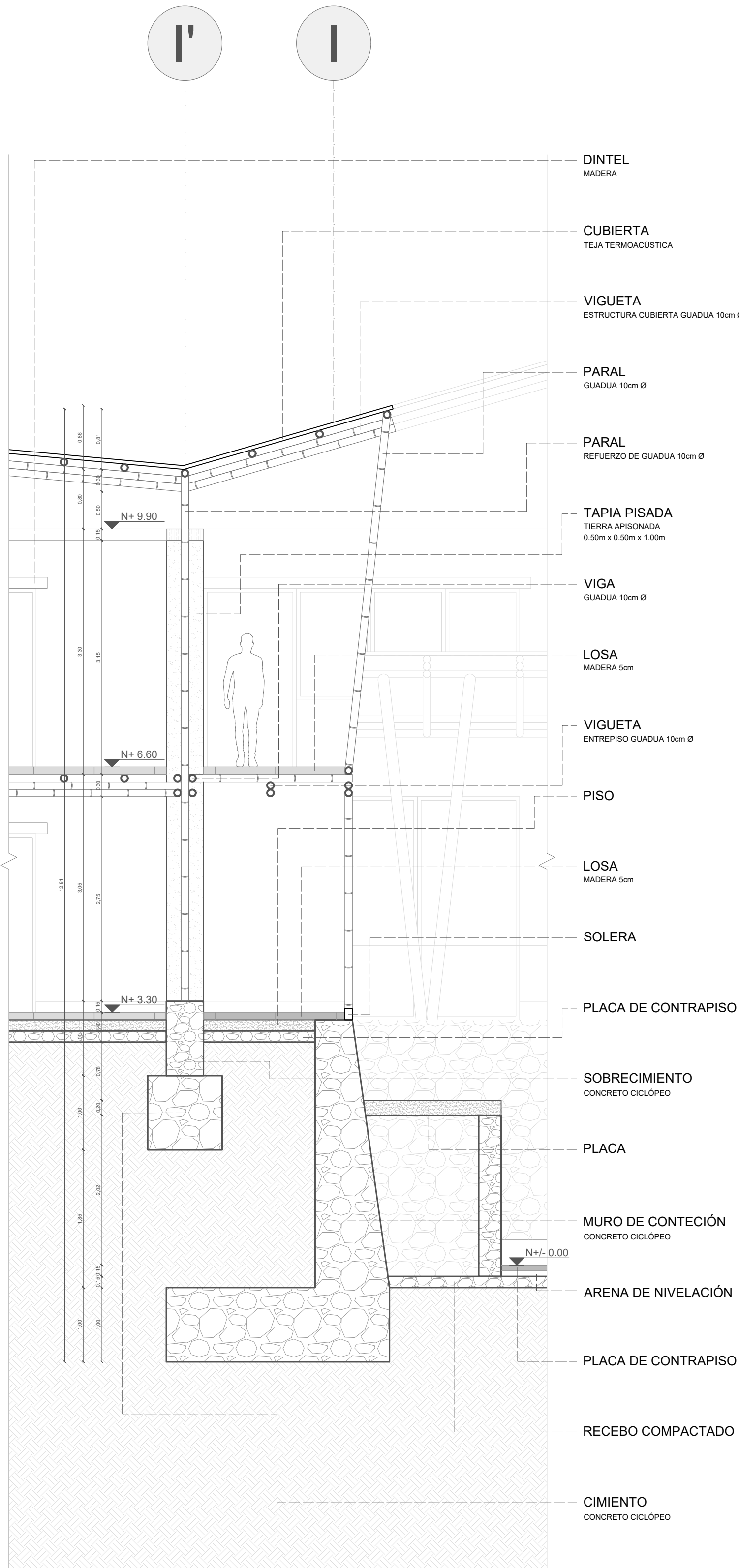
CORTE POR FACHADA 01
