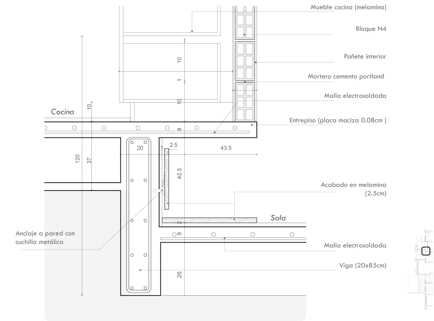
Detalle Nicho de sala D-2 Esc 1:10
