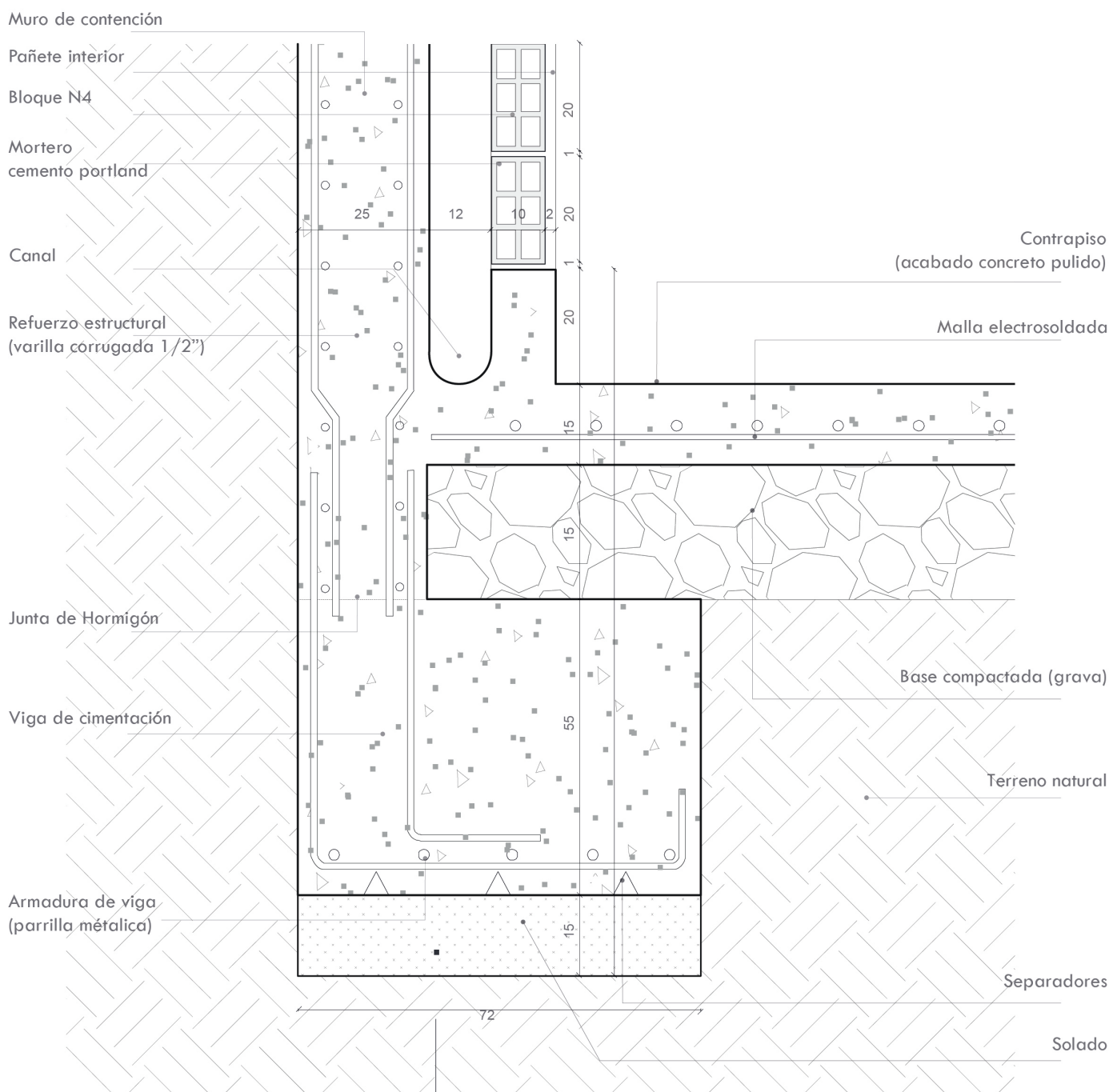
Detalle cimentación D-4 Esc 1:10
