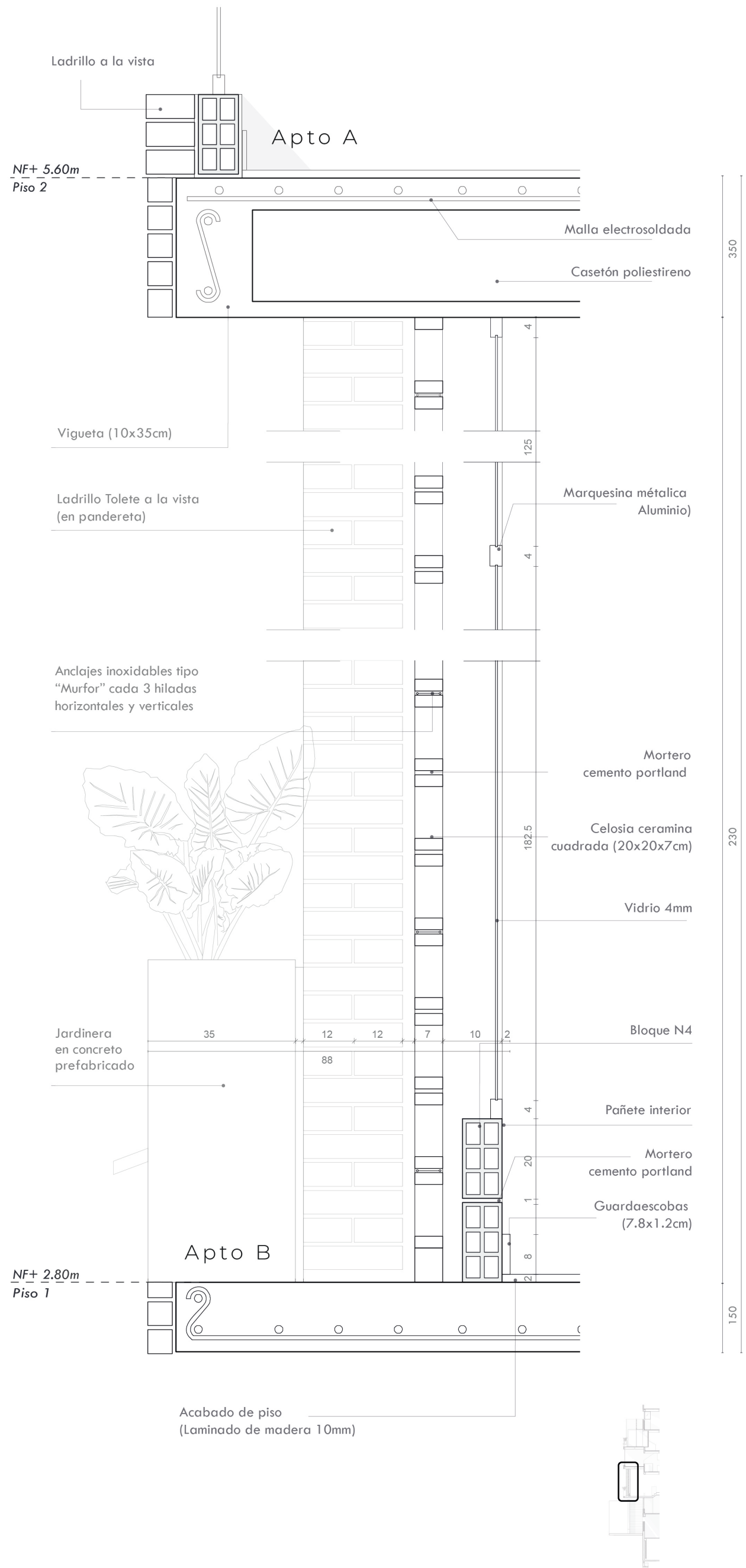
Detalle corte por fachada D-1 Esc 1:10
