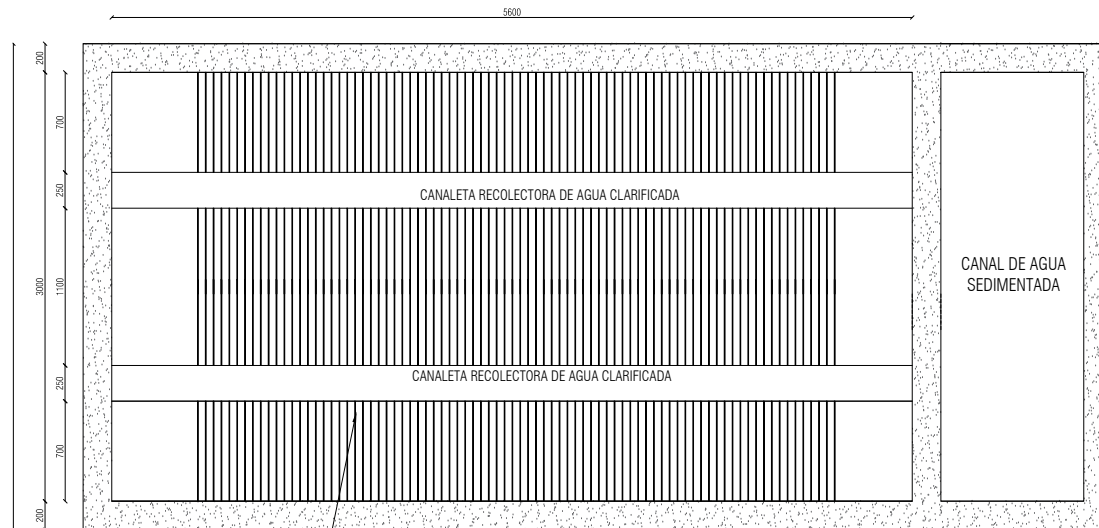
VISTA EN PLANTA ESC. 1:20
