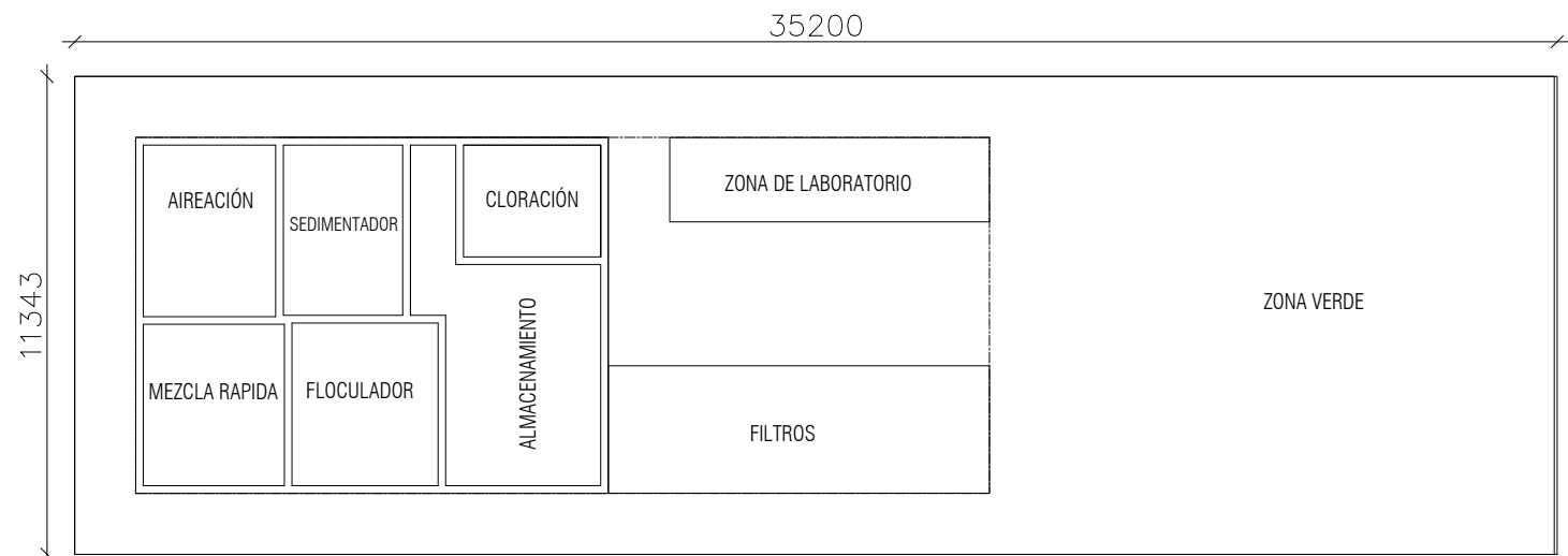
VISTA EN PLANTA ACTUAL PTAP SOSIEGO ESC. 1:10
