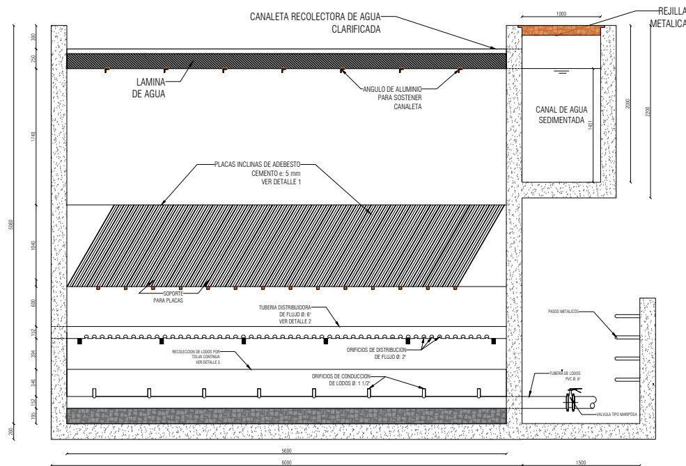
VISTA LATERAL ESC. 1:20
