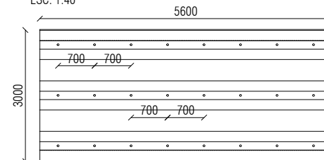
DETALLE 1 DIMENSIONAMIENTO PLACAS ESC. 1:40
