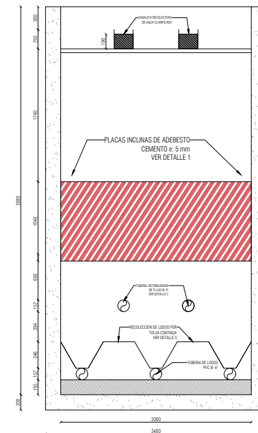
VISTA FRONTAL ESC. 1:20
