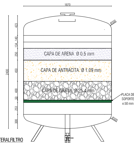
VISTA LATERAL FILTRO ESC. 1:40
