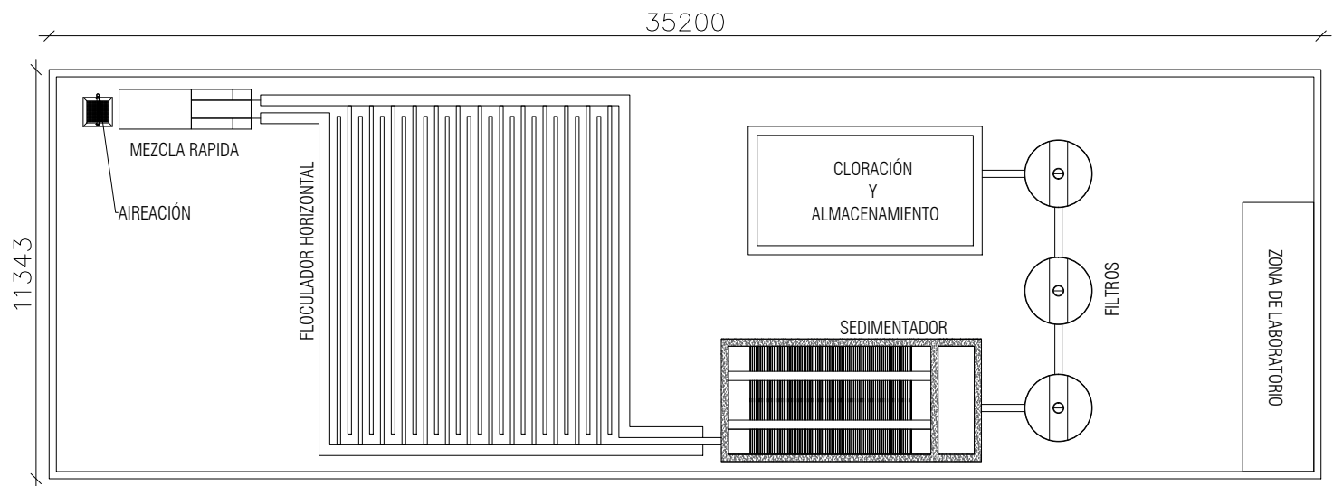
VISTA EN PLANTA REDISEÑO PTAP SOSIEGO ESC. 1:10
