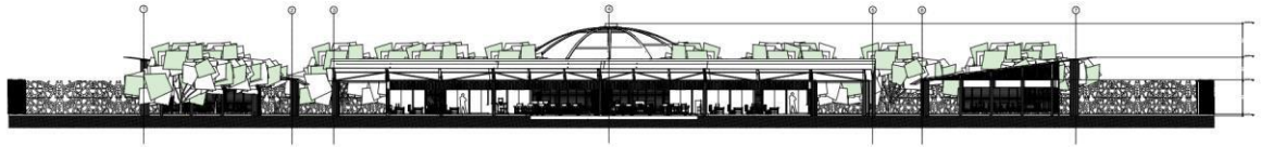
CORTE LONGITUDINAL D-D
