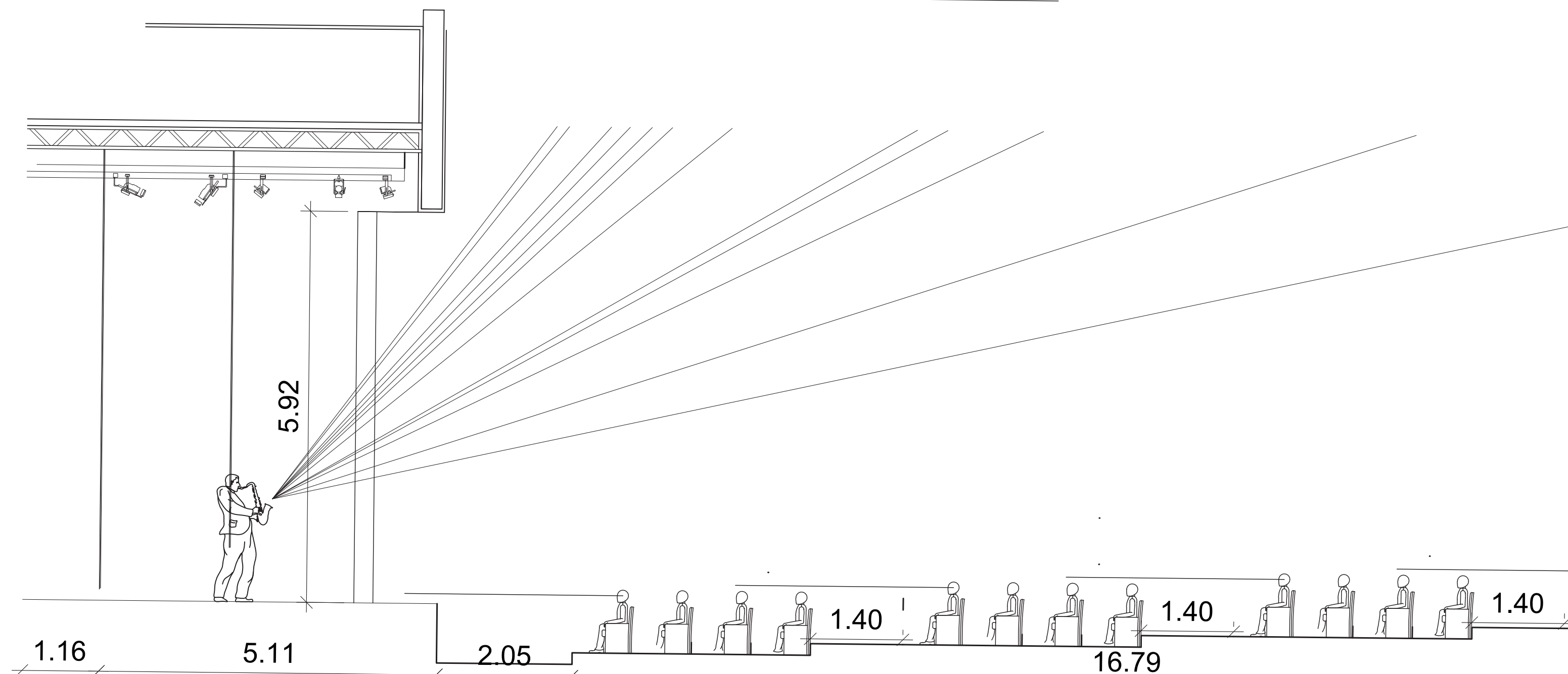
DETALLE TEARINO ESCALA 1:50
