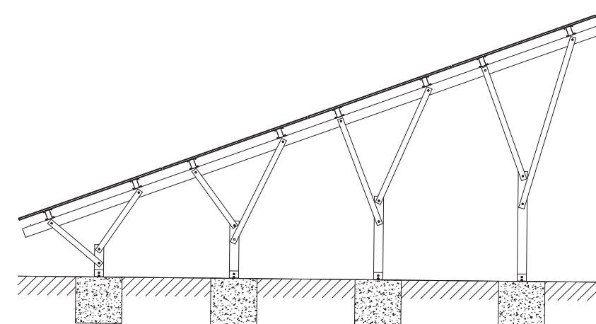
DETALLE PANEL SOLAR ESCALA 1:50
