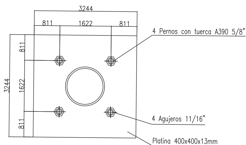
DETALLE ANCLAJES-PANEL ESCALA 1:10
