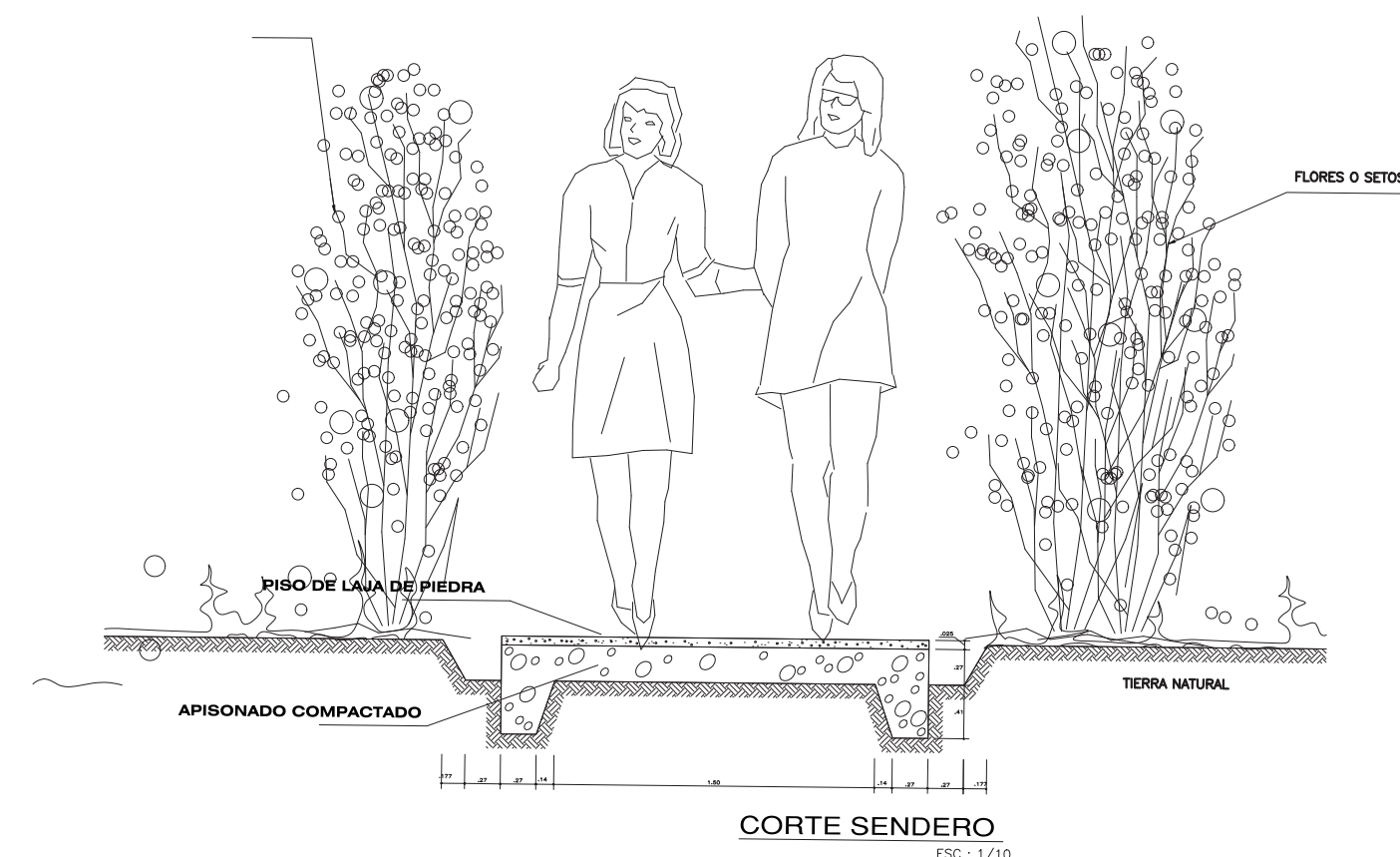
DETALLE SENDERO PEATONAL ESCALA 1:50
