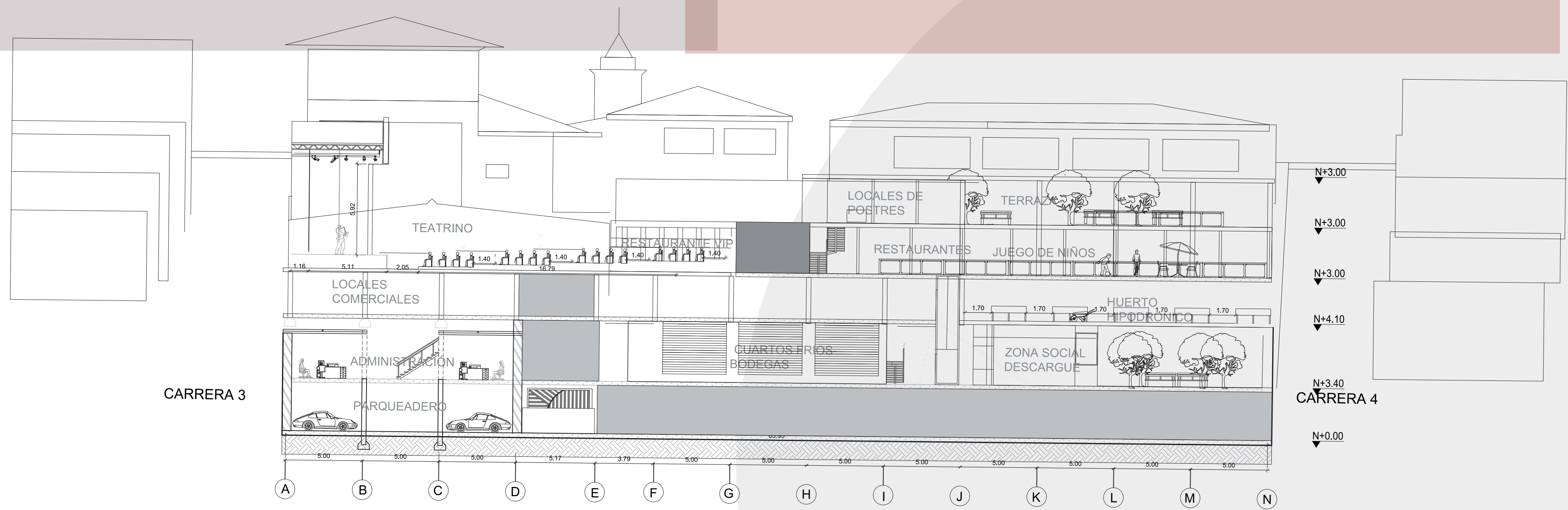
SECCIÓN LONGITUDINAL C-C ESC 1:200
