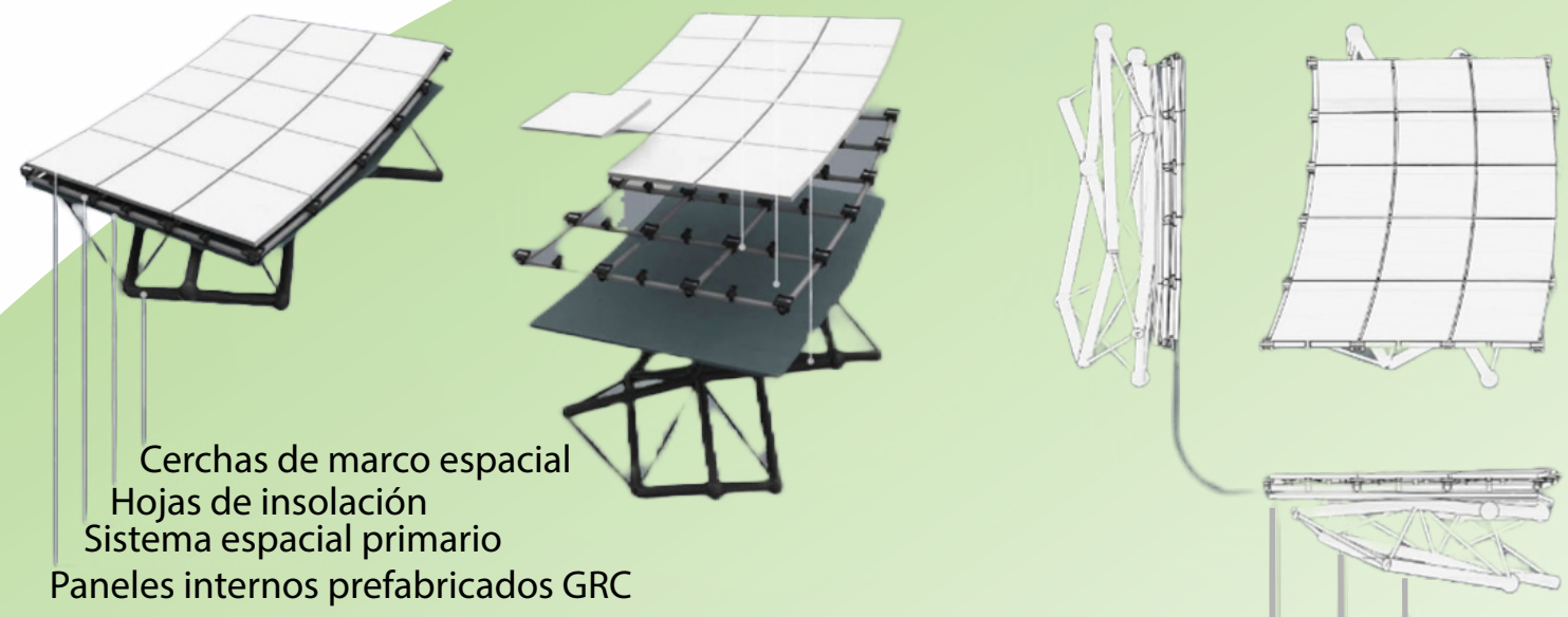
Paneles internos prefabricados GRC
