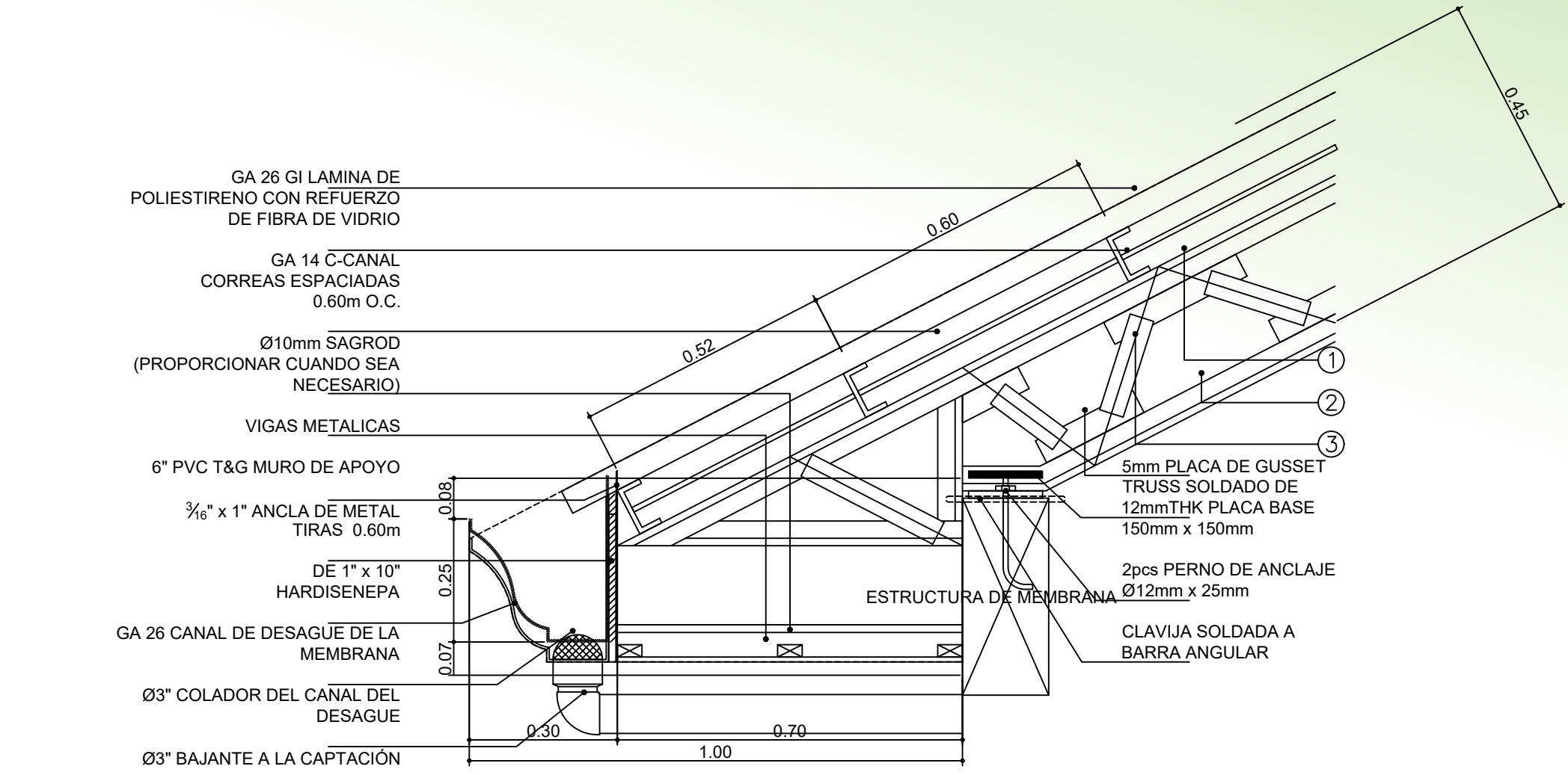
DETALLE ESTRUCTURAL DE PANELES SCALE 1:10M
