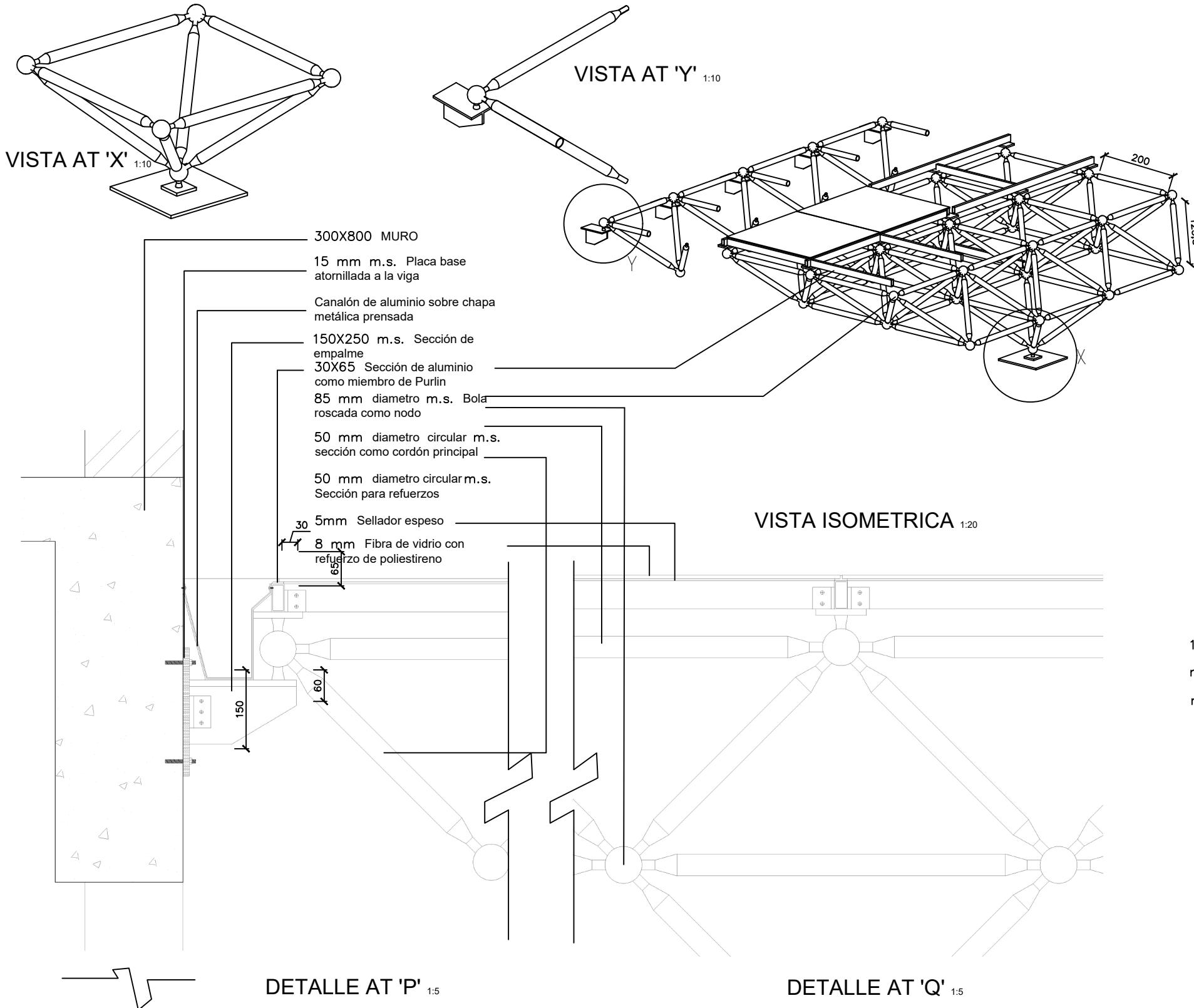
DETALLE ESTRUCTURAL DE PANELES SCALE 1:10M
