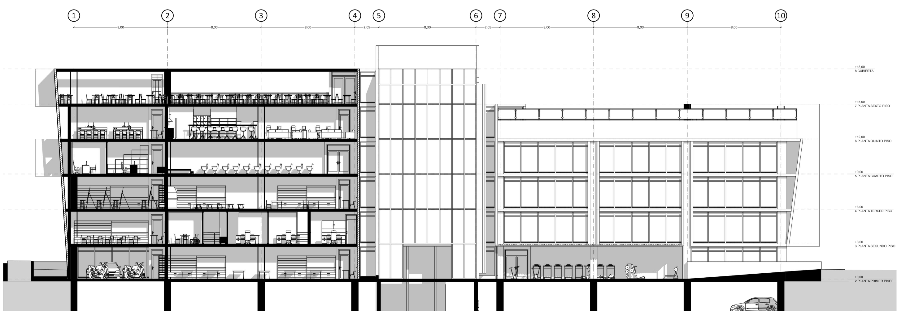
CORTE A
