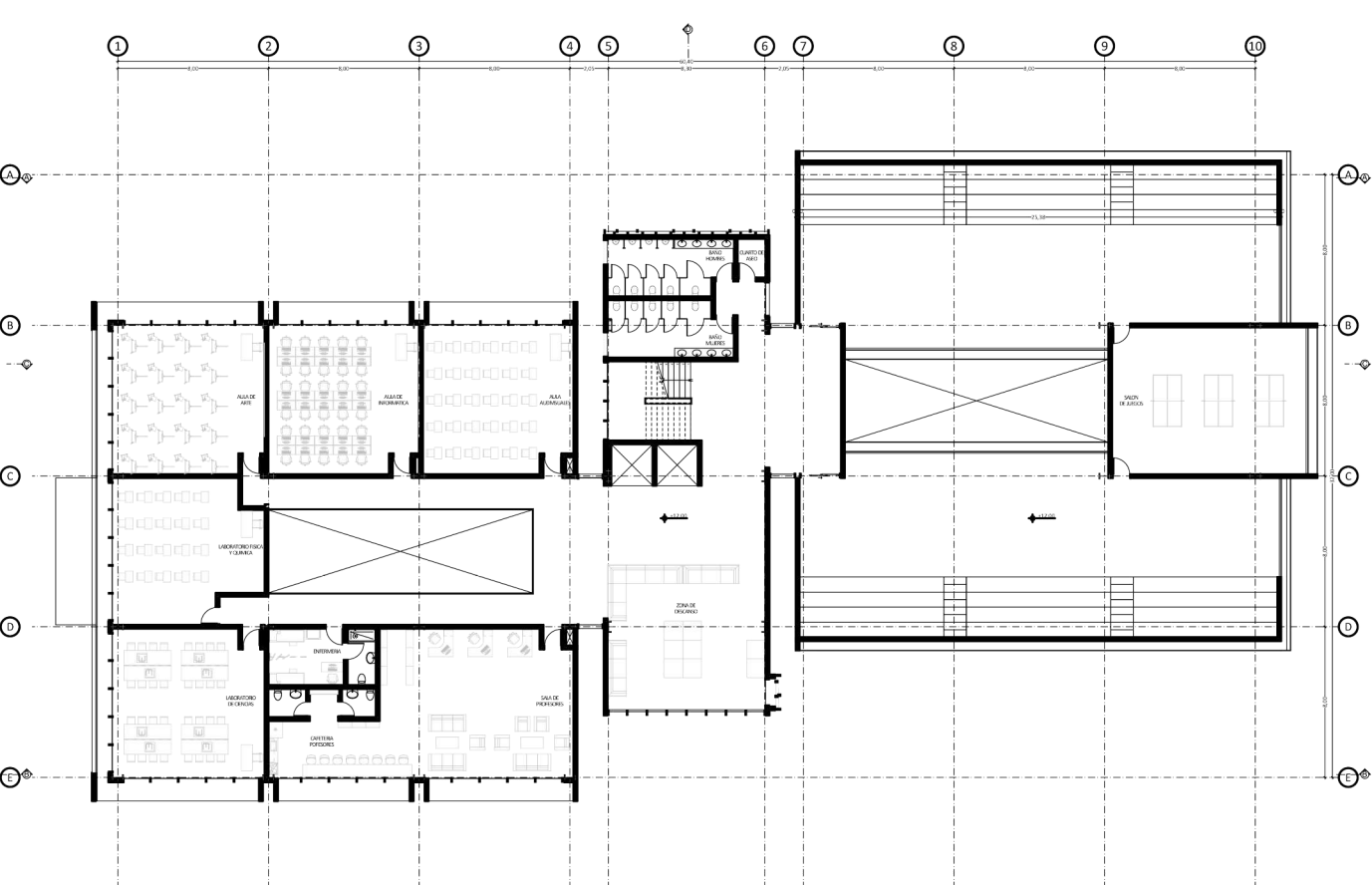
QUINTO PISO
