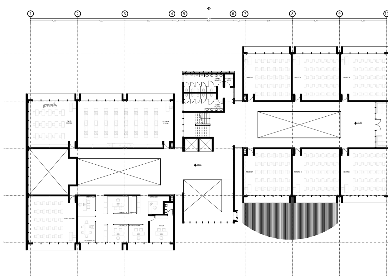
SEGUNDO PISO
