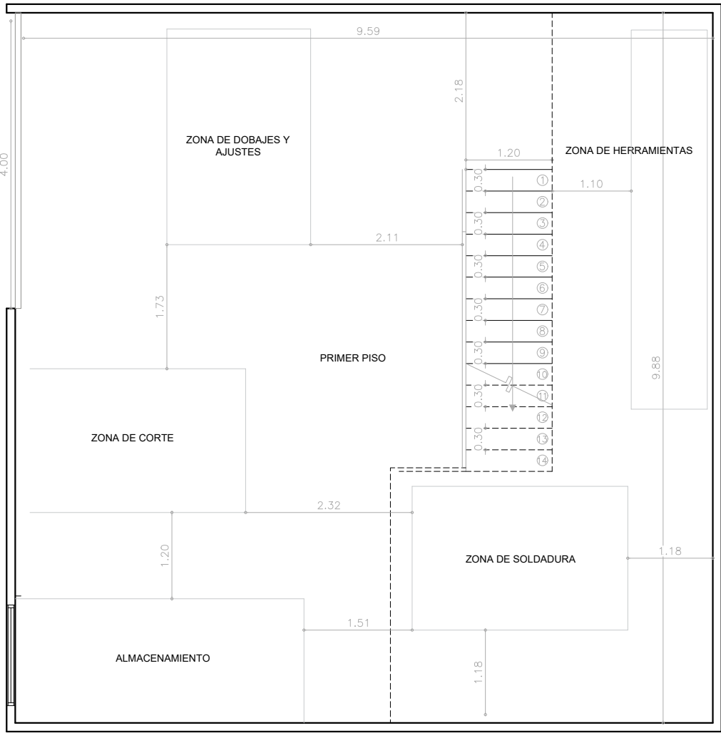
A-1 TALLER DE HERRERIA ESC.... 1:75
