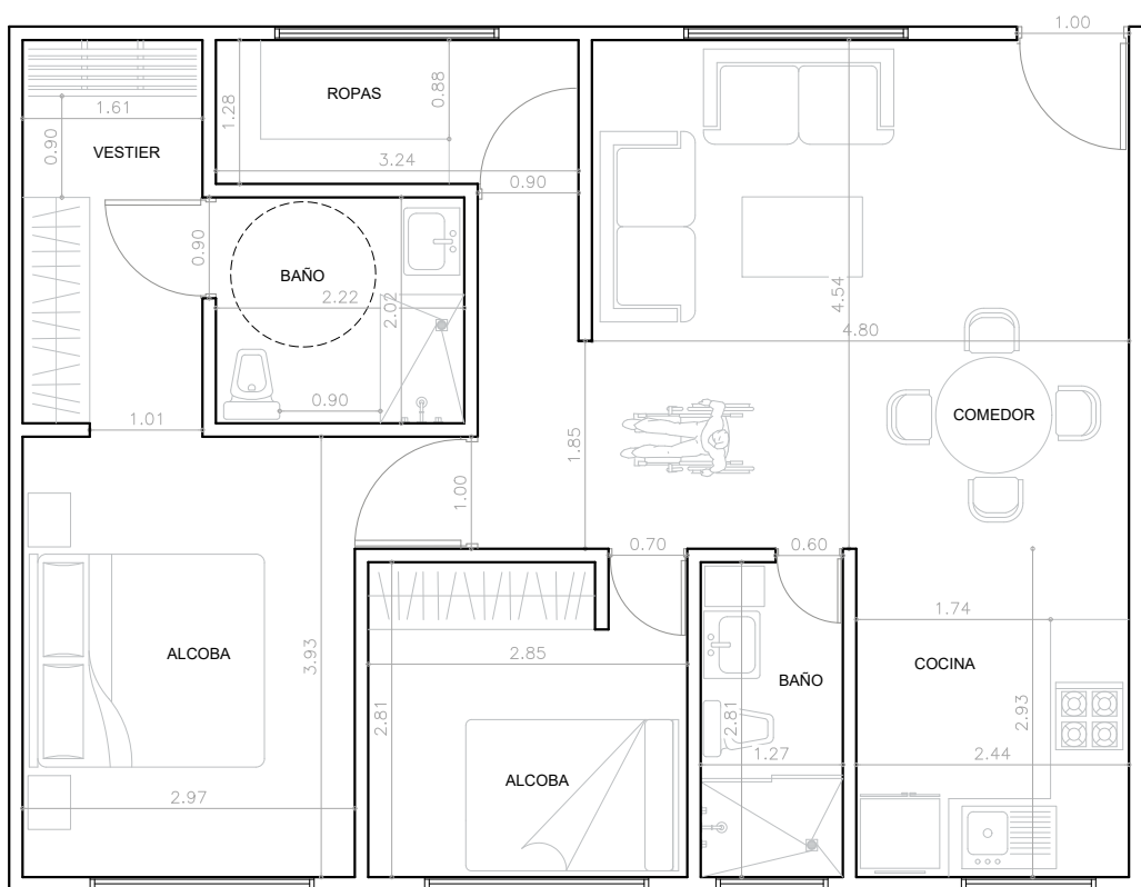
A-1 PLANTA TIPOLOGIA 2 ESC.... 1:75
