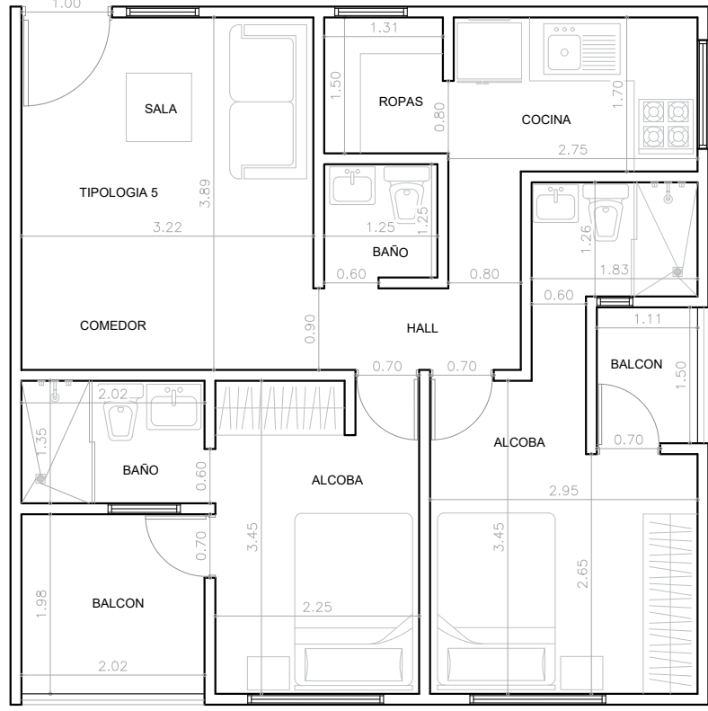
A-1 PLANTA TIPOLOGIA 5 ESC.... 1:75
