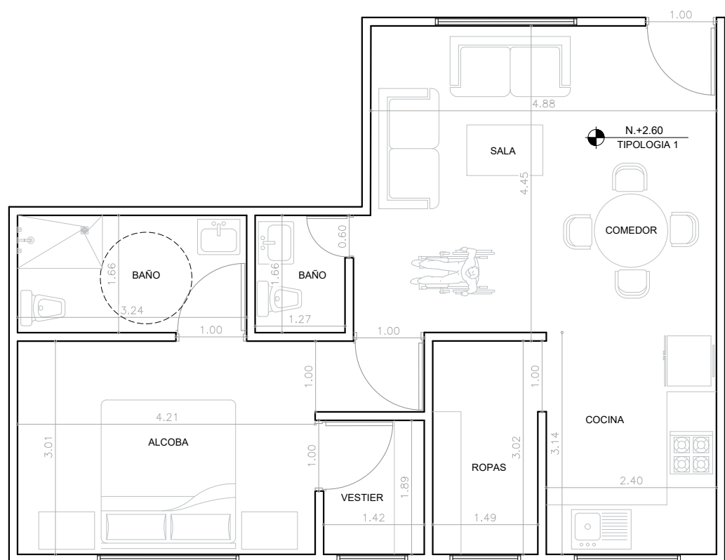
A-1 PLANTA TIPOLOGIA 1 ESC.... 1:75
