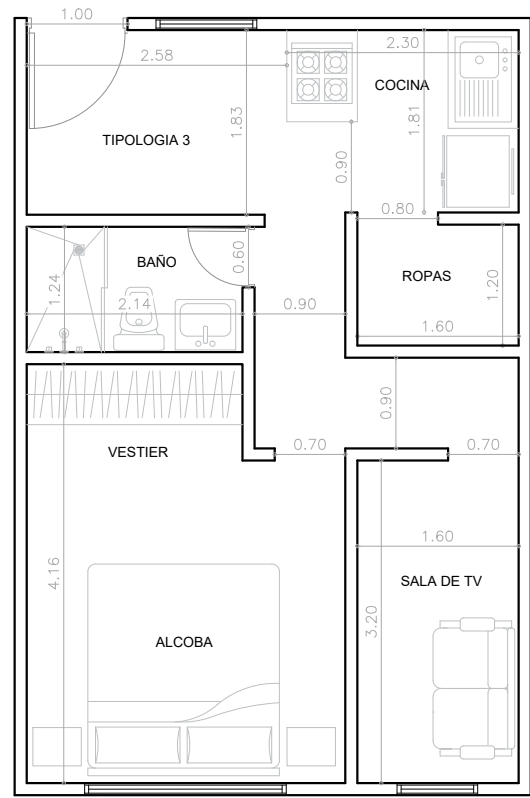
A-1 PLANTA TIPOLOGIA 3 ESC.... 1:75
