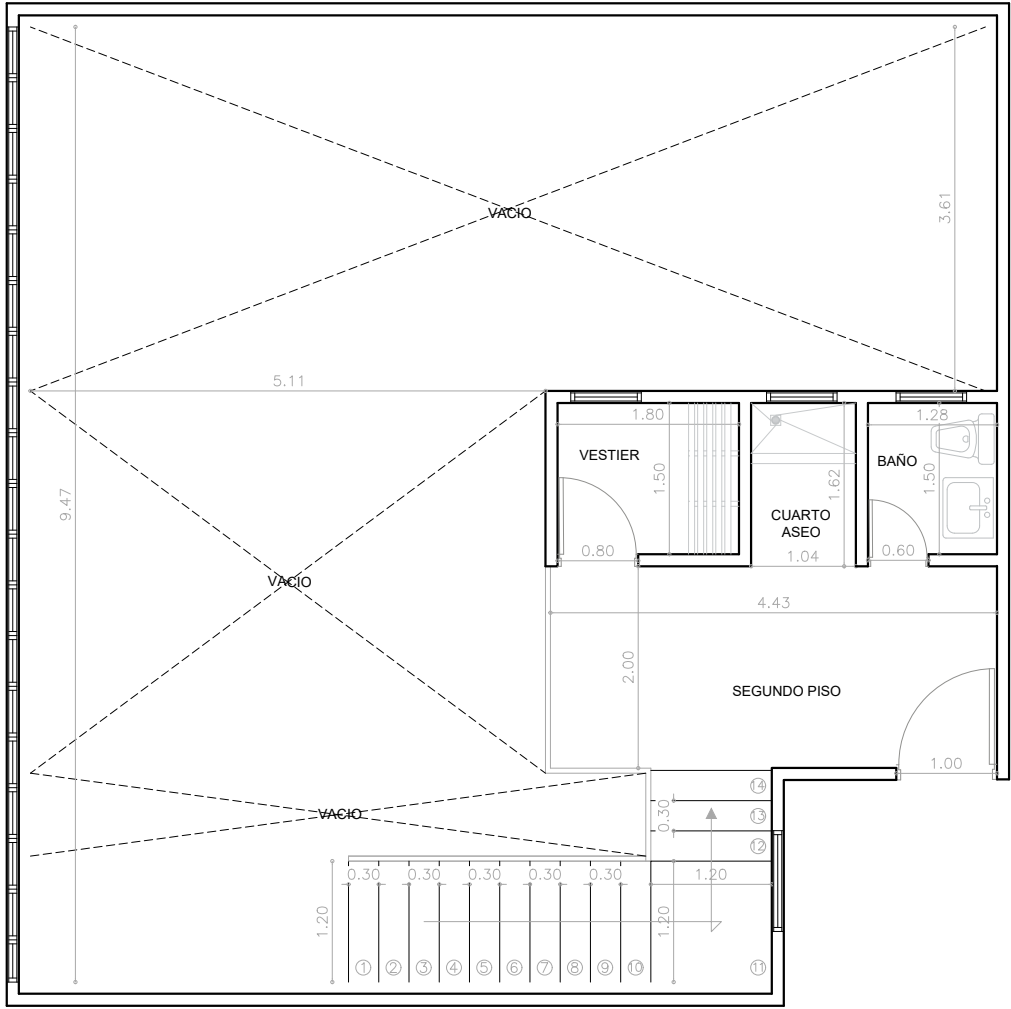
A-1 TALLER DE CARPINTERIA ESC.... 1:75
