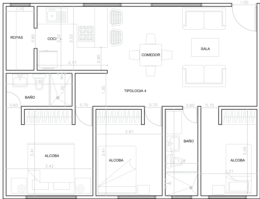
A-1 PLANTA TIPOLOGIA 4 ESC.... 1:75
