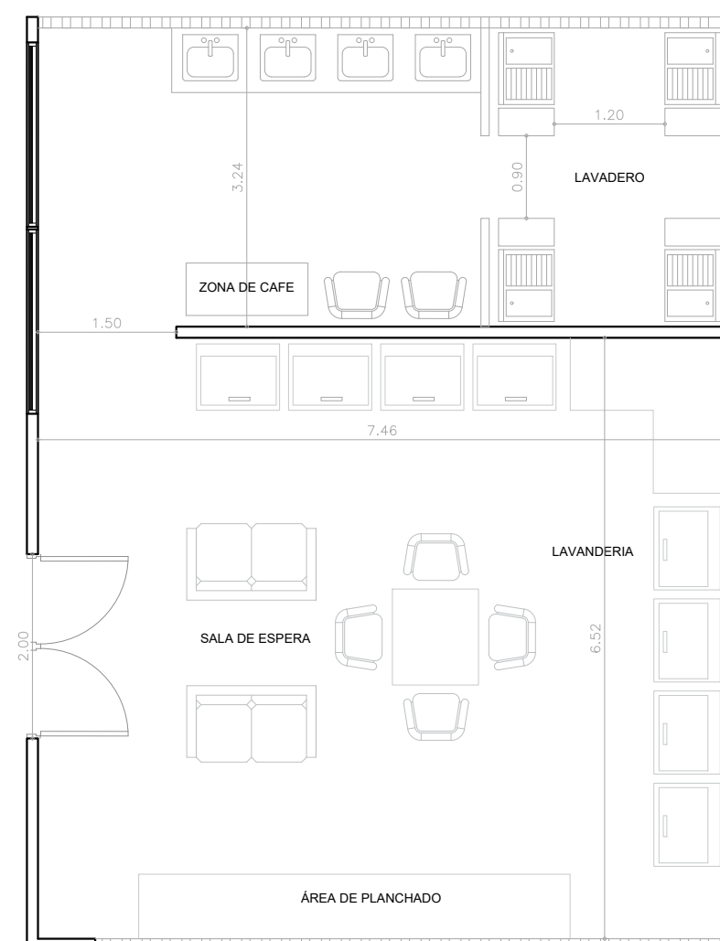
A-1 LAVANDERIA ESC.... 1:75
