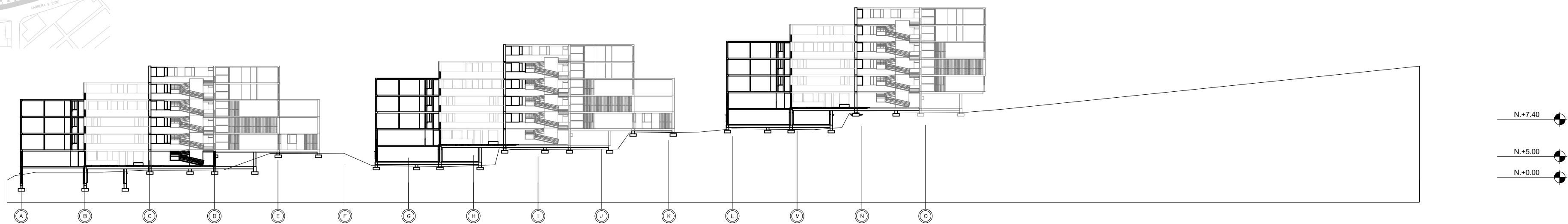
A-1 CORTE B-B ESC.... 1:500
