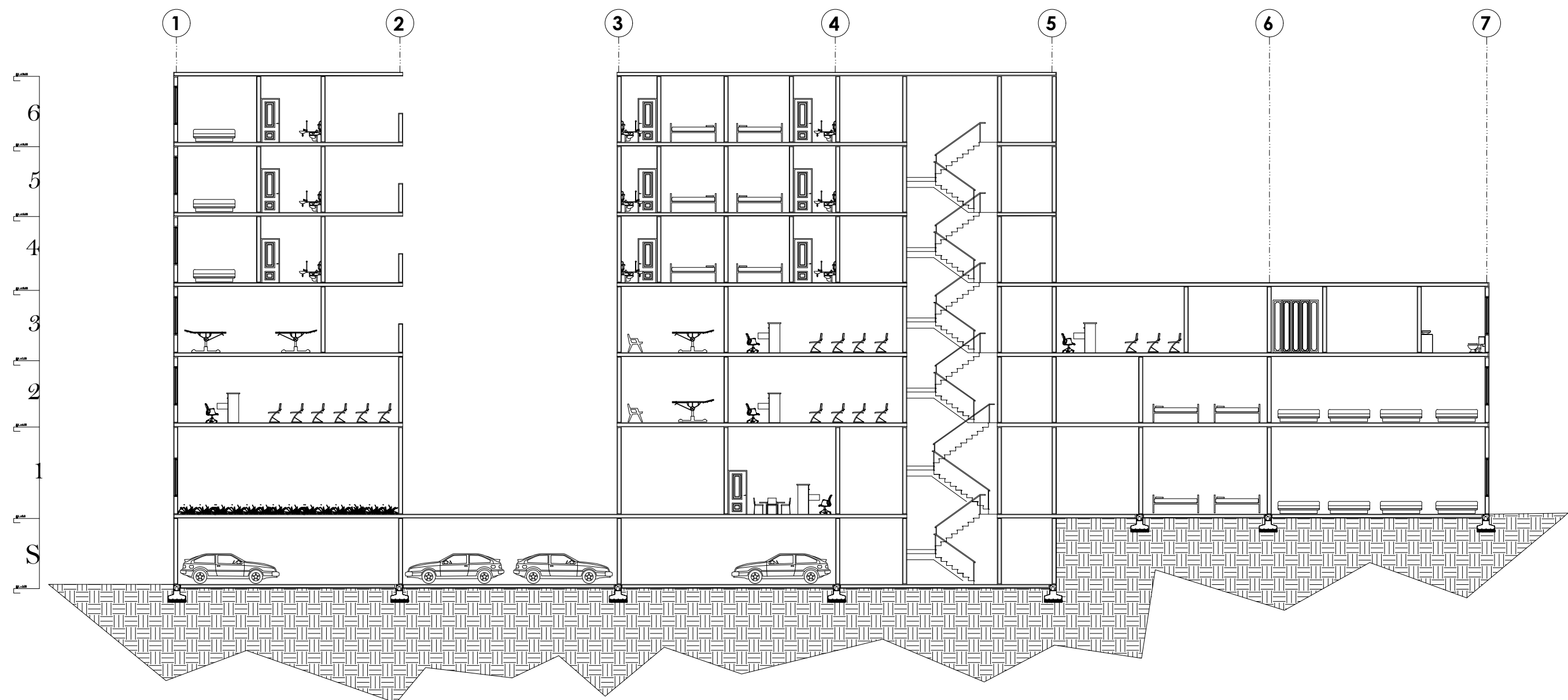
CORTE TRANSVERSAL 0 20 40 60 80 100 200 ESCALA 1/200
