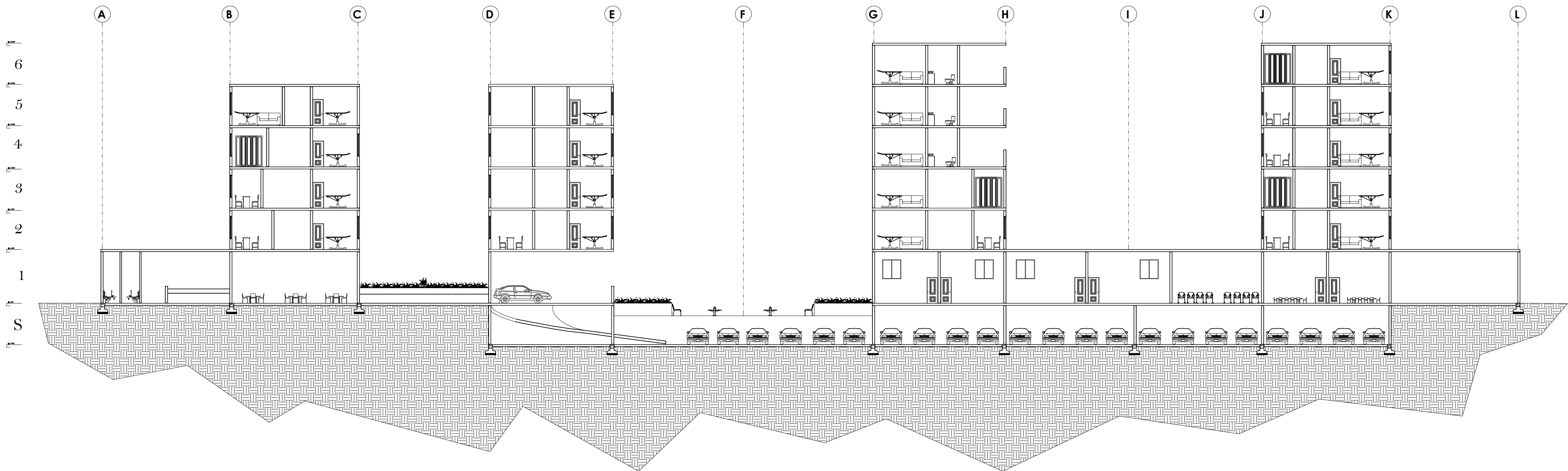
CORTE LONGITUDINAL 0 20 40 60 80 100 200 ESCALA 1/200
