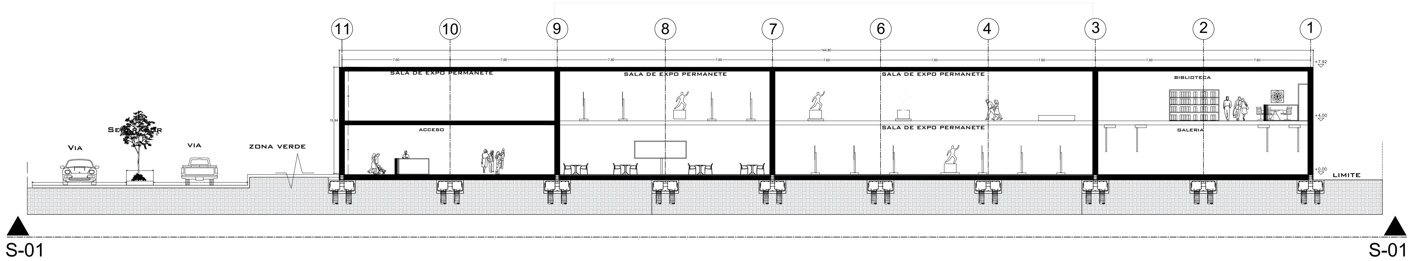
Seccion Longitudinal Esc: 1_150 S1
