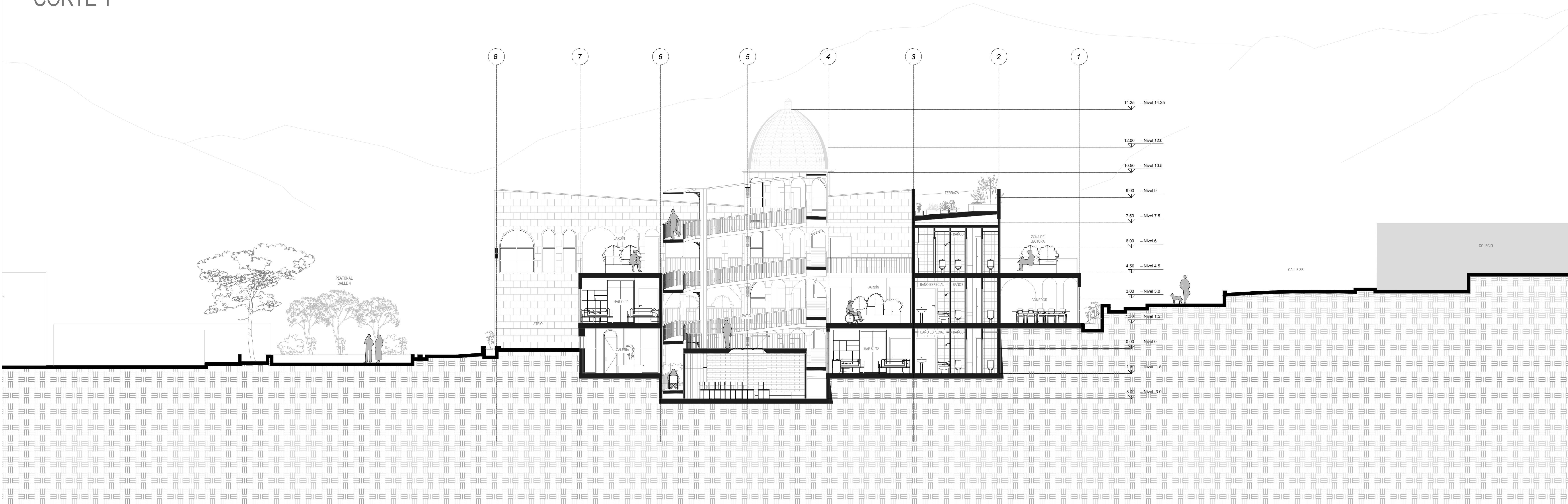
CORTE 1
