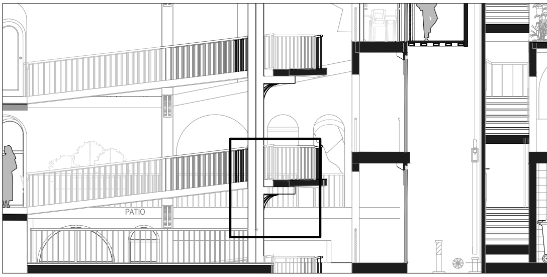
DETALLE 5 / ZAPATA ESC 1:20
