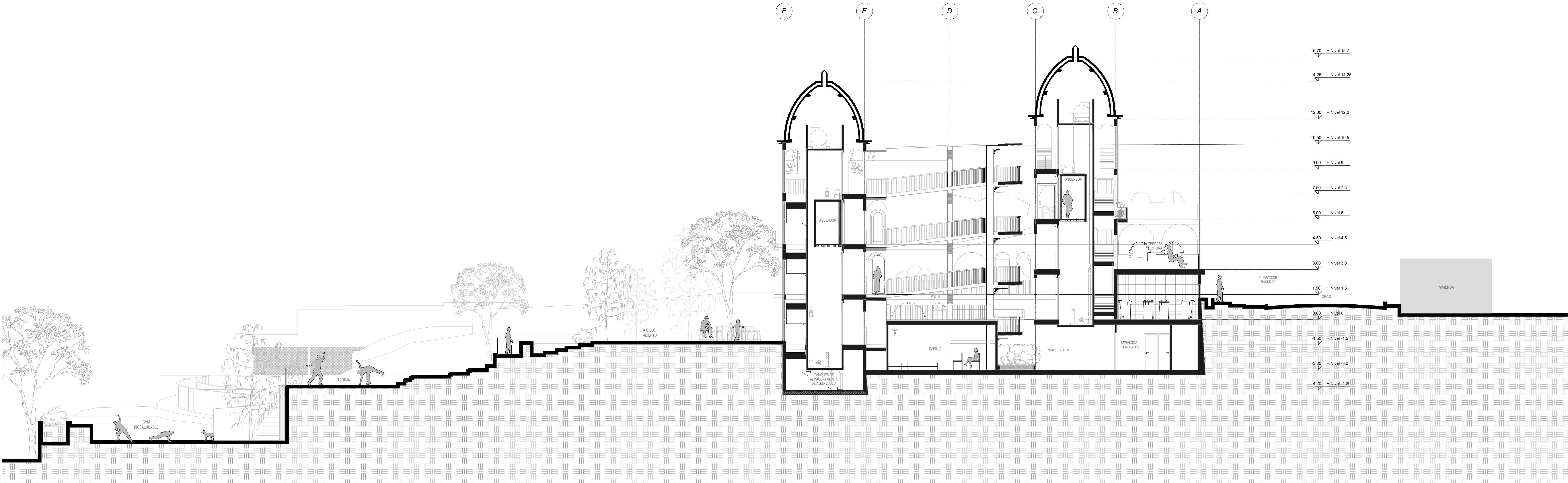
CORTE 2
