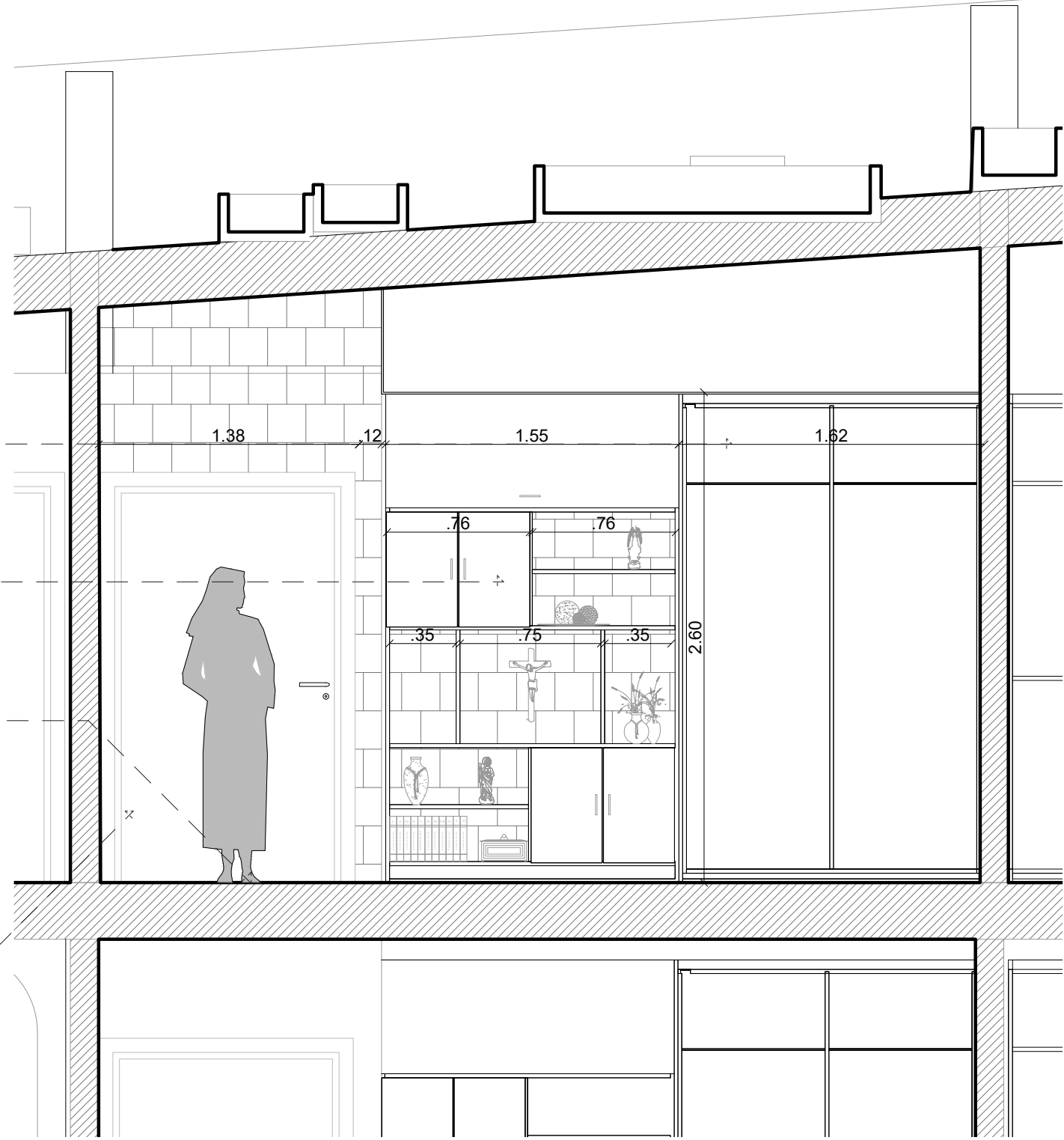
CORTE ESC 1:25
