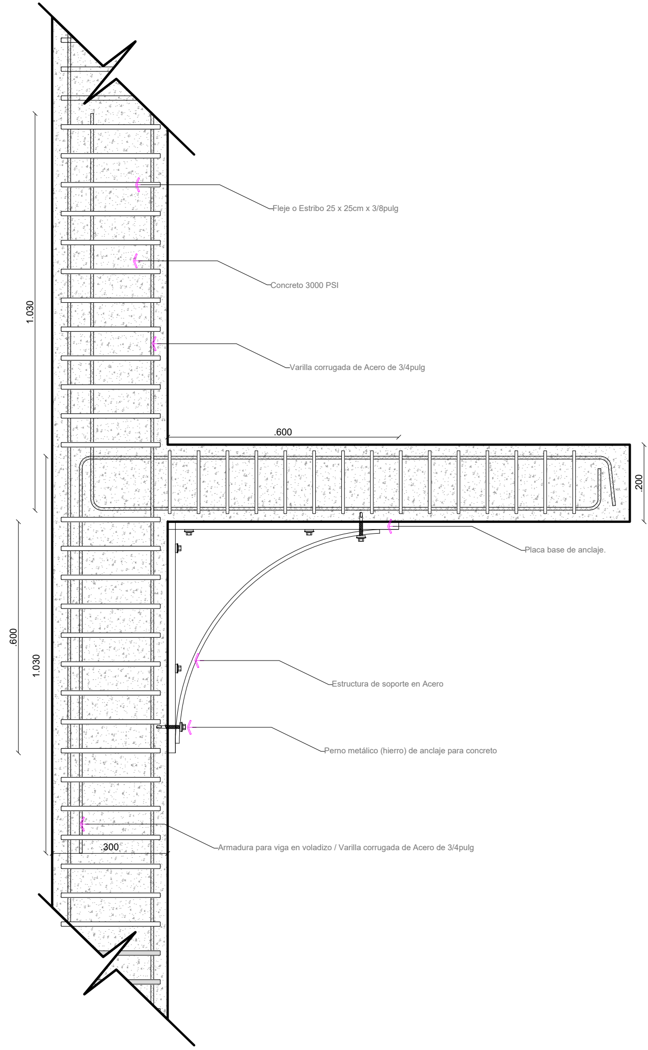
DETALLE 1 / COLUMNA CON VIGA EN VOLADIZO ESTRUCTURAL ESC 1:10
