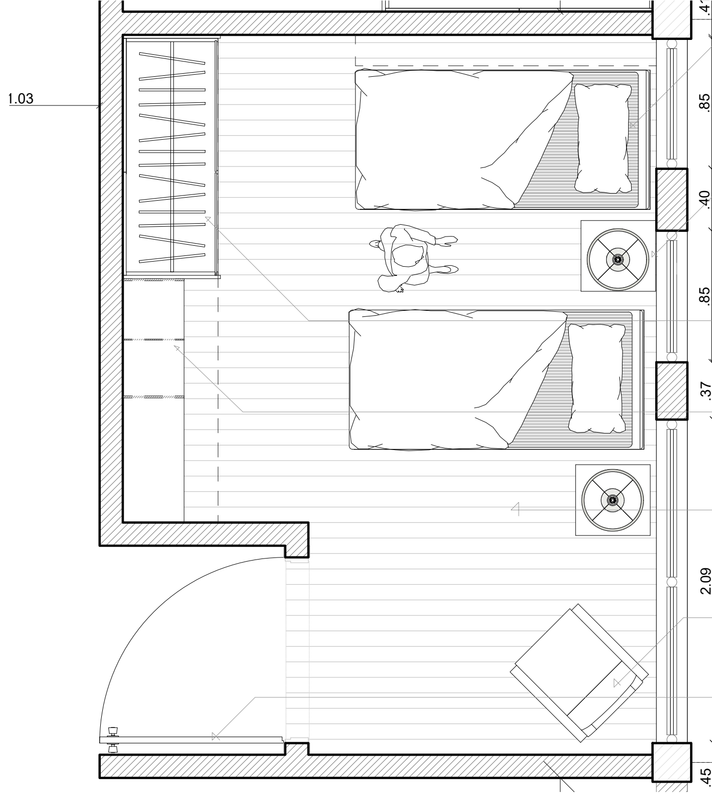
PLANTA ESC 1:25
