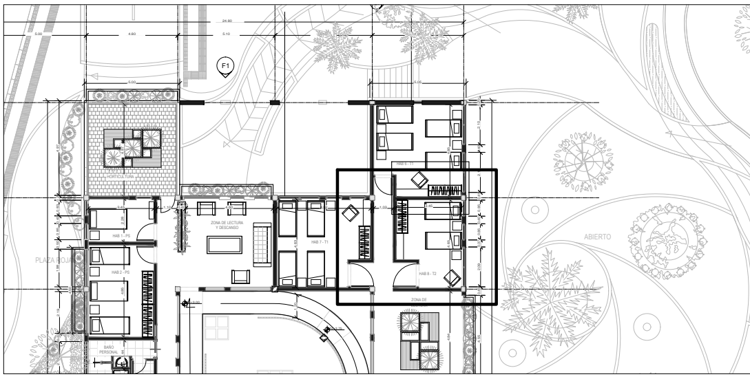
PLANTA ESC 1:25
