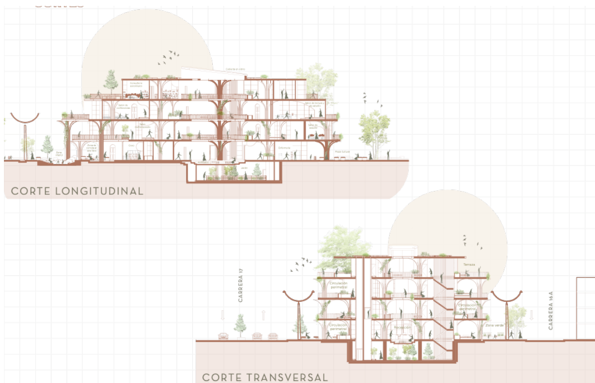
Ilustración 26: Corte longitudinal y transversal Centro de Integración Venus. Elaboración propia. 2022.
