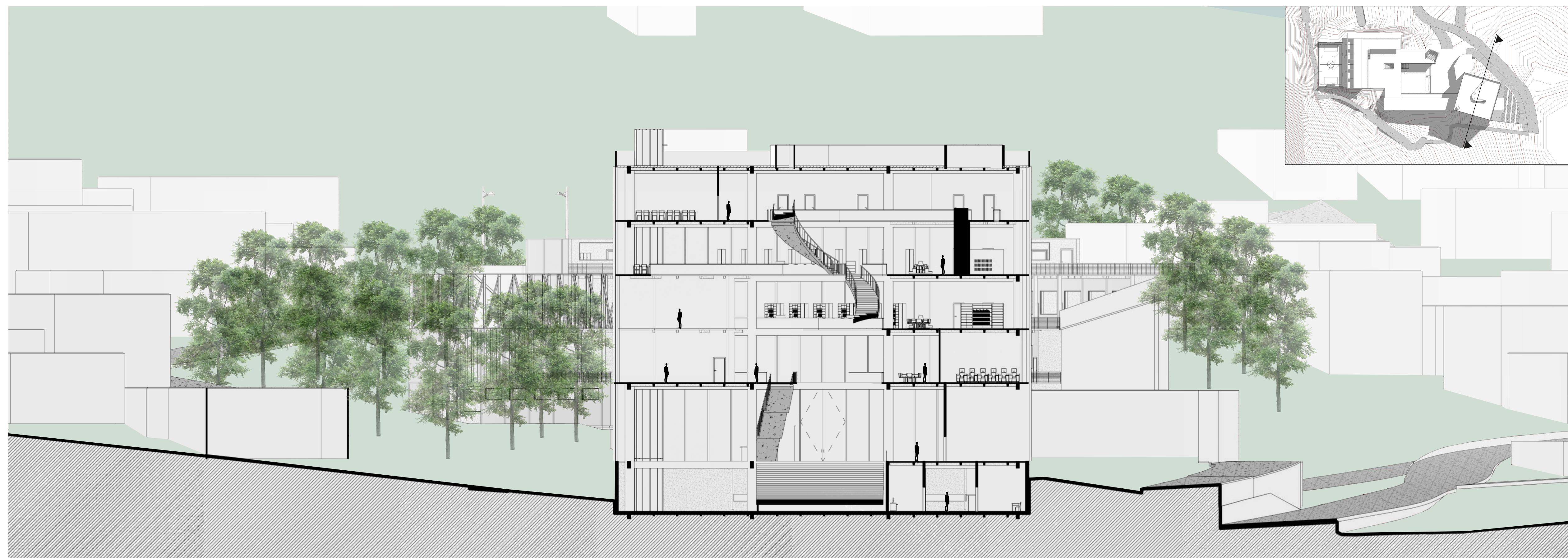
Sección Transversal
