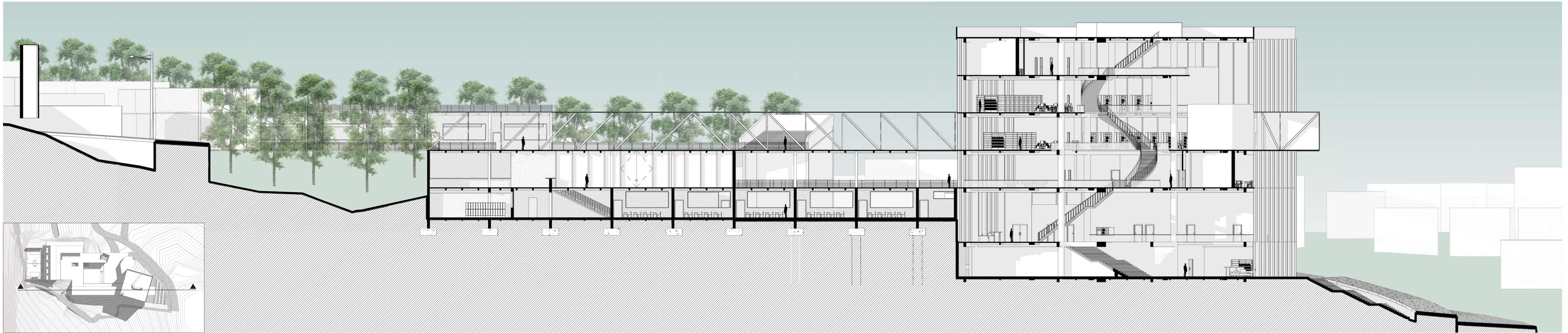
Sección Longitudinal
