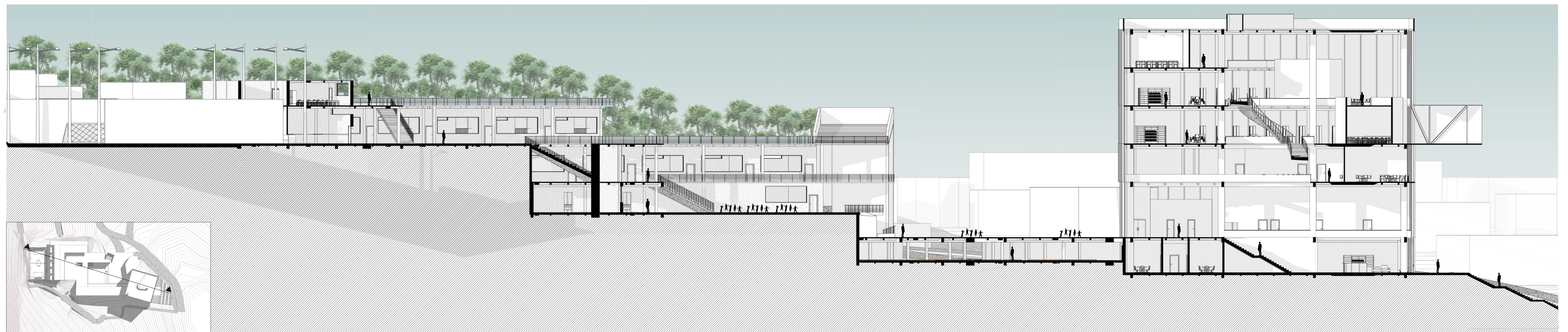
Sección Longitudinal
