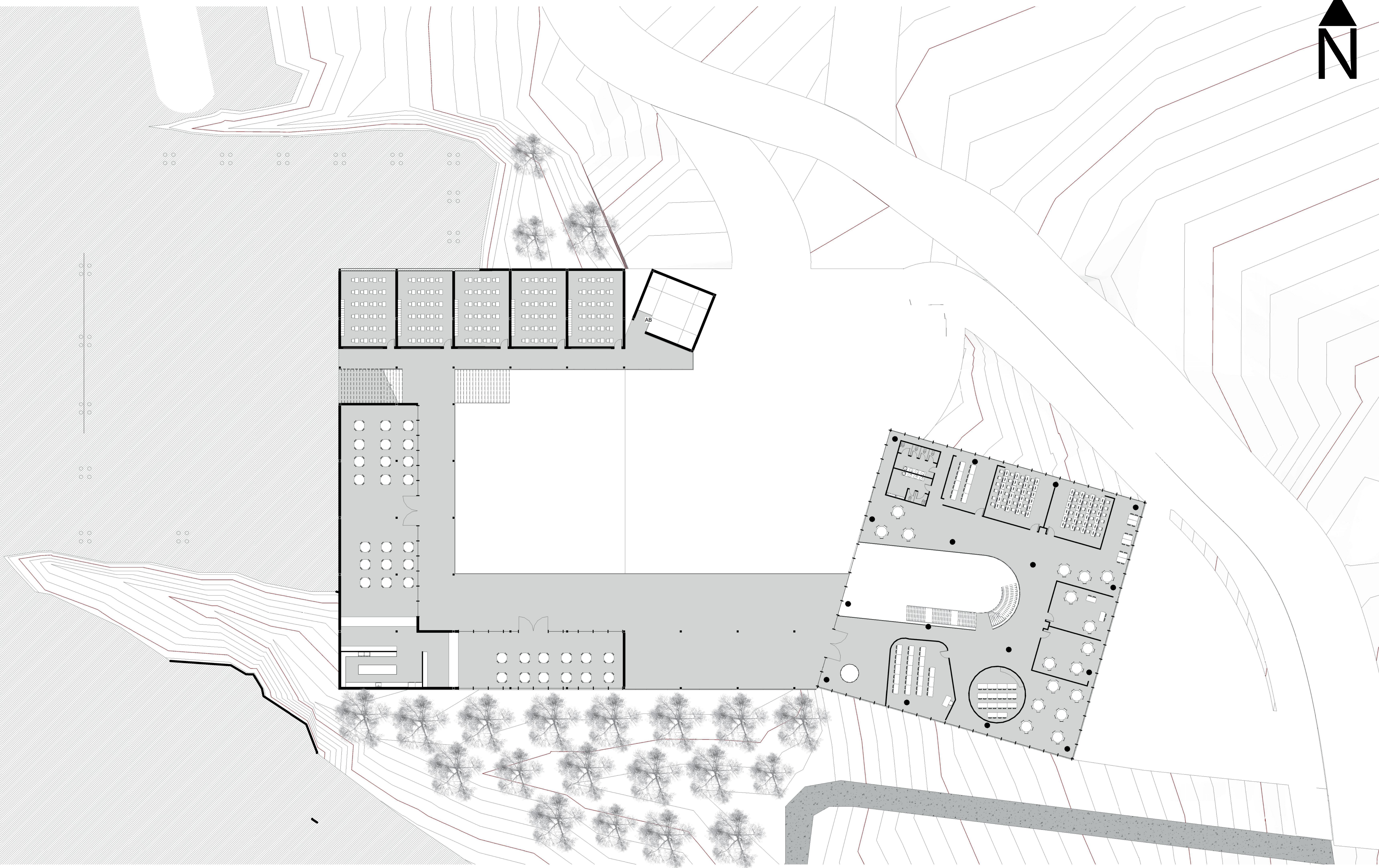
Planta Nivel 3
