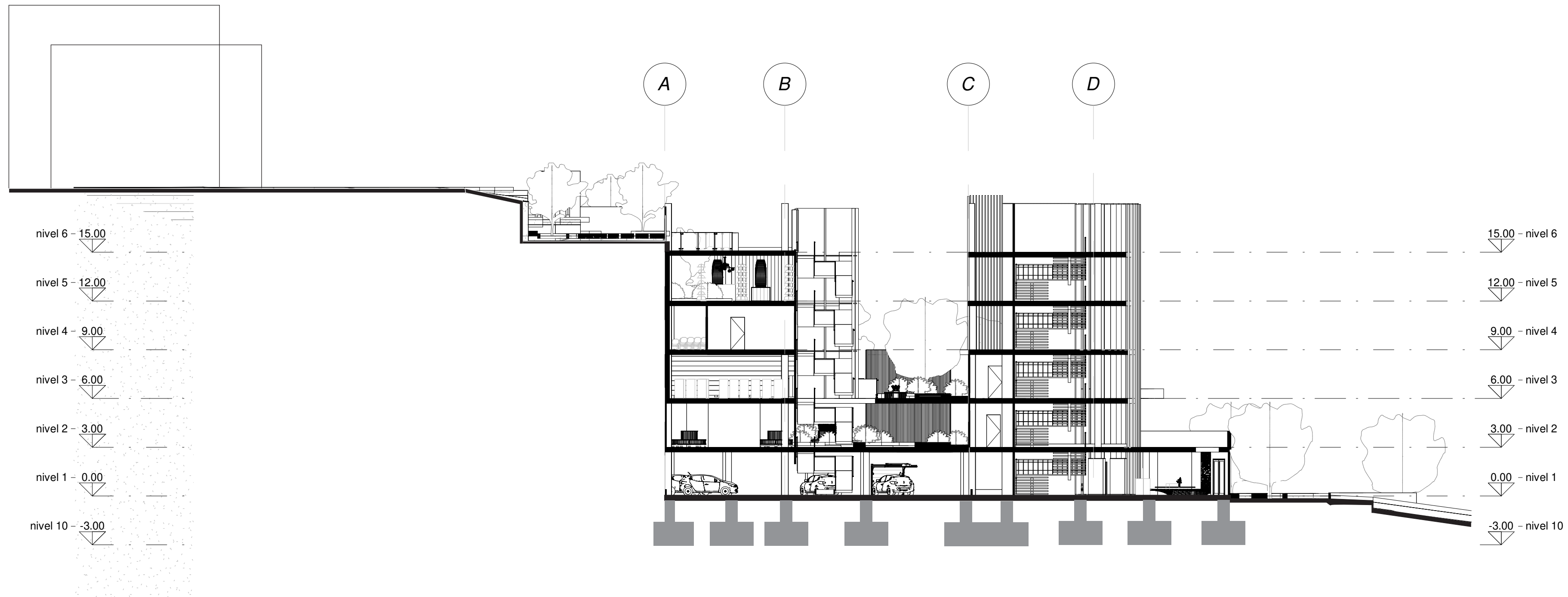
3 Sección 3 A108 1 : 200
