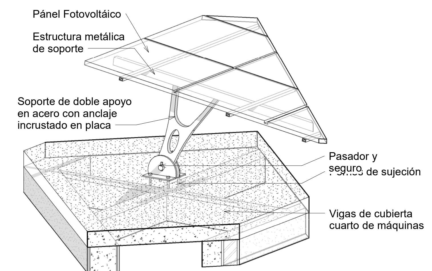
5 DET ANCLAJE PANELES
