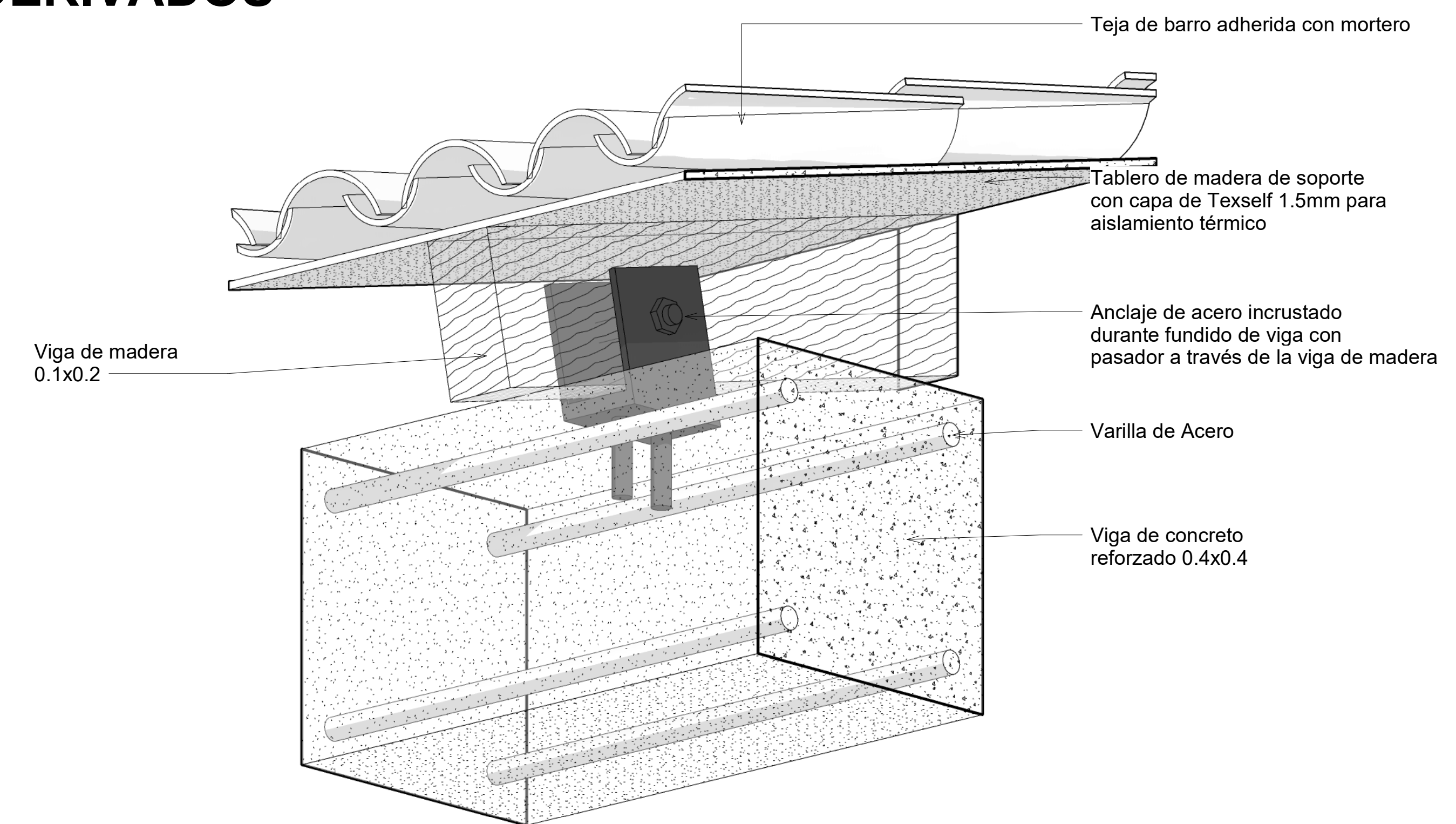
3 DET ANCLAJE 3D
