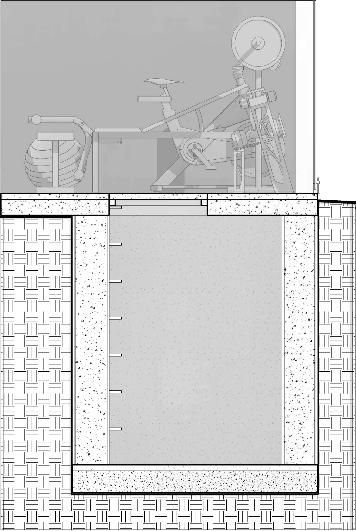
4 TANQUE AGÜA
