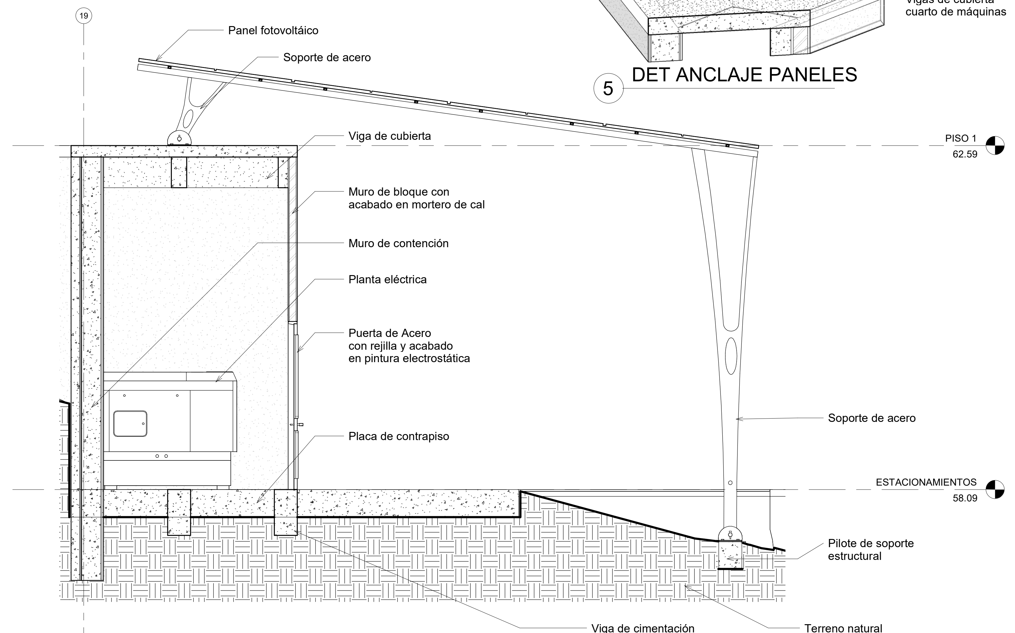
6 CUBIERTA PARQUEO 1 : 30
