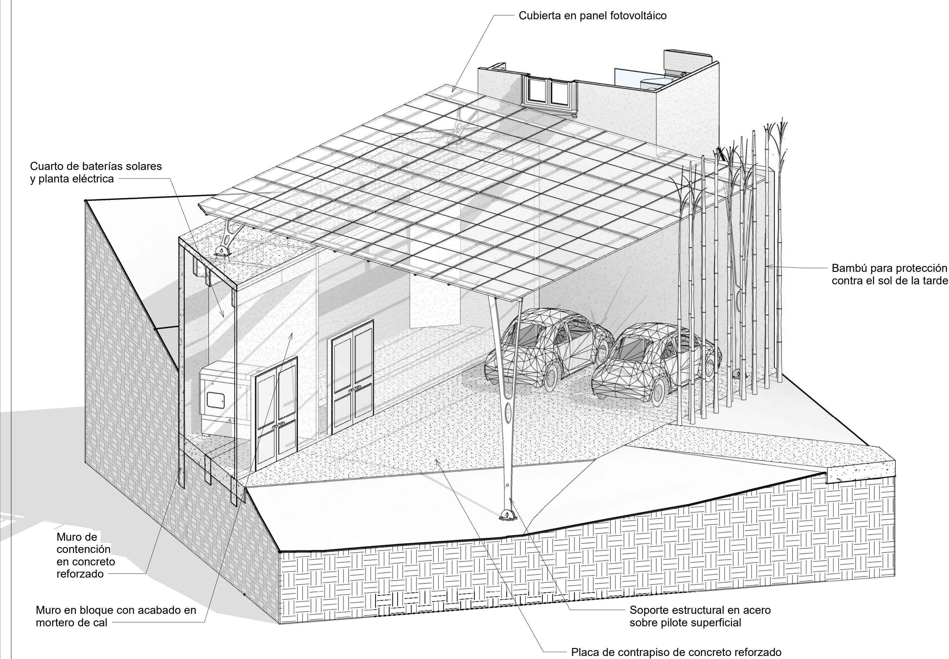
4 DET CUBIERTA PARQUEO
