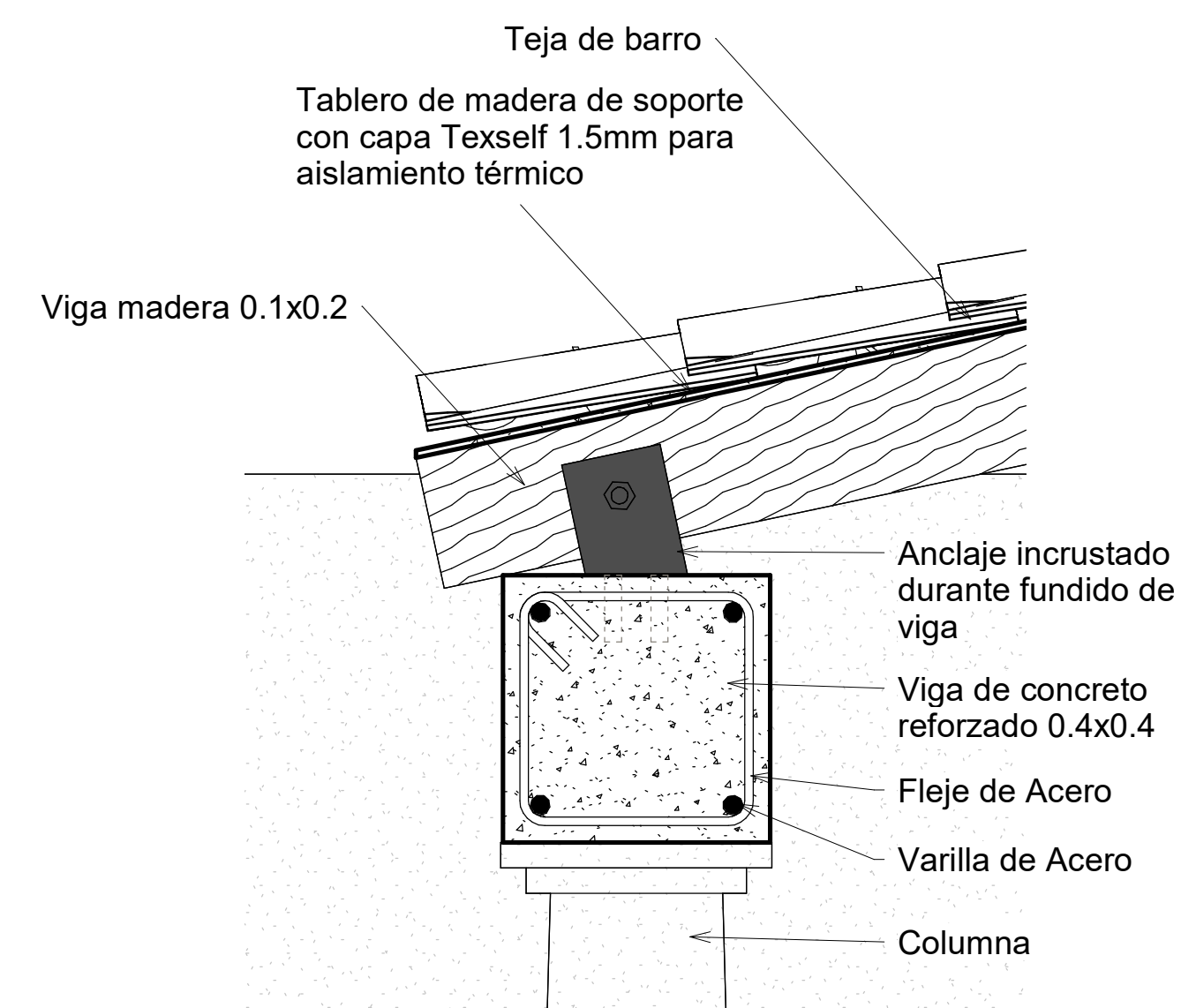
2 VIGA Y ANCLAJE 1 : 10
