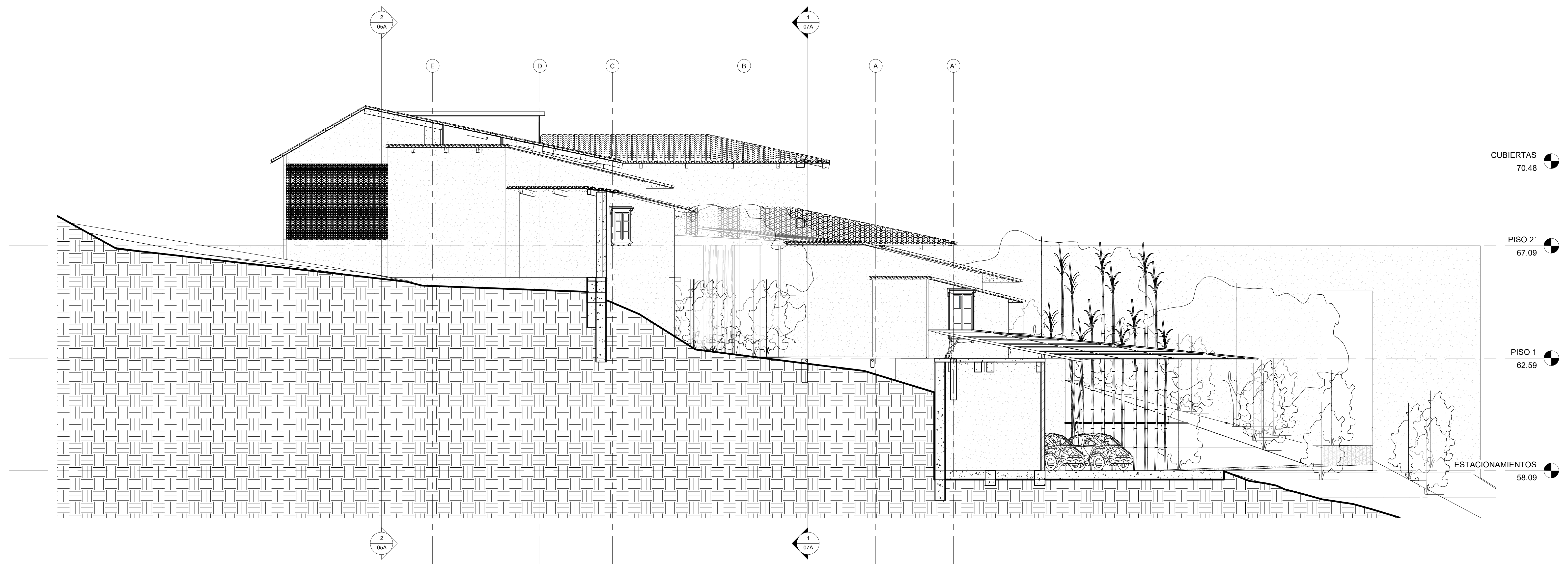
2 FACHADA ESTE 1:75
