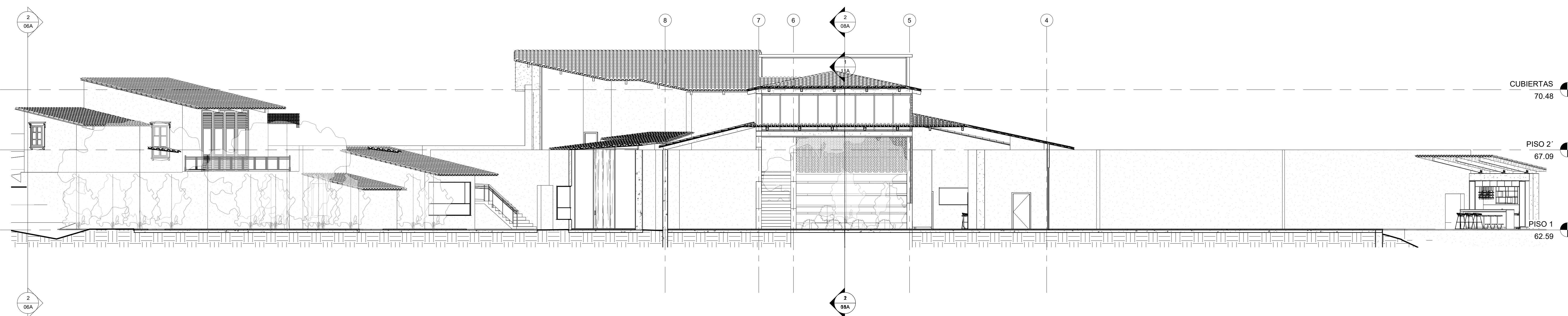
1 CORTE LONGITUDINAL 1 1 : 100
