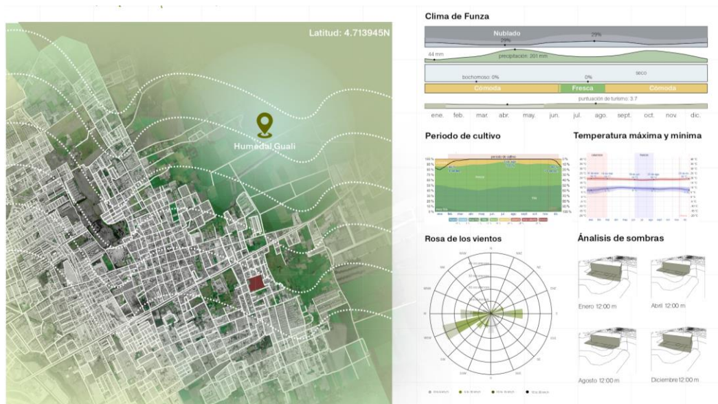
Ilustración 7. Datos climáticos Funza, Cundinamarca.
