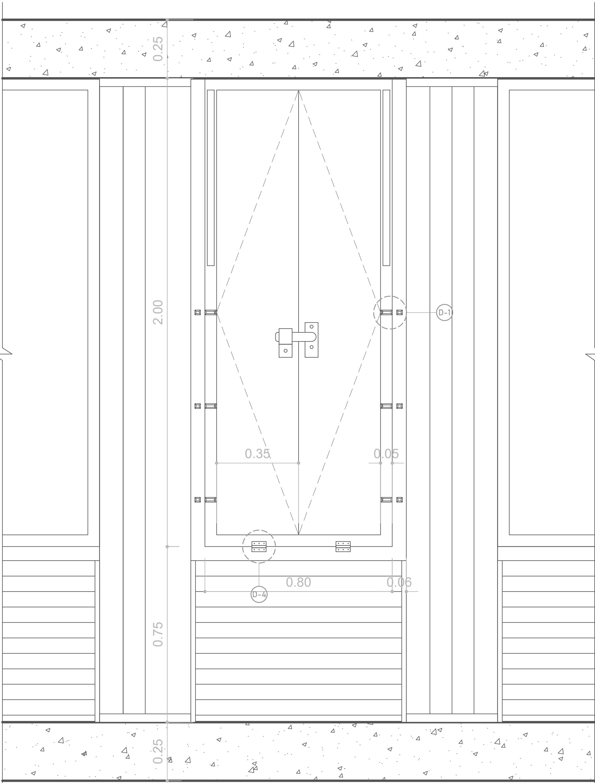
Vista frontal mesa plegada Esc 1:10
