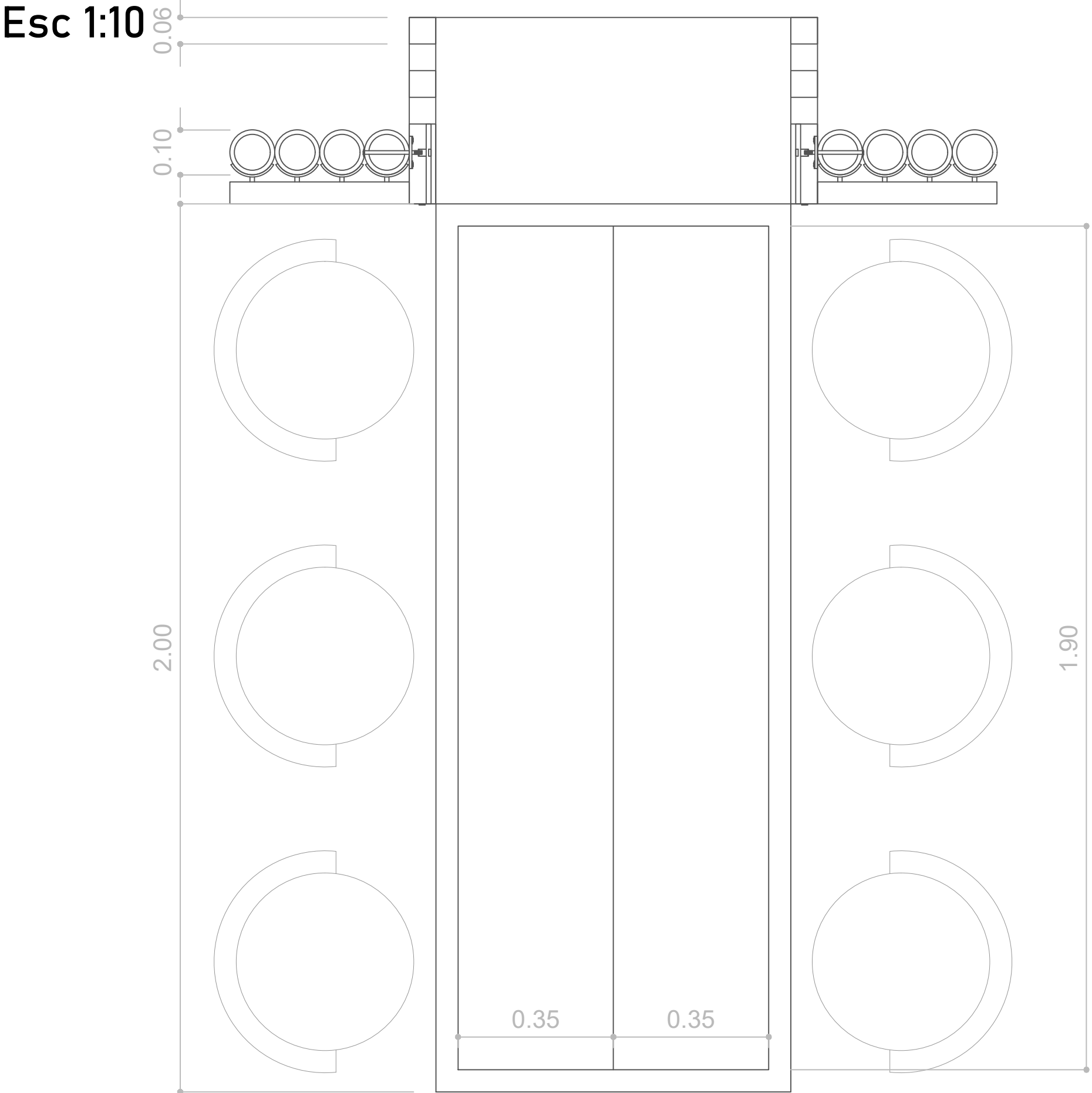
Vista frontal mesa desplegada
