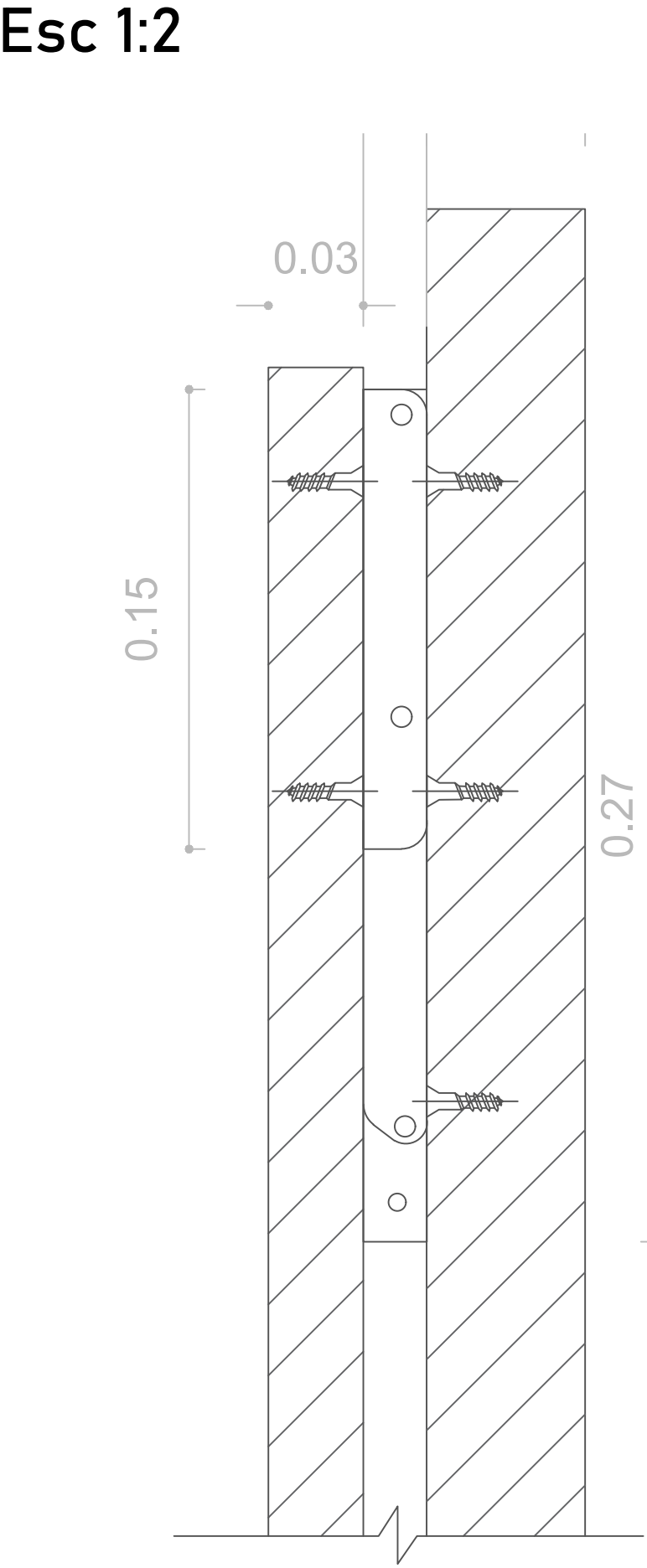
D4- Bisagra en mesa plegada
