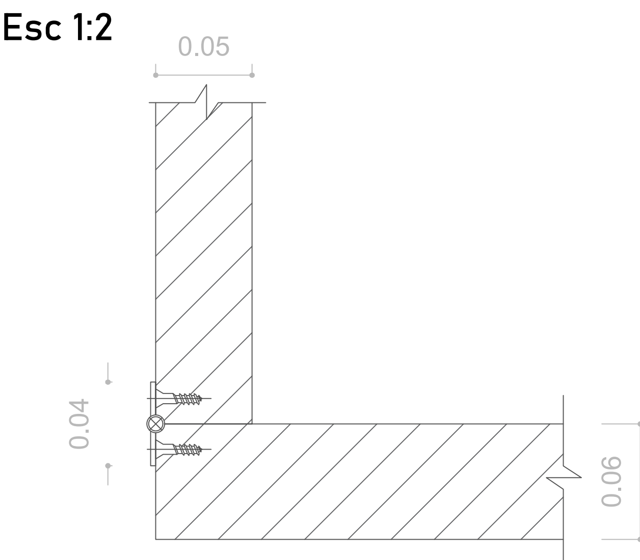
D5- Bisagra en mesa desplegada
