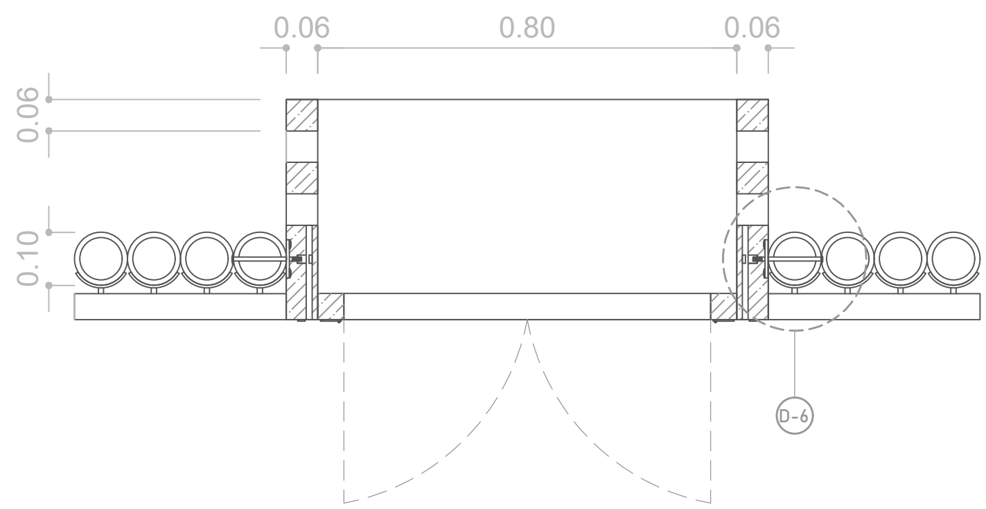
Planta mesa plegada Esc 1:10
