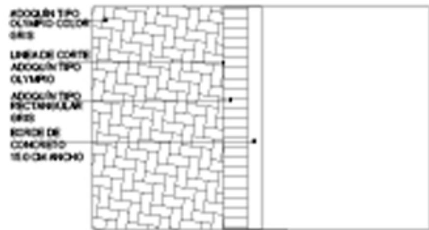
DETALLE ADOQUÍN Y PAVIMENTO DE CONCRETO
