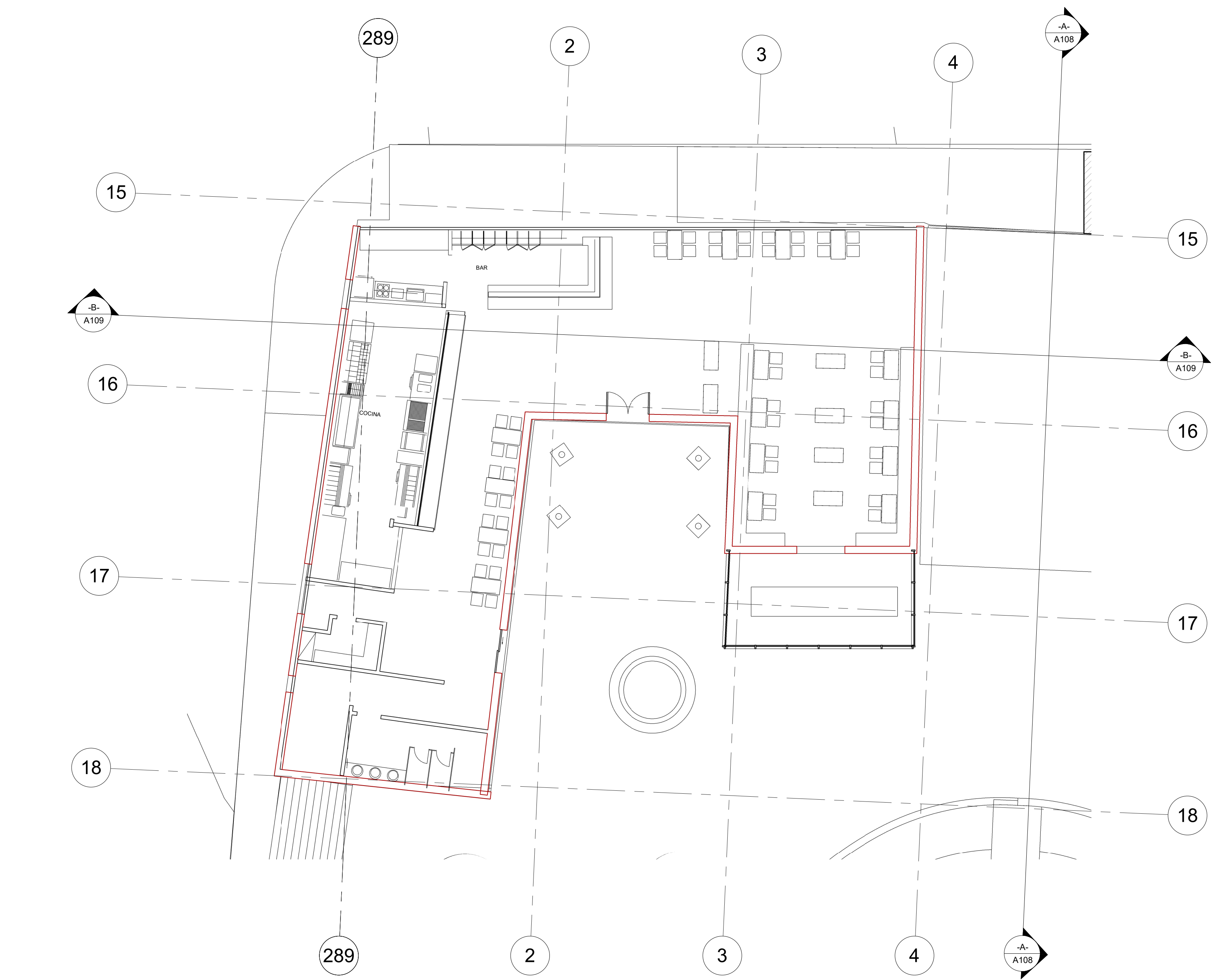
1 Nivel 9 - Llamada 1 1 : 125
