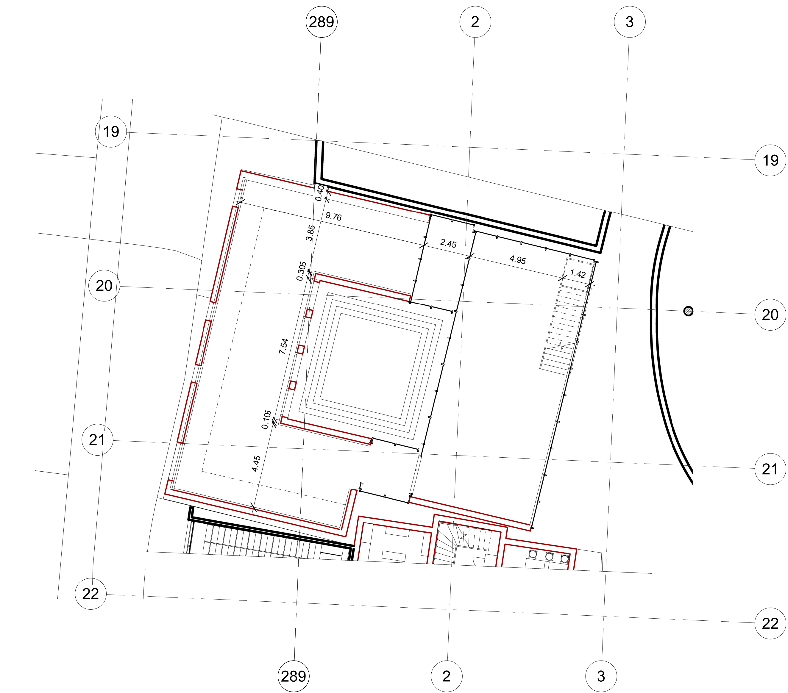
1 Nivel 5 - recinto casa 1 : 125
