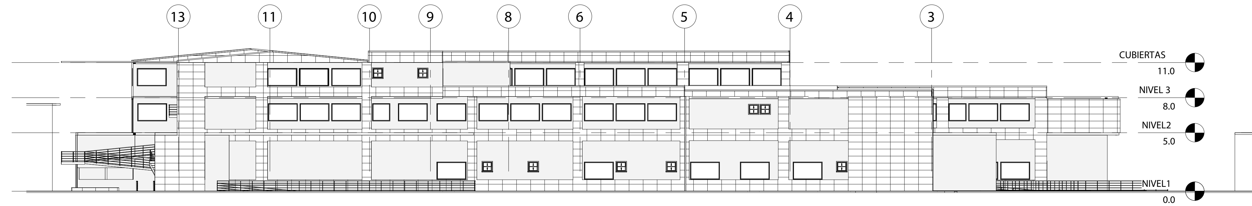
F-1 FACHADA NORESTE 1 : 200
