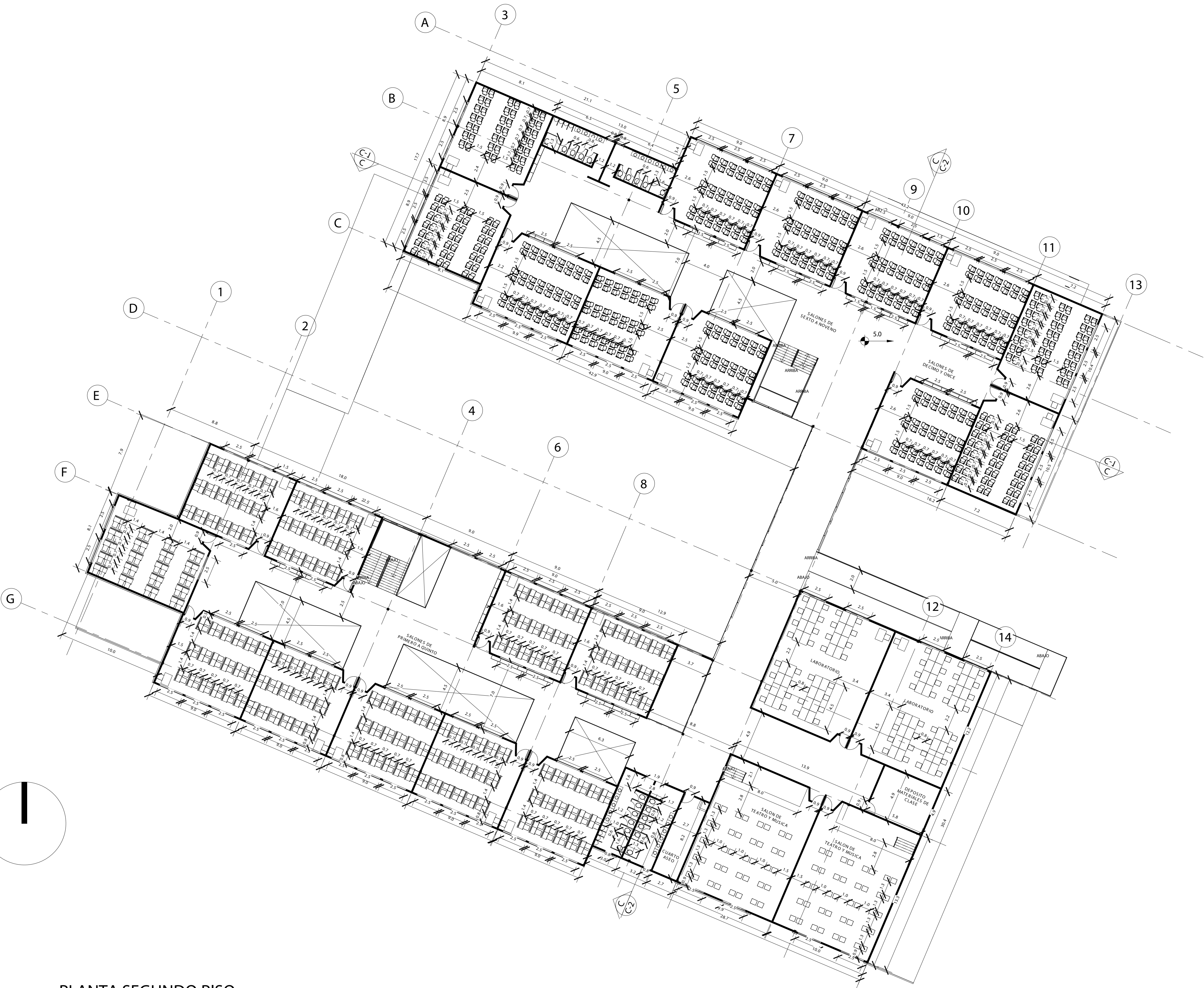
P-2 PLANTA SEGUNDO PISO 1:200
