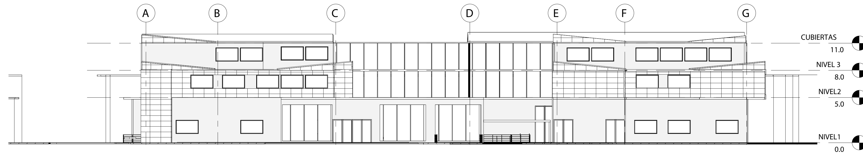
F-2 FACHADA NOROESTE 1 : 200
