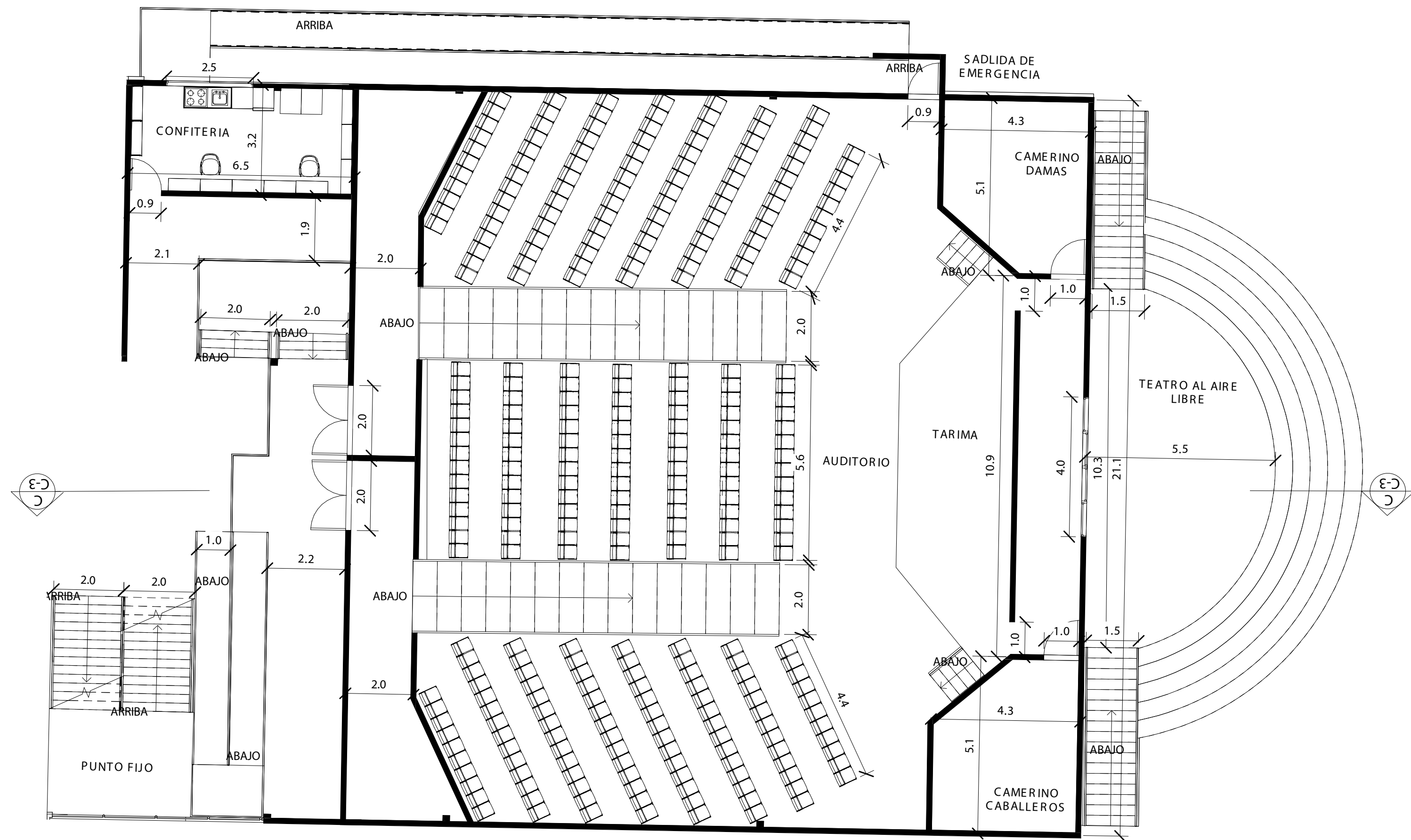
A-1 AMPLIACION AUDITORIO 1 : 100
