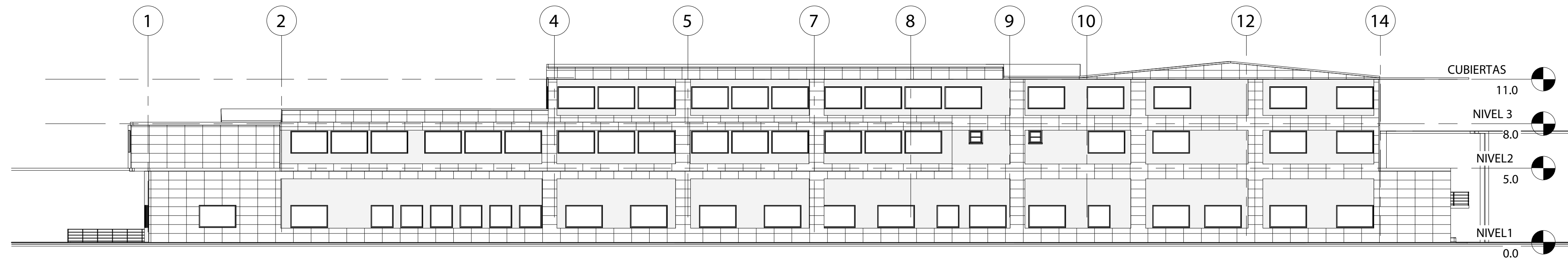
F-3 FACHADA SUROESTE 1 : 200
