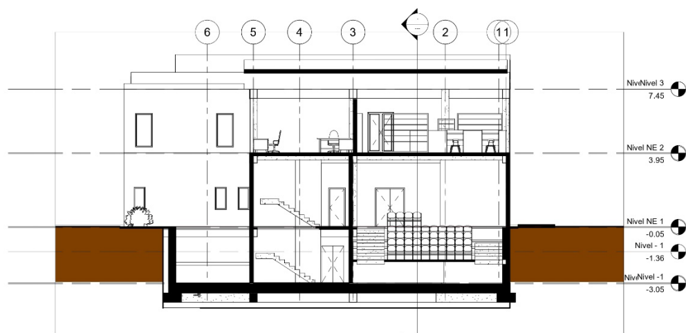
Ilustración 33 Corte transversal Auditorio y biblioteca Esc. gráfica
