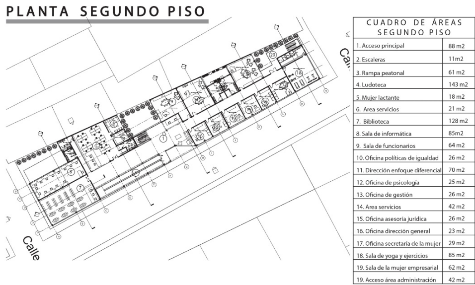
Ilustración 26 Planta general segundo piso con su respectivo cuadro de áreas
