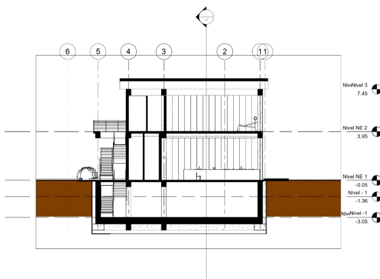
Ilustración 35 Corte transversal taller gastronomía y salón de yoga Esc. gráfica
