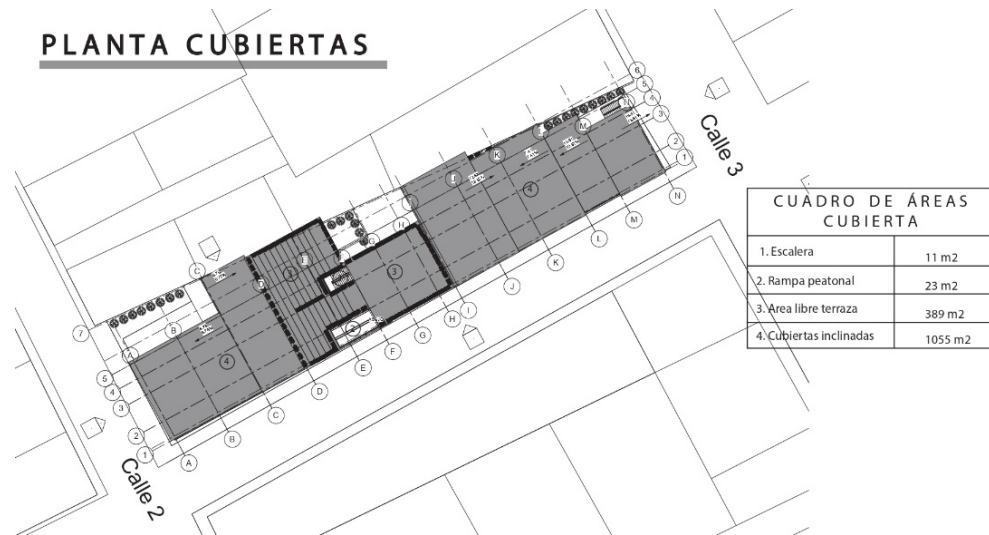
Ilustración 27 Planta general cubiertas con su respectivo cuadro de áreas
