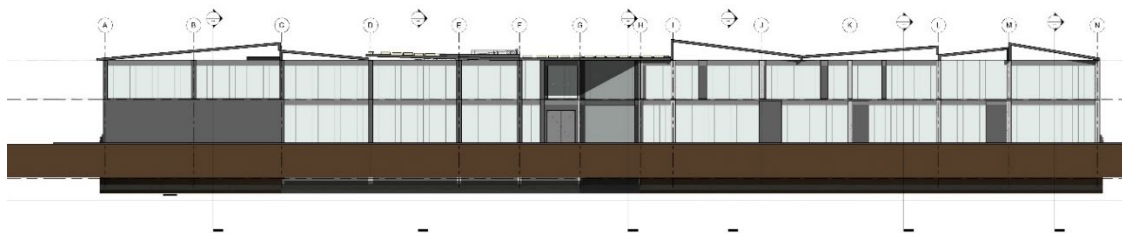
Ilustración 28 Alzado fachada norte Esc. gráfica
