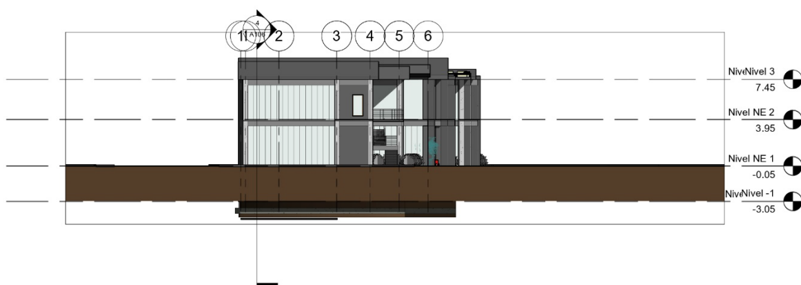
Ilustración 31 Alzado fachada occidente Esc. gráfica
