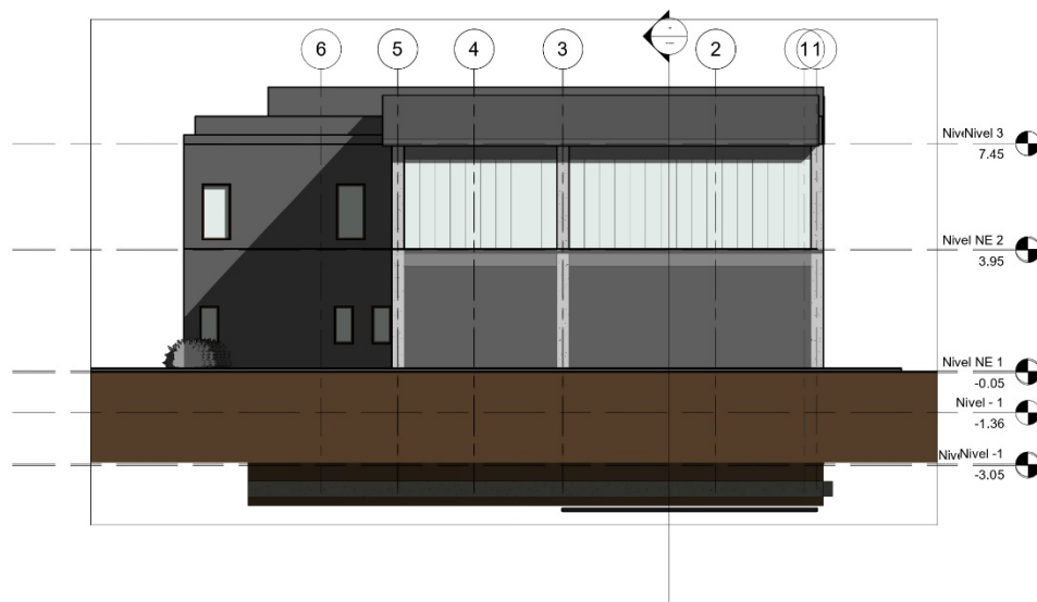
Ilustración 30 Alzado fachada oriente Esc. gráfica
