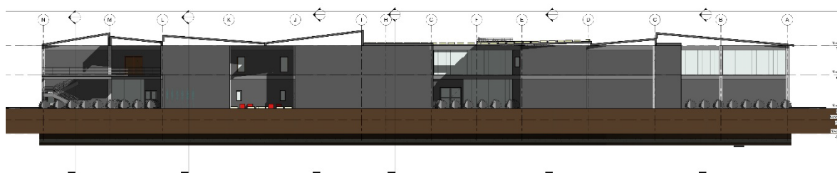
Ilustración 29 Alzado fachada sur Esc. gráfica
