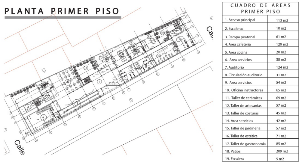
Ilustración 25 Planta general primer piso con su respectivo cuadro de áreas
