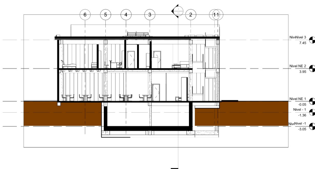
Ilustración 34 Corte transversal cafetería, rampa y ludoteca Esc. gráfica
