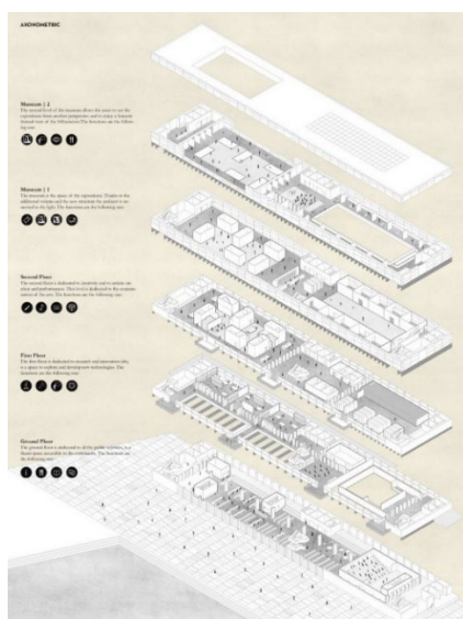
Ilustración 14 Explotado general proyecto Kajskjul 113, Suecia.
