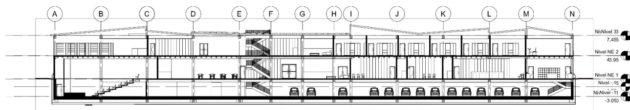
Ilustración 32 Corte longitudinal Esc. gráfica
