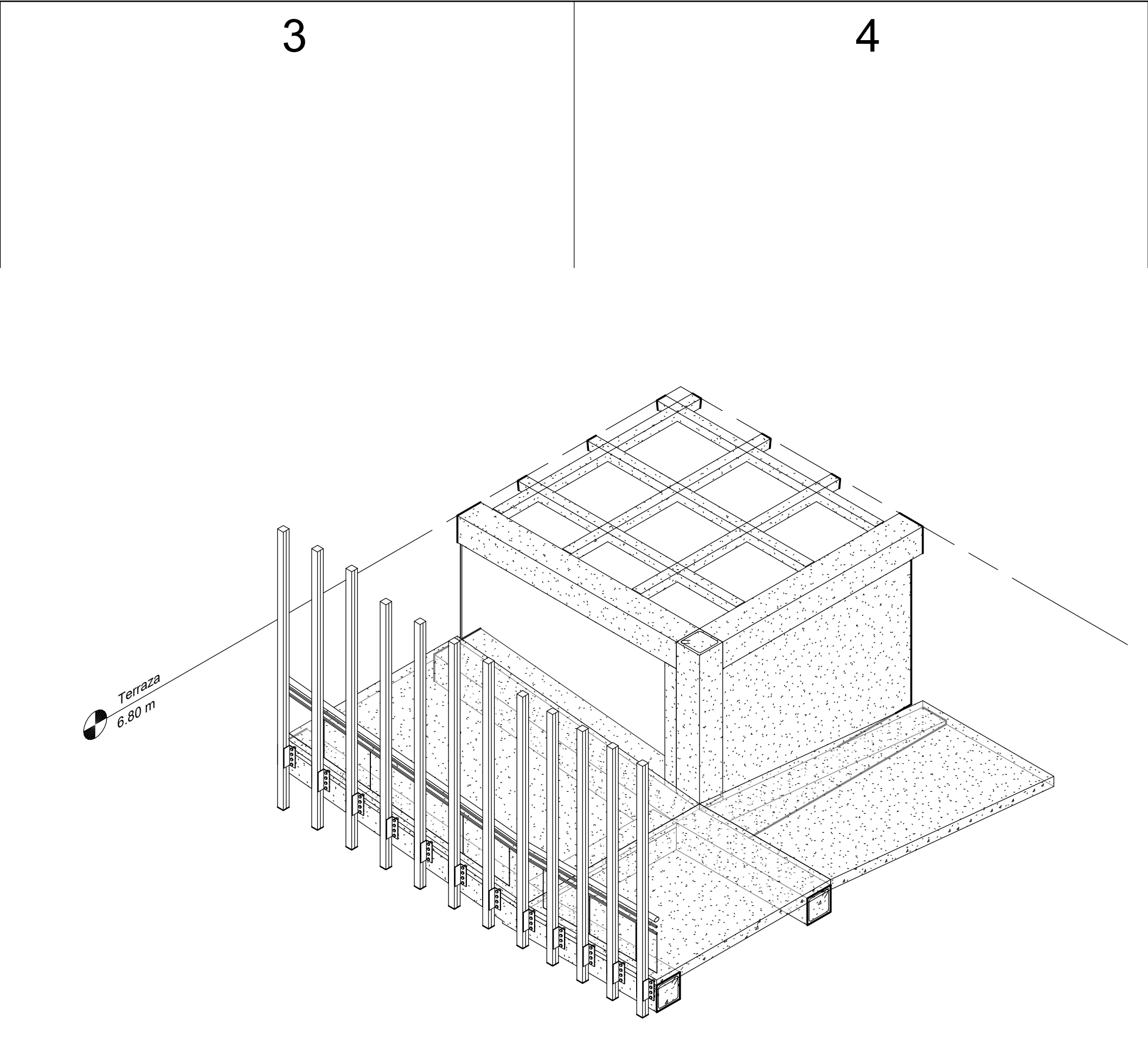
3 Detalle rampa
