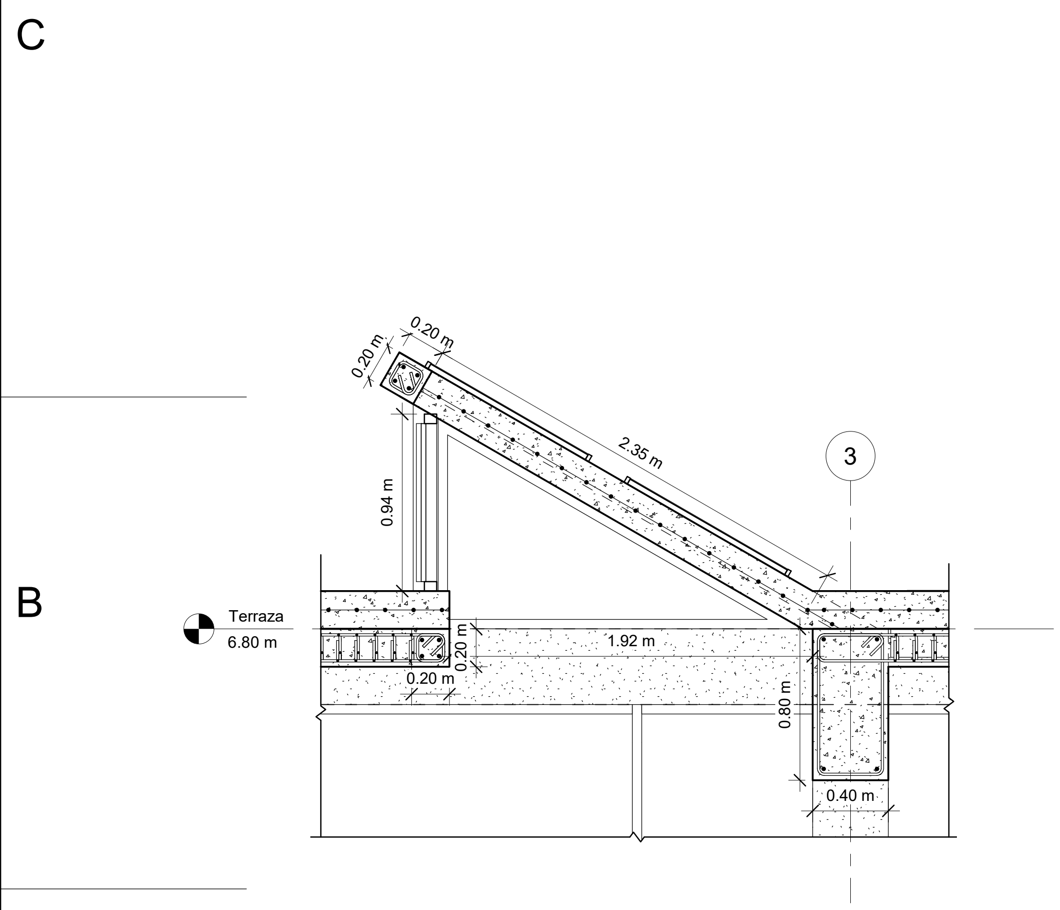
2 Corte cubierta auditorio 1 : 20
