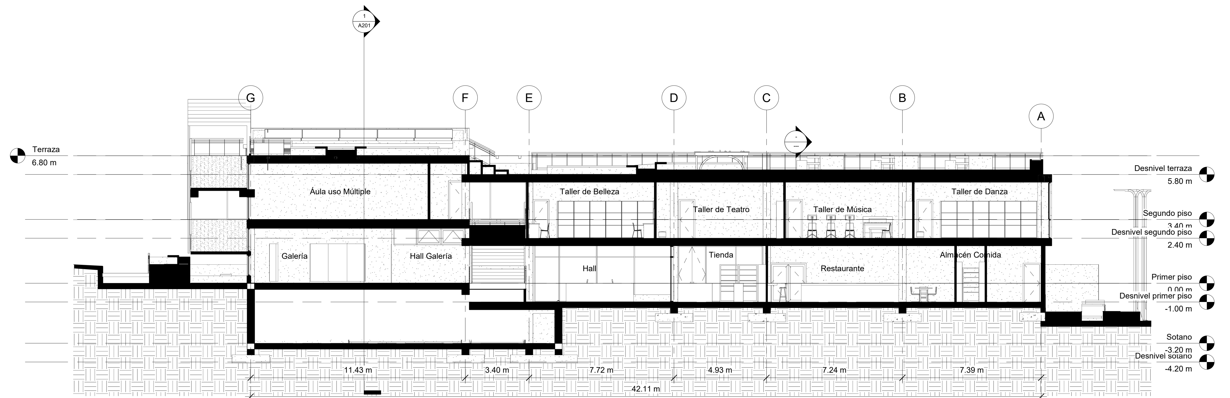
2 Corte Longitudinal 1 : 100
