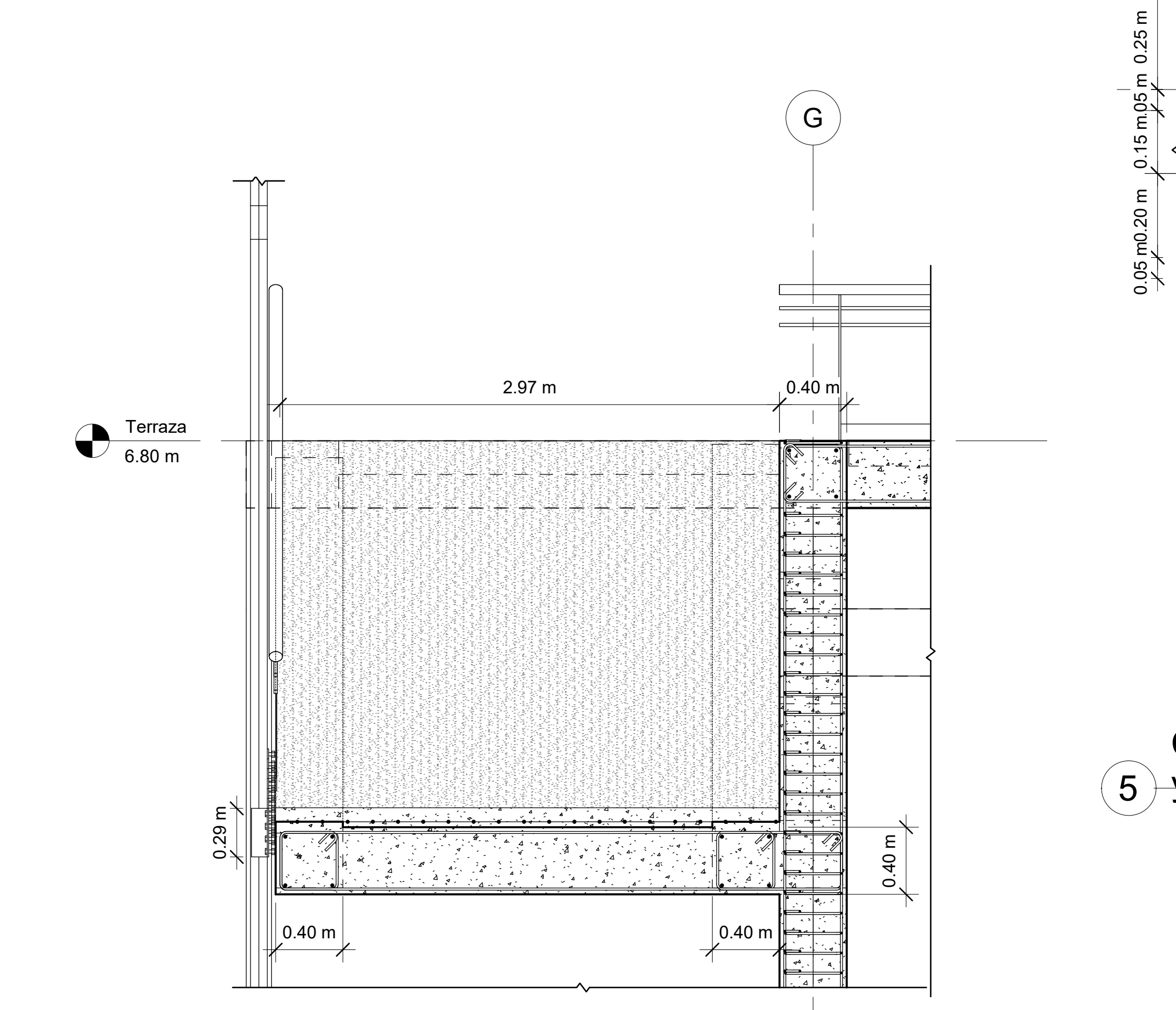
4 Corte detalle rampa
