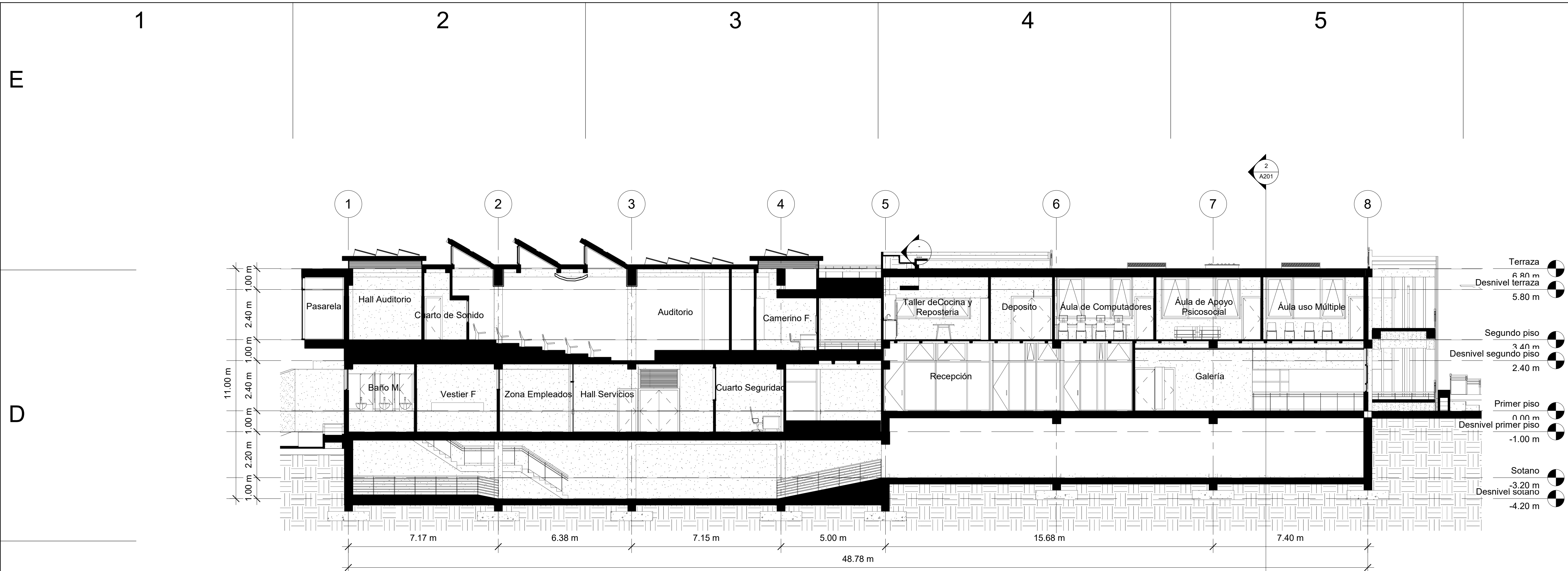
1 Corte Transversal 1 : 100
