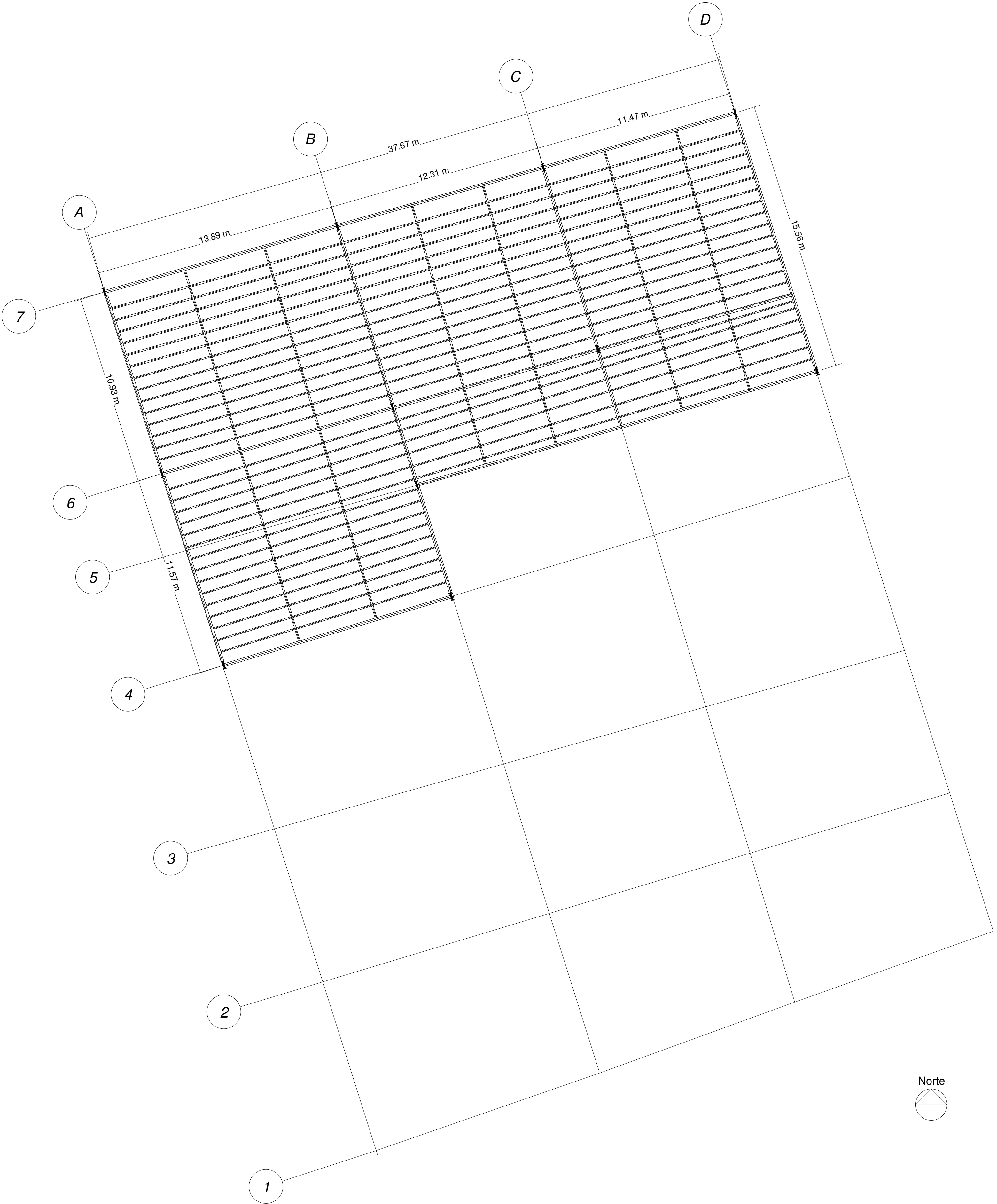
2 PLACA DE CUBIERTA NIVEL E103
