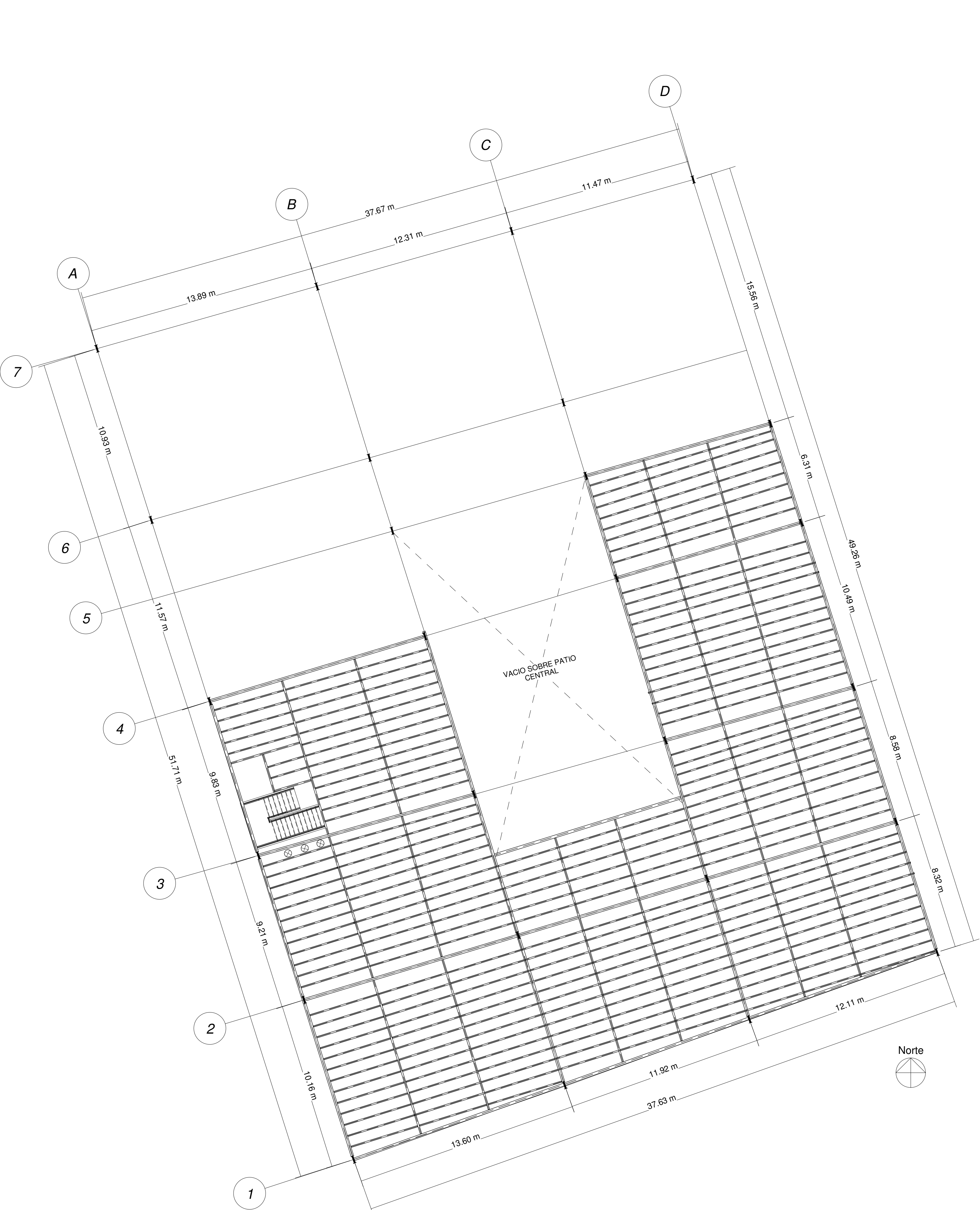
1 PLANTA DE ENTREPISO E103
