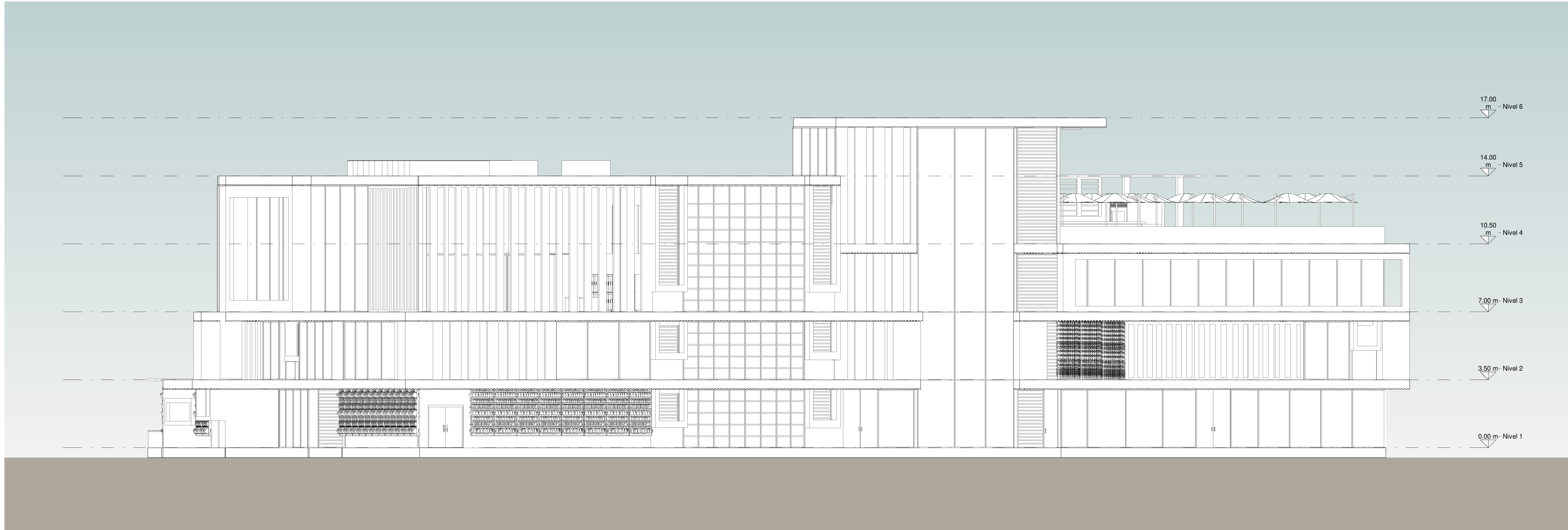
1 Fachada Oeste A108 1:100
