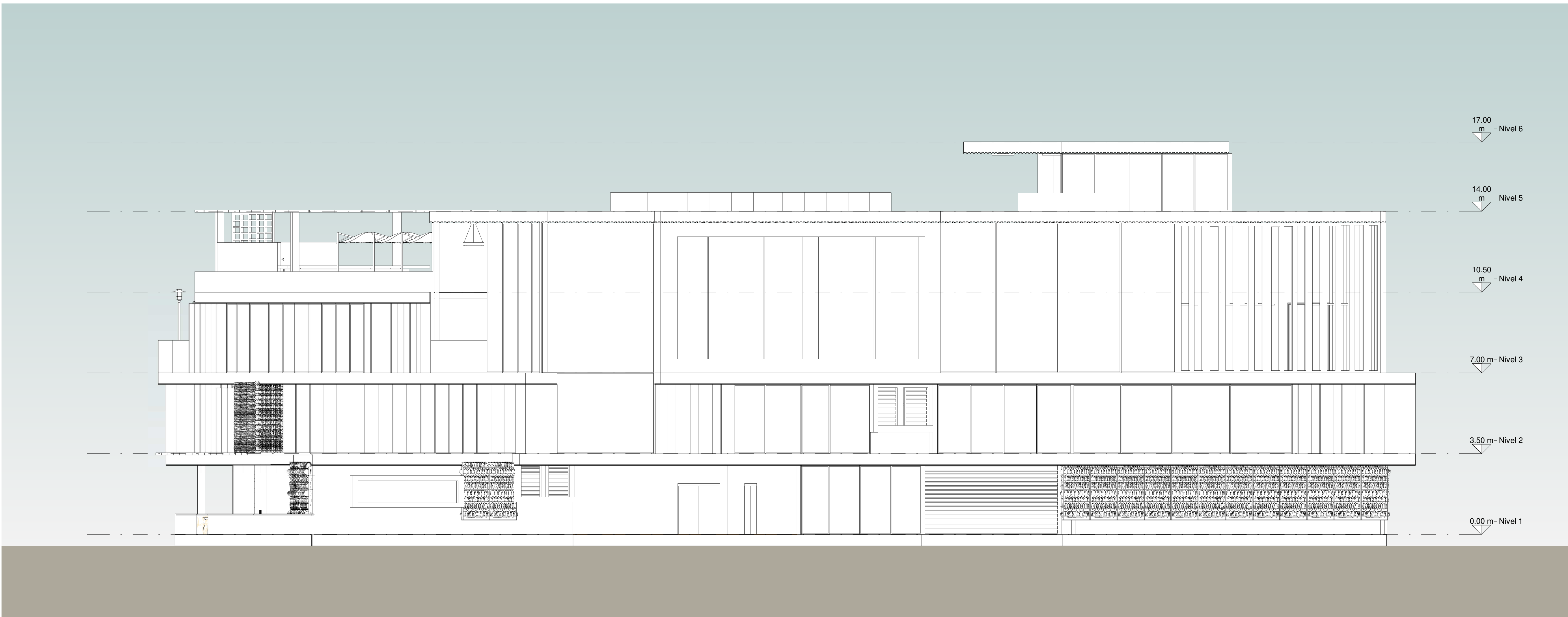
2 Fachada Norte A107 T: 100
