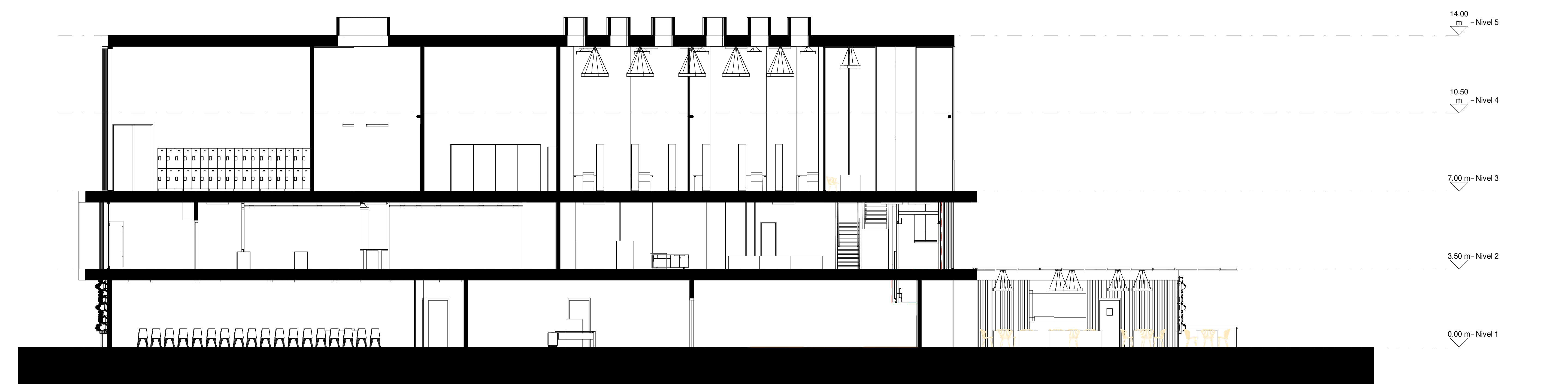
1 CORTE CC. A106 | 1:100
