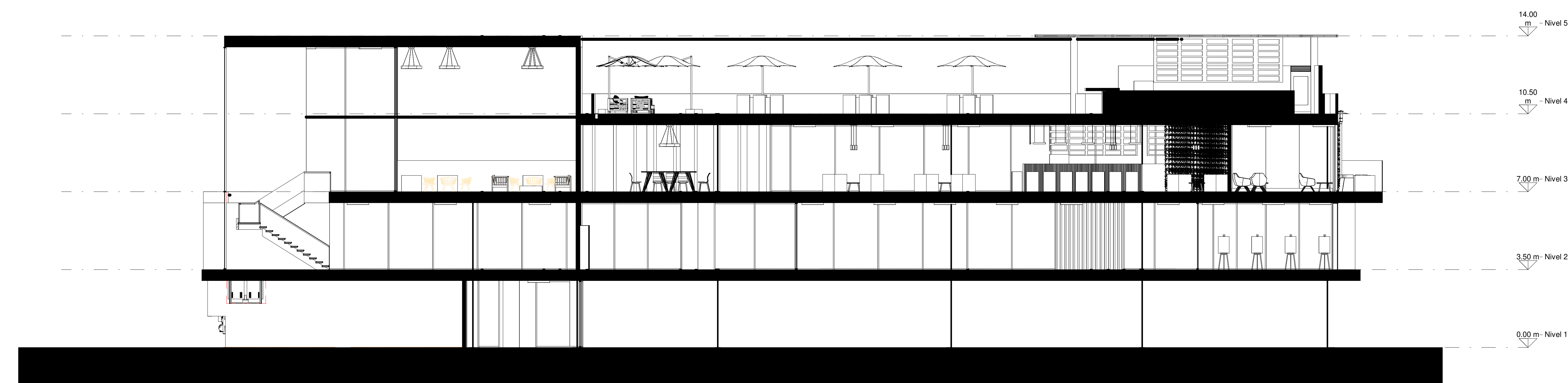
2 CORTE DD. A106 | 1:100
