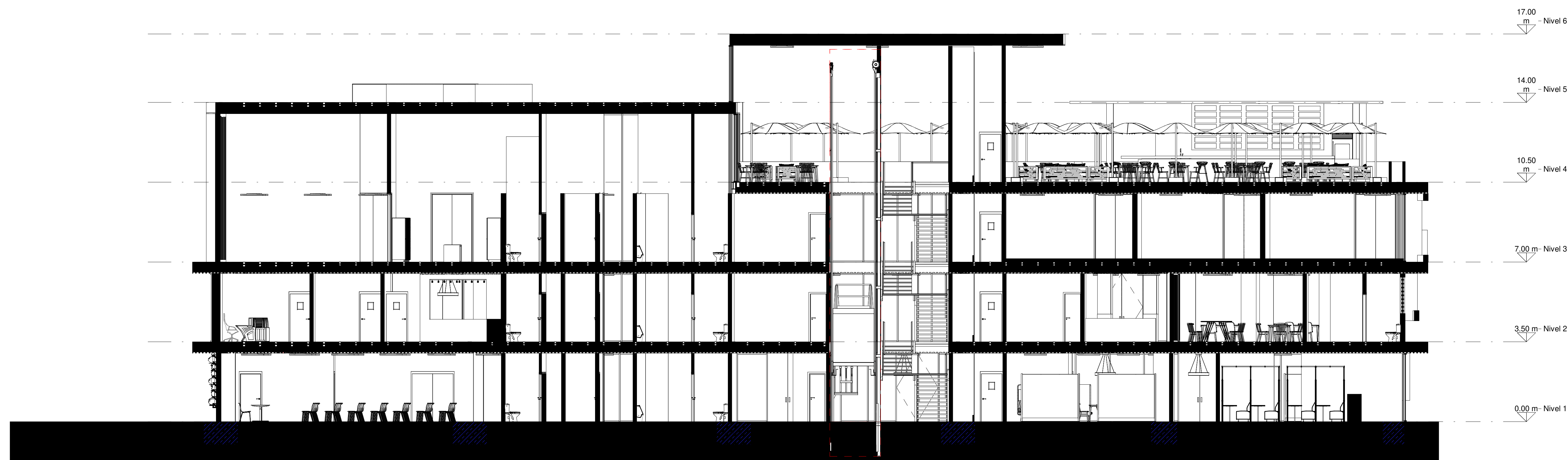
1 | CORTE AA A105 1:100
