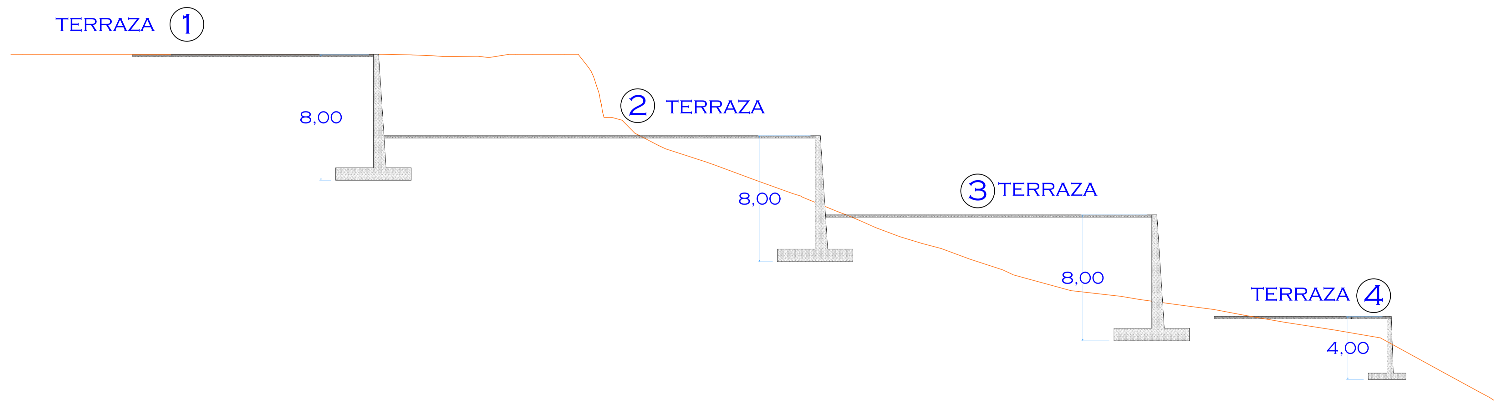
4 PT-4 PERFIL TERRENO 4 1:150
