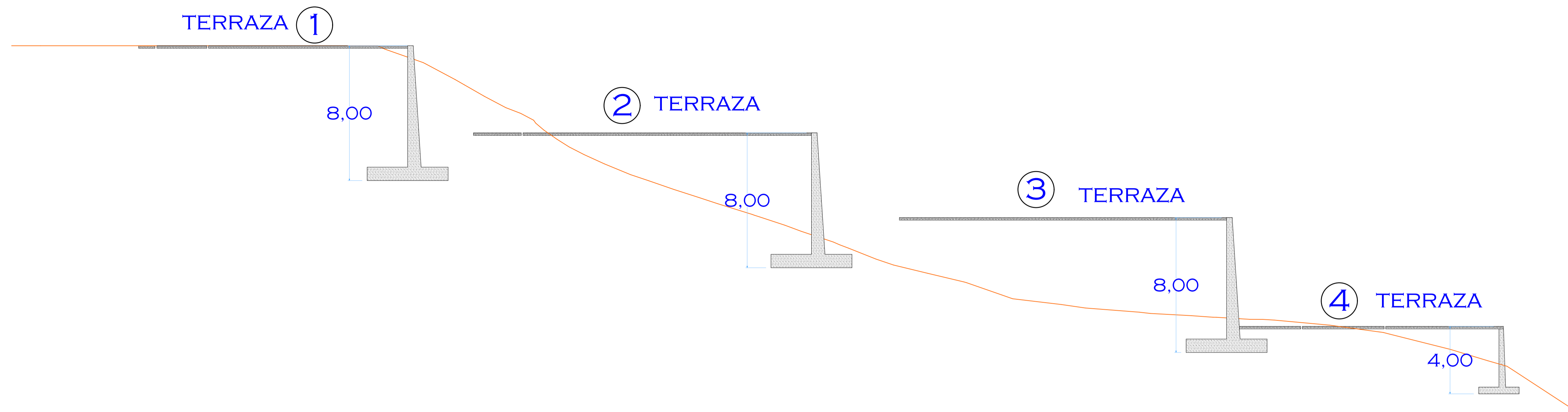
3 PT-3 PERFIL DEL TERRENO 3 1:150
